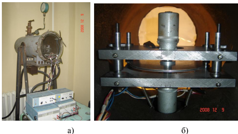
Рис. 1. Общий вид экспериментального оборудования и устройства в вакуумной камере
