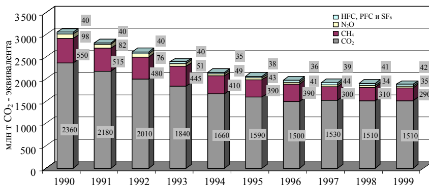
Рис. 3.1. Динамика выбросов парниковых газов в России в 1990–1999 гг. (без учета нетто-стока CO 2 в лесах) /138/
