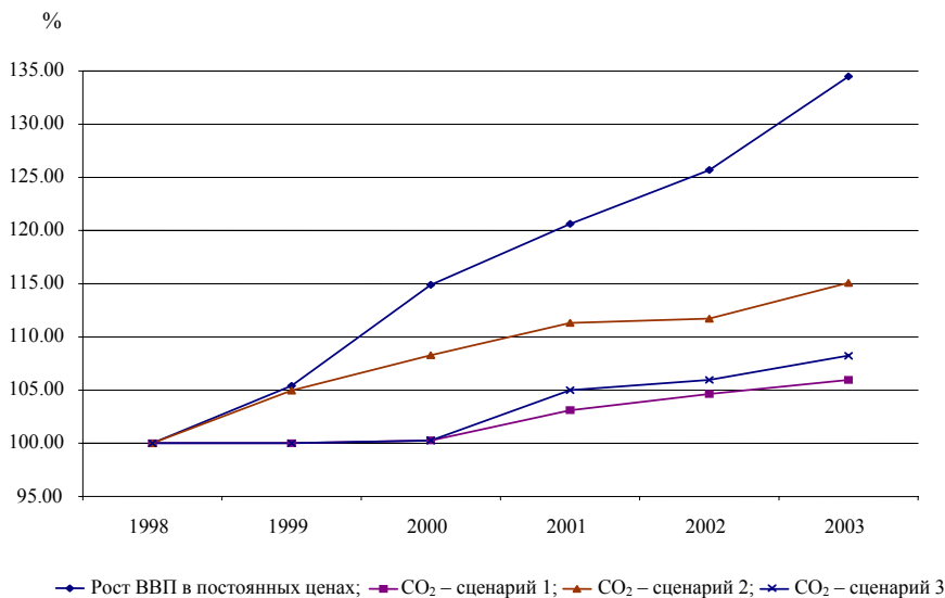
Рис. 3.2. ВВП и динамика выбросов CO 2 в России
