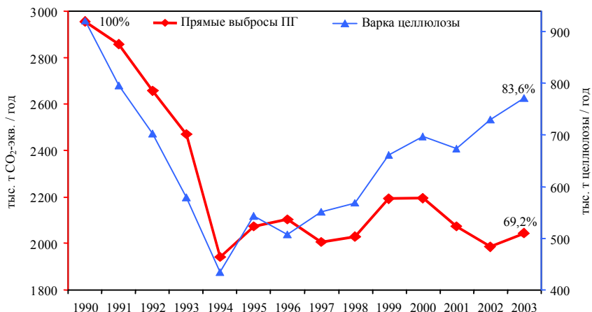
Рис. 3.3. Варка целлюлозы и выбросы парниковых газов на ОАО «Архангельский ЦБК» в 1990–2003 гг. (в % к уровню 1990 г.)/153/
