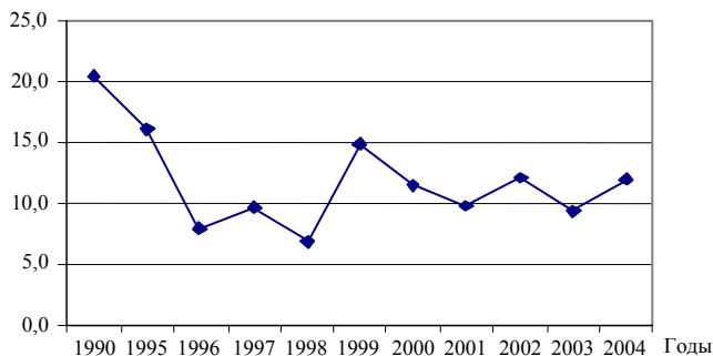
Рис. 4.3. Эмиссии НМУ в промышленности, Гг
