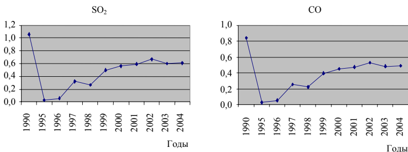
Рис. 4.4. Эмиссия SO 2 и CO в промышленности, Гг
