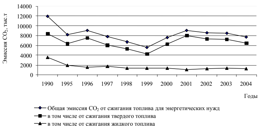
Рис. 4.1. Динамика эмиссии \text{CO}_2 от сжигания топлива в энергетических целях
