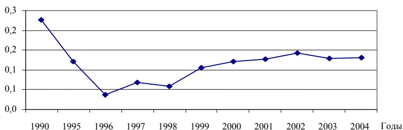
Рис. 4.2. Эмиссия NO x в промышленности, Гг
