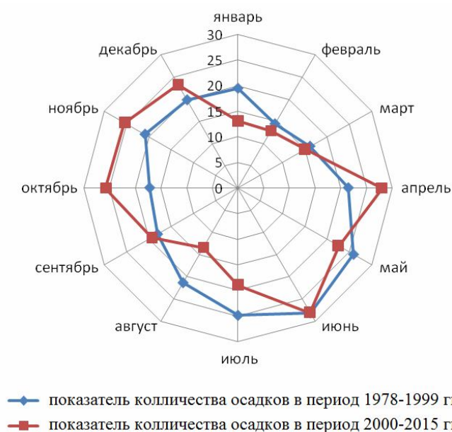
Рис. 3. Распределение количества осадков (мм) в Астраханской области по месяцам за периоды 1978–1999 гг. и 2000–2015 гг.
