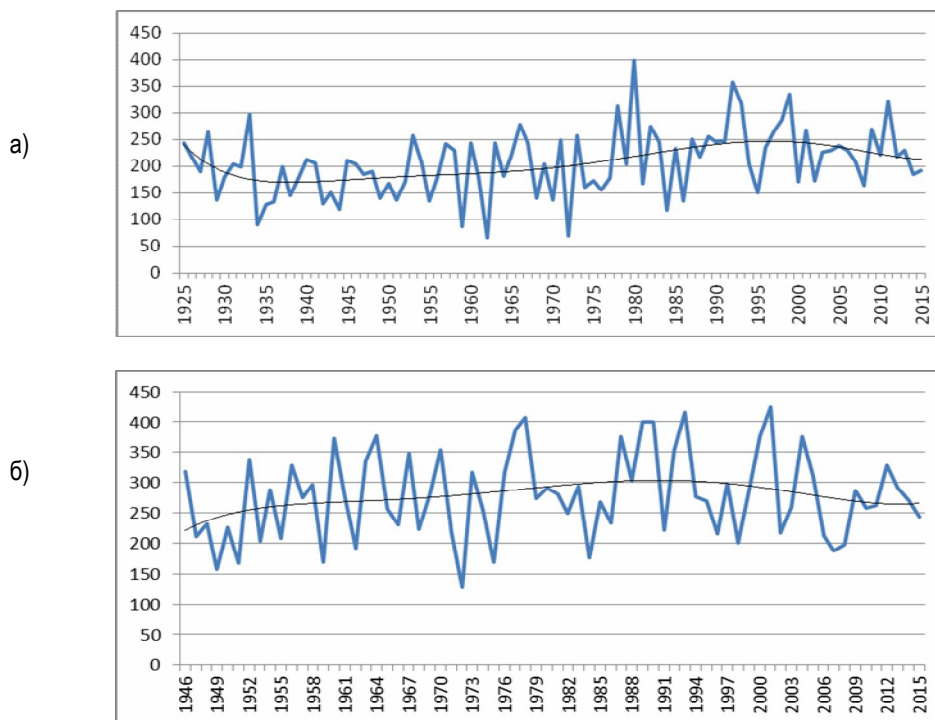
Рис. 2. Средний многолетний ход годового количества атмосферных осадков в аридной зоне
