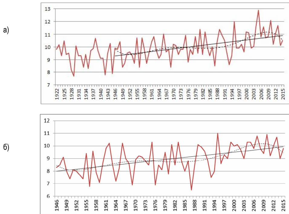
Рис. 1. Временной ход среднегодовой температуры воздуха: а) по метеостанции Астрахань; б) по метеостанции Черный Яр
