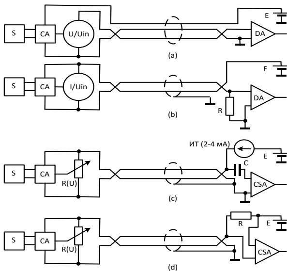
Рисунок 1 – Основные типы аналоговых интерфейсных решений
