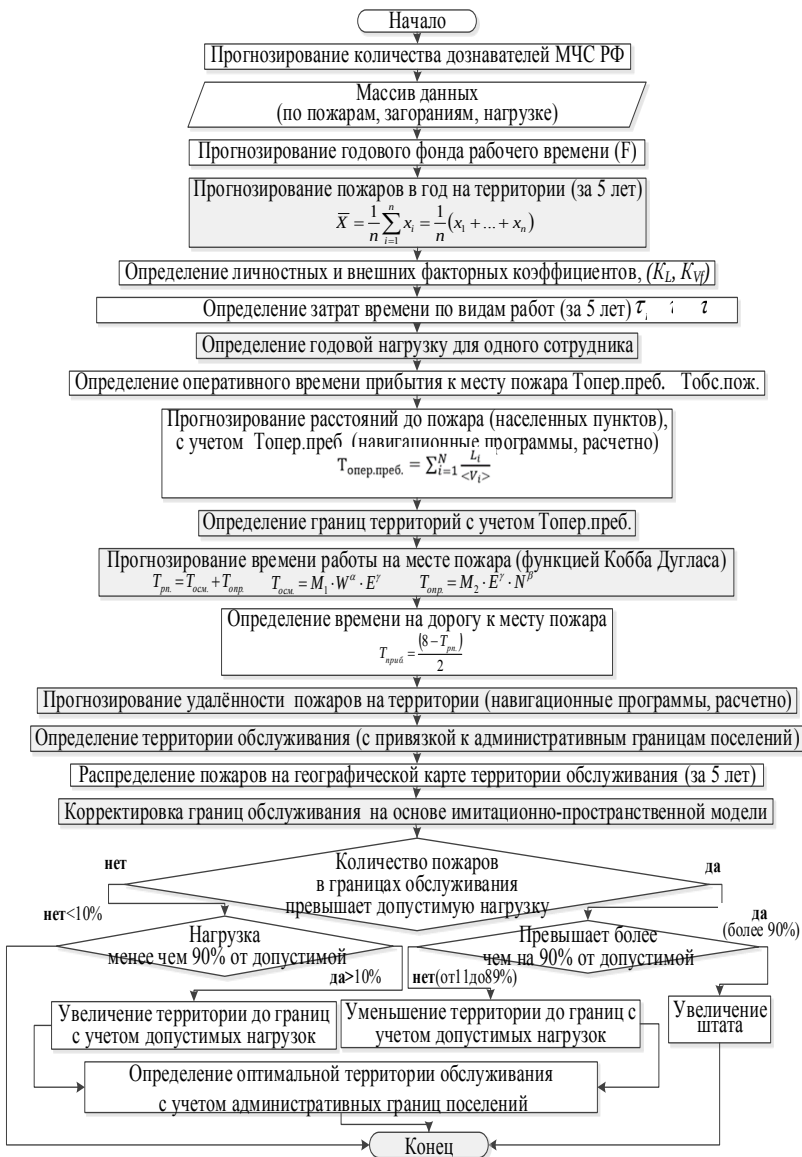
Рисунок 1 – Блок-схема общего алгоритма прогнозирования оптимальной численности дознавателей территориальных подразделений ФГПН
