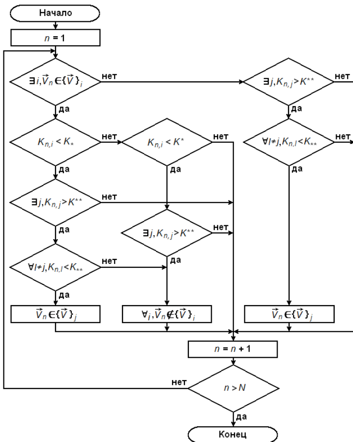
Рисунок 1 – Упрощенная блок-схема алгоритма переклассификации
