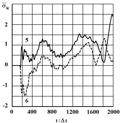
Рисунок 5 – Изменение упругого контурного напряжения \bar{\sigma}_k в точках 5 и 6 на контуре десятиэтажного здания во времени t/\Delta t
