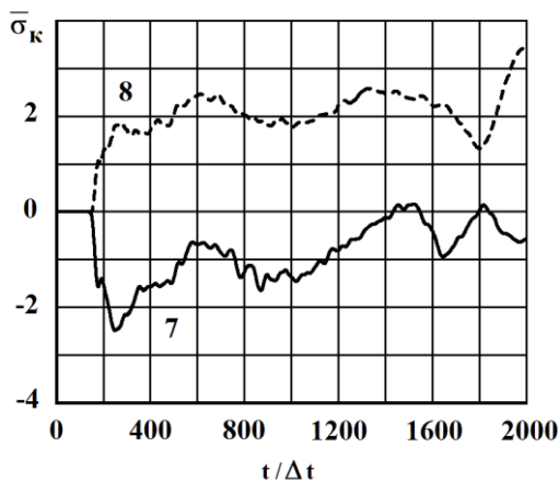
Рисунок 6 – Изменение упругого контурного напряжения \bar{\sigma}_к в точках 7 и 8 на контуре десятиэтажного здания во времени t/\Delta t
