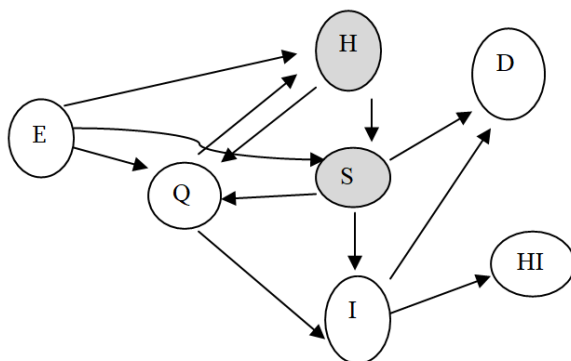
Рисунок 1 – Ориентированный граф борьбы с эпидемией
