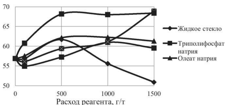
Рисунок 2. Влияние расхода ПАВ на прирост класса крупности -0,074 мм в измельченной магнетитовой руде
