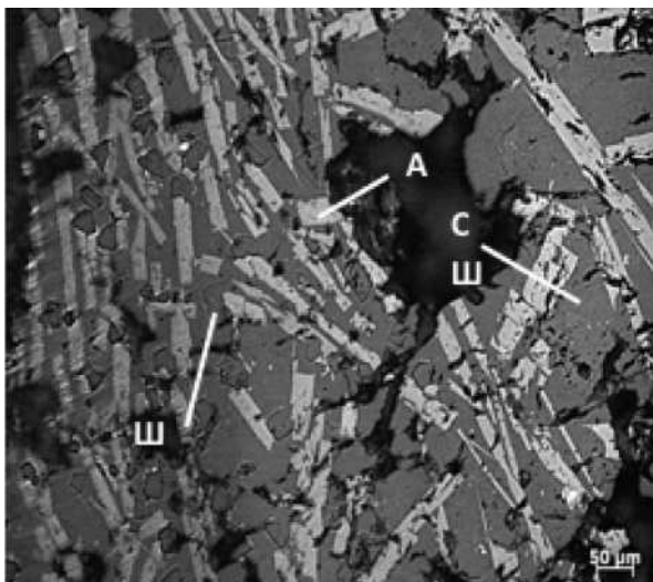
Рисунок. Микрофотография шлака, полученного при 1475°C:
