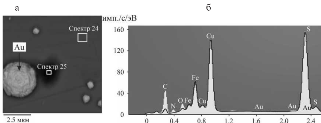
Рисунок 1. ASEM-снимок аншлифа халькопирита с Au и ЦЭДЭТК (а). Сравнение энергодисперсионных спектров аншлифа халькопирита с нанесенным золотом и реагента ЦЭДЭТК на поверхности минерала (б).
