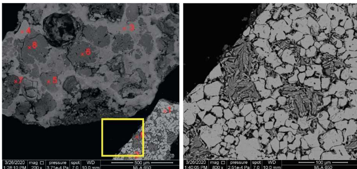
Рисунок 4. Агрегаты обломков кремнисто-глинисто-железистого состава, сцементированных гидрогетитом, и агрегатов гематита и акерманита ( \text{Ca}_2\text{MgSi}_2\text{O}_7 ). Крупность -2,5+1,6 мм.
