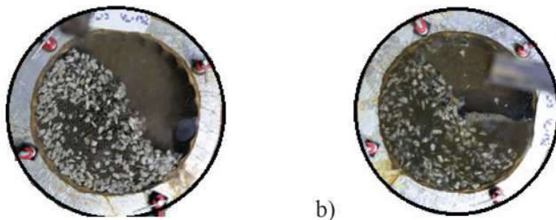
Рисунок. Распределение загрузки в сечении барабана мельницы ММПСИ при размерах частиц минералов больше диаметра шаров: а) при сухом и б) при мокром измельчении
