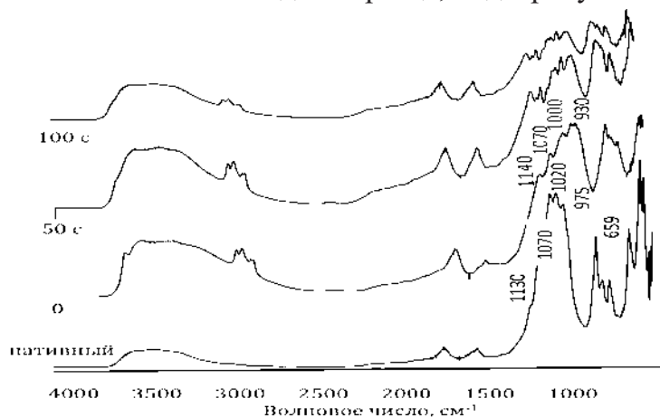
Рисунок 2. ИК-спектры эвдиалита в нативном состоянии и после контакта с соляной кислотой в исходном ( P_{бр}=0 с) и модифицированном ДБР состоянии ( t_{обр} = 50 и 100 с)
