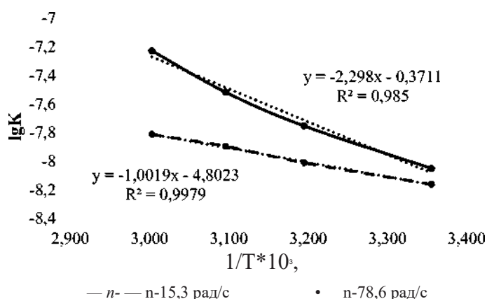
Рисунок 2. Зависимость константы скорости растворения ( \text{LgK} ) золота в тио-цианатных растворах от температуры при частоте вращения диска 15,7 и 78,6 рад/с
