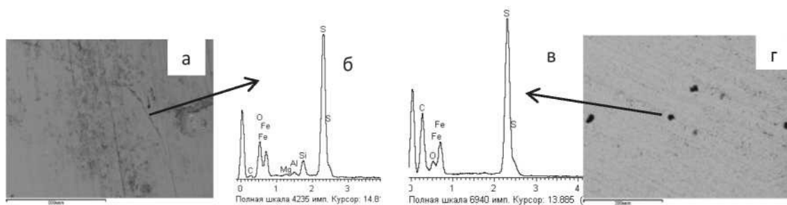
Рисунок 1. Микрофотографии поверхности аншлифа пирита и энергодисперсионные спектры участка аншлифа пирита Кургашинканского месторождения (а, б), Березовского месторождения (в, г), после контакта с 0,1% раствором ДТМ
