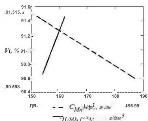
Рисунок 4. Области изменения концентраций марганца в нейтральном растворе и серной кислоты в отработанном электролите, при которых выход цинка по току экстремальный
