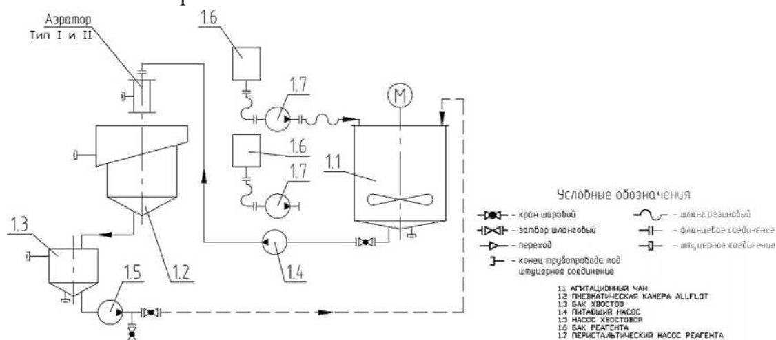
Рисунок 2. Схема цепи аппаратов «allflot» - подключение в условиях действующей технологической схемы
