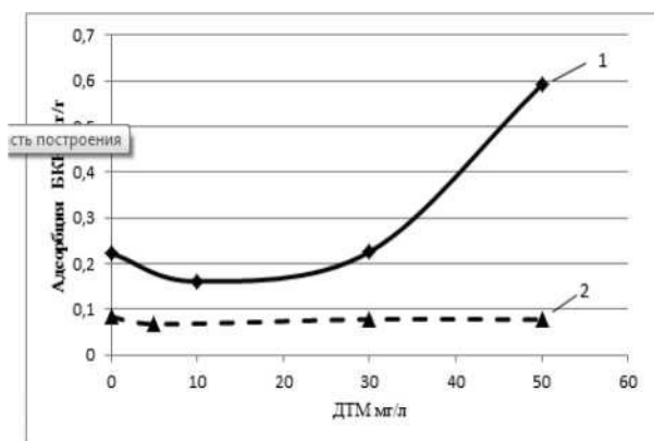
Рисунок 3. Влияние концентрации дитиопирилметана в пульпе на адсорбцию бутилового ксантогената на мономинеральных фракциях пирита Кургашиинканского (1), пирита Березовского (2) месторождений
