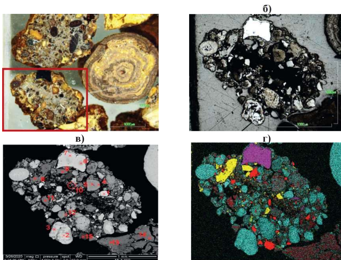
Рисунок 3. Агрегат оолитов и обломков гидрогетита, оксидов марганца, кальцита,
