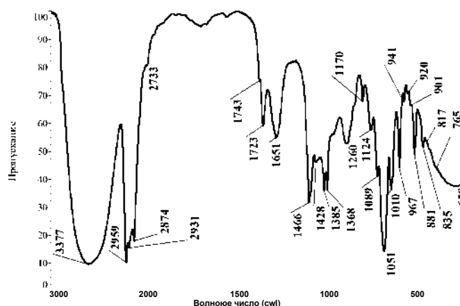
Рисунок. ИК-спектральный анализ пенообразователя СВИМ
