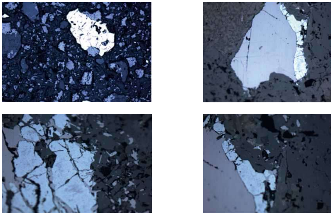
Рисунок 1. Микроструктура образцов:
