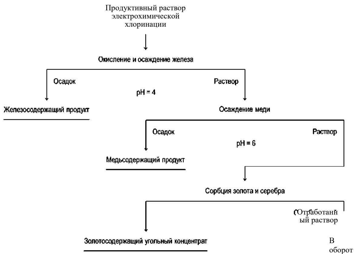
Рисунок 3. Схема переработки продуктивного раствора электрохимической хлоринации
