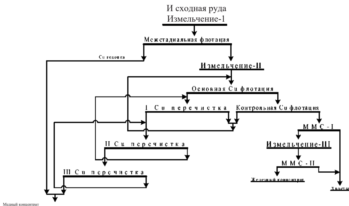
Рисунок. Технологическая схема обогащения руды Волковского месторождения на АО «Святогор»
