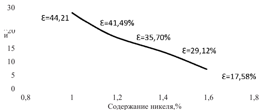
Рисунок 2. Зависимость качества концентрата дофлотации и извлечения никеля в него от выхода (содержание никеля в исходном МНПП 0,64%)
