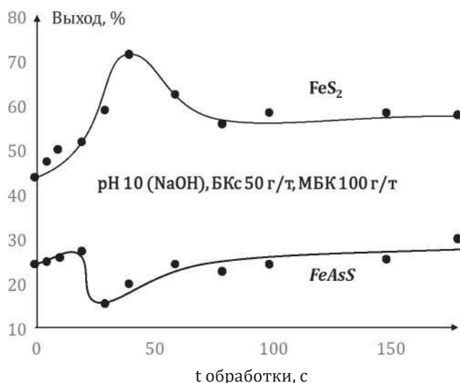
Рисунок 1. Зависимость флотационной активности пирита и арсенопирита от продолжительности обработки ДБР
