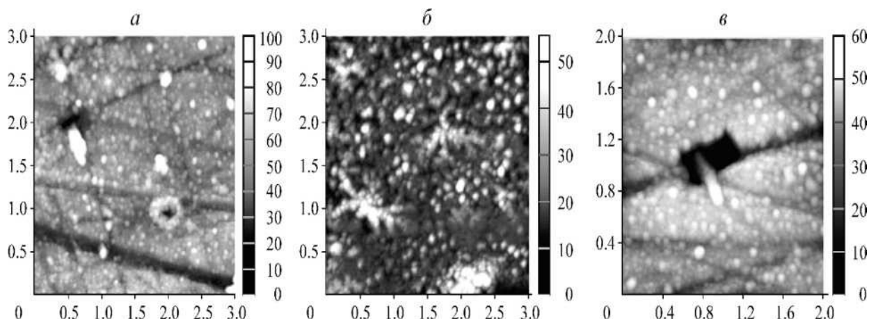
Рисунок 1. АСМ-изображения фрагментов поверхности эвдиалита после воздействия ДБР ( P_{бр} = 50 с). Размер области сканирования: 3 x 3 (а, б); 2*2 (в) мкм
