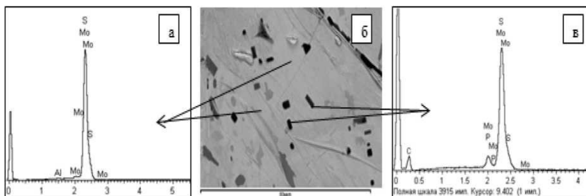
Рисунок 1. ASEM-изображение поверхности молибденита после обработки реагентом КР (б) и энергодисперсионные спектры участков (а, в)
