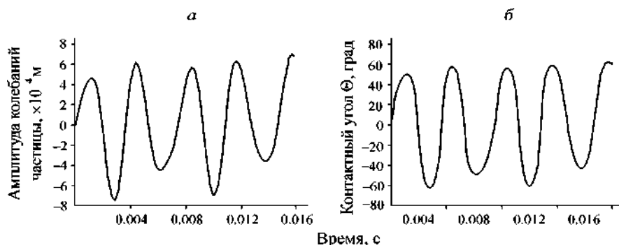
Рисунок. Амплитуда колебаний частицы на поверхности пузырька (а); угол отклонения \Theta границы раздела «газ- жидкость» от горизонта по линии контакта с минеральной поверхностью в зависимости от времени (б); скорость диссипации энергии e = 15 \text{ м}^2/\text{с}^3
