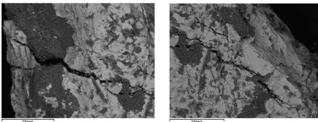
Рисунок 2. Микротрещиноватость исходной руды
