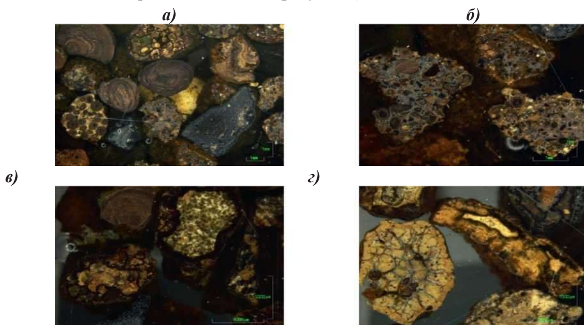
Рисунок 1. Материал классов крупности -5+2,5 мм (а, б) и -2,5+1,6 мм (в, г), представленный оолитами и агрегатами, состоящими из оолитов и обломков кварца и полевых шпатов, сцементированных глинисто-гидрогётитовым цементом
