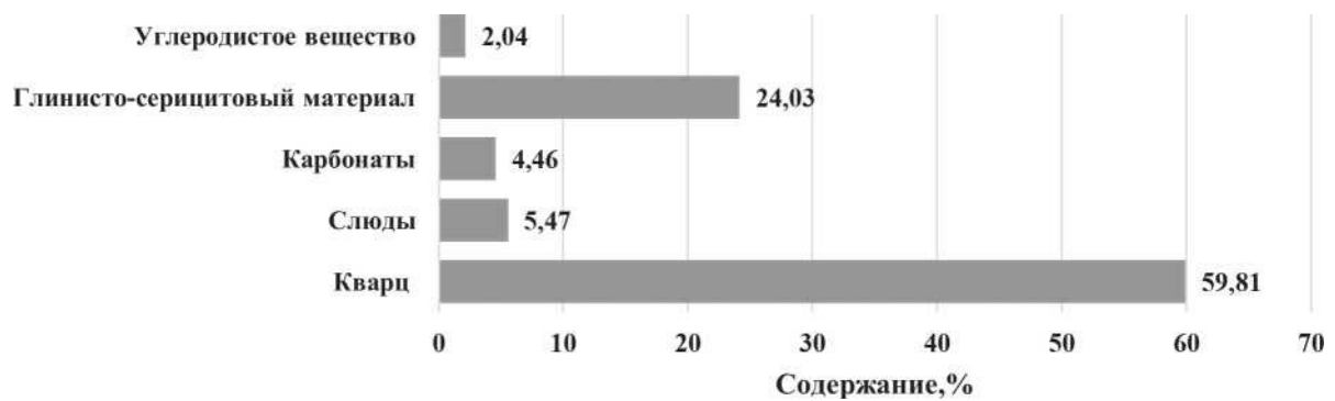
Рисунок 1. Минералогический состав исследуемых образцов руд
