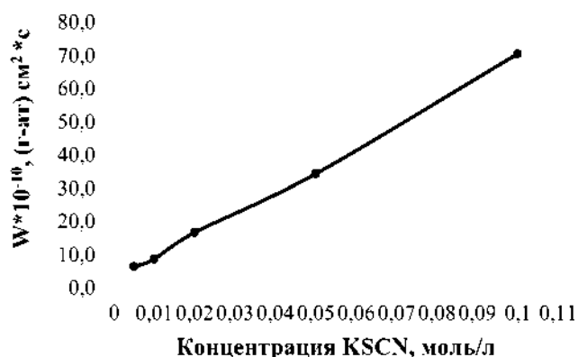
Рисунок 3. Зависимость скорости растворения золота от концентрации тиоцианата калия при температуре 298 K
