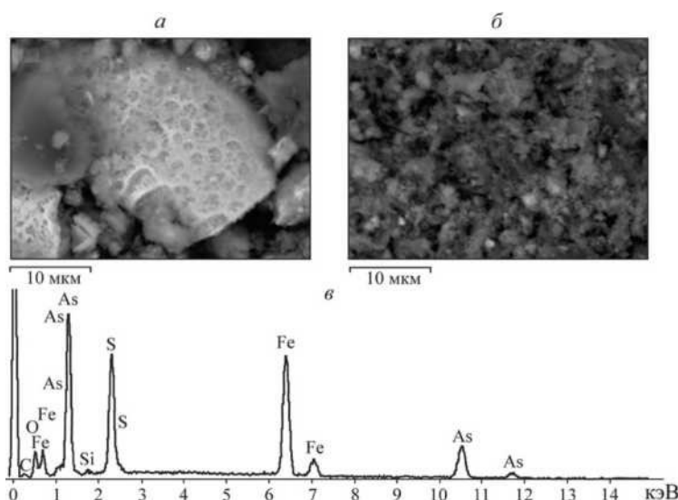
Рисунок 1. Изображение (а, б) и энергодисперсионный спектр (в) поверхности частиц арсенопирита после выщелачивания ультразвуком 1.25 Вт-ч/г
