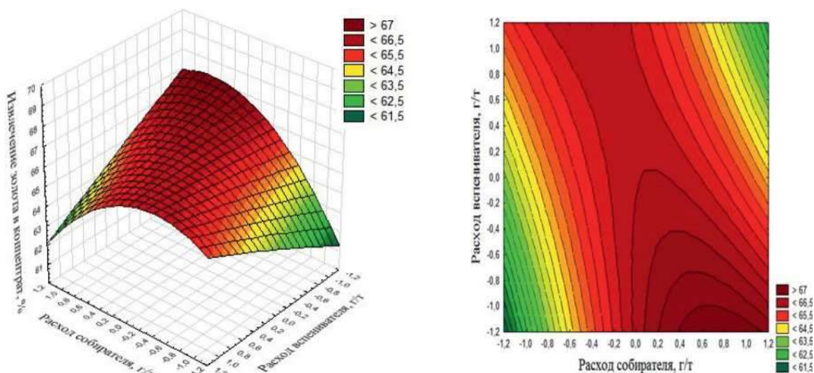
Рисунок 3. Поверхность отклика (слева) и карты линий уровня (справа) для извлечения золота в концентрат отхода собирателя и вспенивателя
