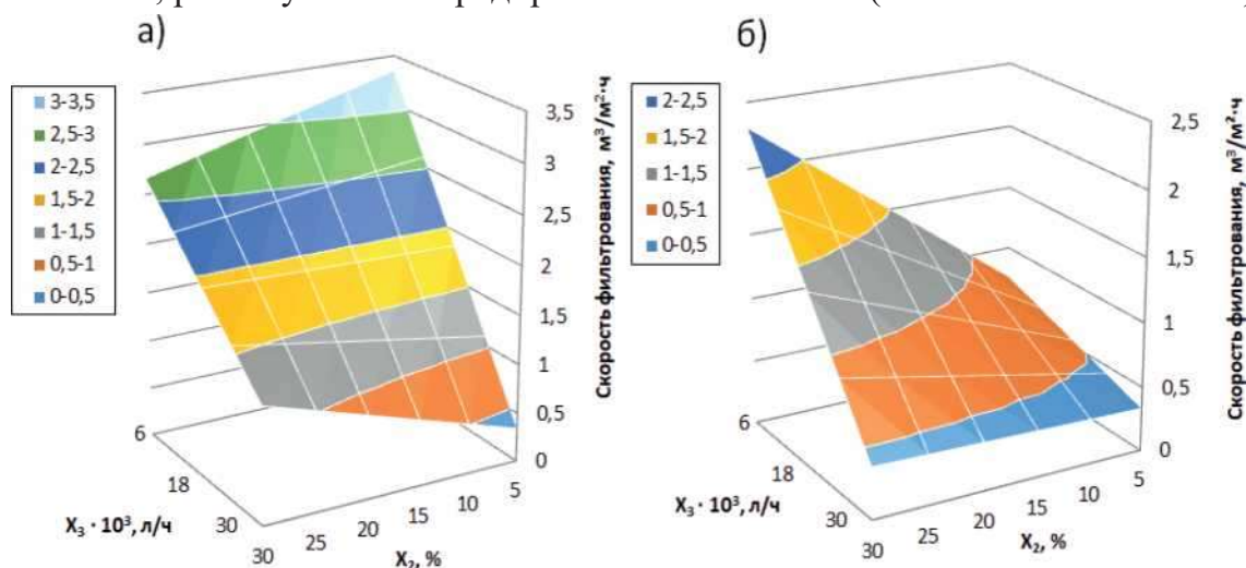
Рисунок. Поверхность изменения скорости фильтрования пульпы карбоната лантана
