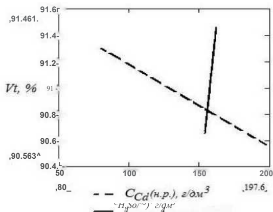
Рисунок 3. Области изменения концентраций кадмия в нейтральном растворе и серной кислоты в отработанном электролите, при которых выход цинка по току экстремальный
