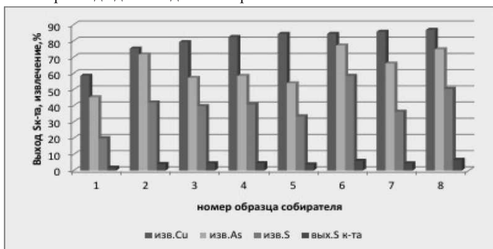
Рисунок. Диаграмма извлечения меди, мышьяка, серы и выхода коллективного концентрата, на исследуемых образцах сульфидных собирателей, г/т:
