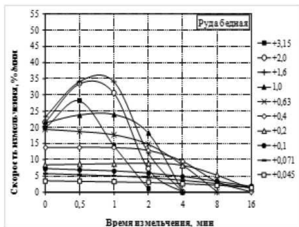
Рисунок 1. Изменение скоростей измельчения расчетных классов от времени при измельчении в стержневой мельнице бедной лопаритовой руды и руды текущей добычи
