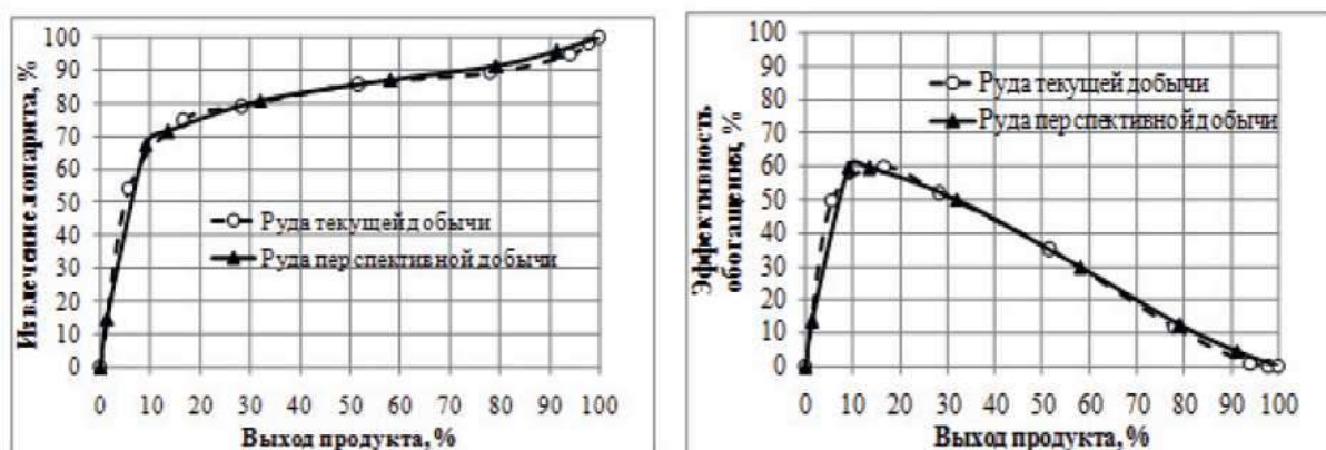
Рисунок 2. Винтовая сепарация лопаритовой руды перспективной и текущей добычи
