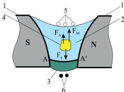
Рисунок 1. Схема способа магнитожидкостной сепарации с двумя несмешивающимися ферромагнитными жидкостями разной плотности: 1 - полюсные наконечники электромагнитной системы; 2, 3 - соответственно слой легкой и плотной ферромагнитной жидкости; 4 - твердое тело
