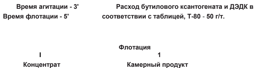
Рисунок 1. Схема флотационного эксперимента с свинцово-цинковой рудой Горевского месторождения
