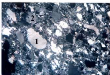
Рисунок 2. Призматические кристаллы кварца с закругленными краями (1), эрозированный полевой шпат (2), агрегаты серицита (3) 25-кратное увеличение, Nikon ECLIPSE LV100-POL
