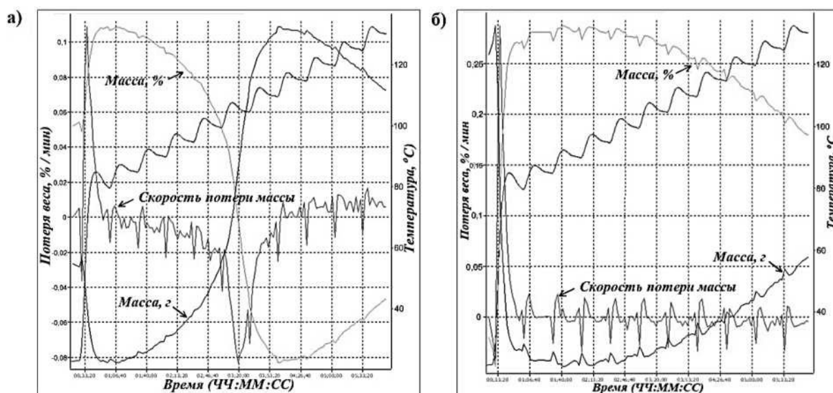
Рисунок 1 - ТГ-зависимости для исследуемых образцов а) древесного угля, пропитанного льняным маслом, б) сухого древесного угля
