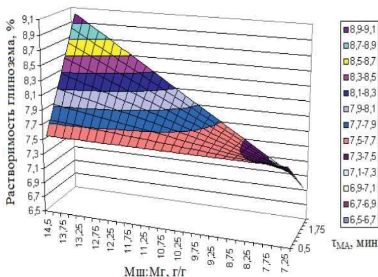
Рисунок. Поверхность изменения растворимости глинозема в криолитовом расплаве ( KO=2,3 ) при температуре 1000^{\circ}C от режимов предварительной МА при скорости вращения барабанов мельницы 100 об/мин
