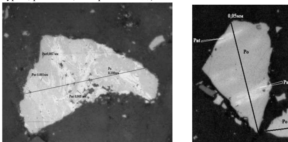
Рисунок 1. Пламневидные выделения пентландита в пирротине
