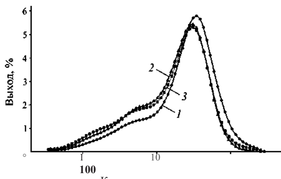
Рисунок 2. Распределение по крупности частиц концентрата:
