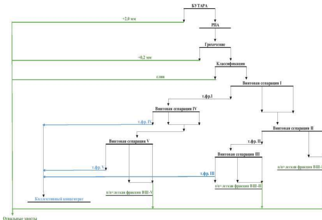
Рисунок 1. Схема получения коллективного концентрата по гравитационной схеме
