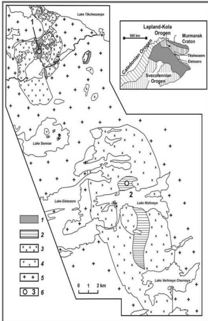
Рис. Обобщенная геологическая схема ультрабазит-базитового щелочно-карбонатитового Тихеозерско-Елетъзерского комплекса:
