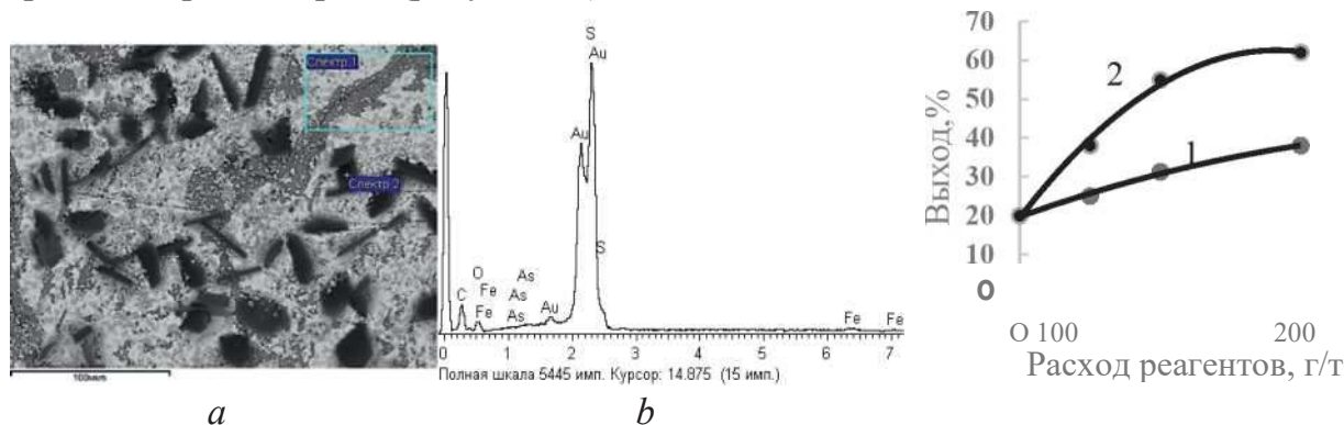
Рисунок 1. ASEM-изображение (a) и энергодисперсионные (X-ray) (b) спектры участков поверхности анишлифа арсенопирита с низкоразмерным Au после воздействия реагента МДТК (LEO 1420VP); флотация природного арсенопирита (1) и с Au (2) комбинацией реагентов МДТК и БутКс (1:1) - (c)
