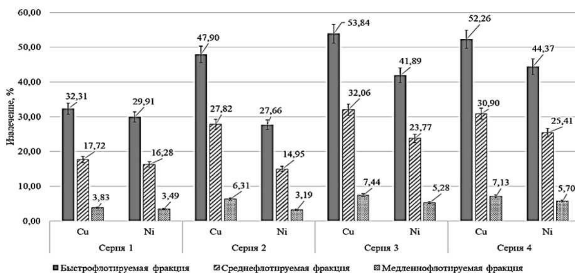
Рисунок. Результаты оценки флотуемости
