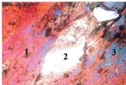
Рисунок 1. Серицитовые чешуйки микроразмера (1), объединенные в параллельные полосы, перемежающиеся с кварцем (2) и полевым шпатом (3) 25-кратное увеличение, Nikon ECLIPSE LV100-POL
