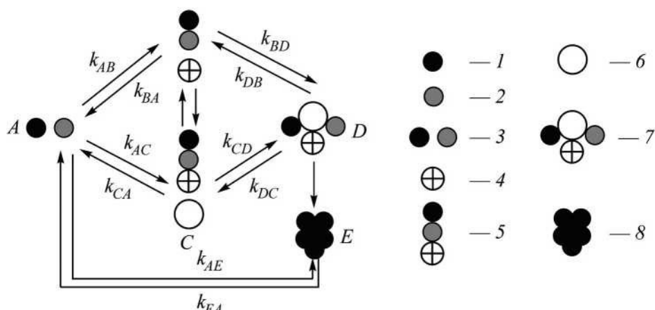
Рисунок 1. Схемамногостадийной модели напорной флотации:
