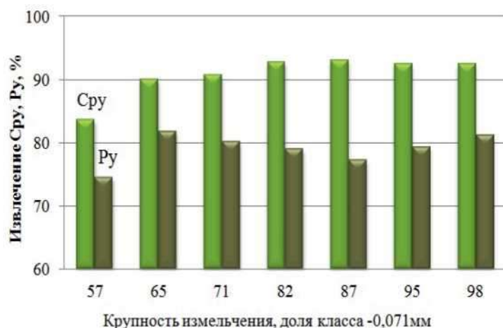
Рисунок 1. Извлечение халькопирита (Cu) и пирита (Py) в коллективные концентраты в зависимости от крупности измельчения
