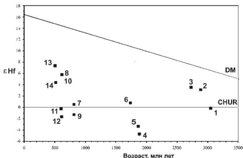
Рис. 2. Диаграмма в координатах «U-Pb изотопный возраст – \epsilon_{\text{Hf}} (T)» для цирконов из гарцбургитов и дунитов Шаманского массива.
