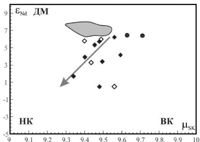
Рис. 2. Диаграмма в координатах \mu_{\text{SK}}\text{--}\epsilon_{\text{Nd}} для поздневендских и раннепалеозойских гранитоидов Каахемского батолита Восточной Тувы и сопредельных территорий ЦАСП. Условные обозначения см. рис. 1.
