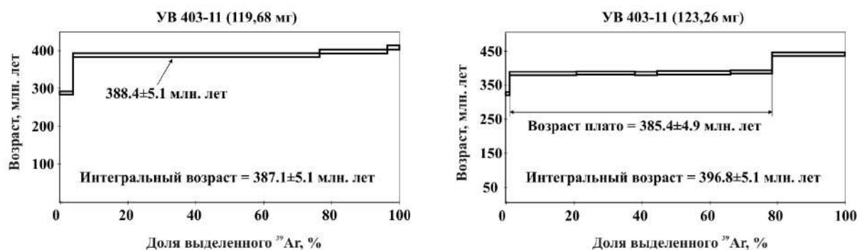
Рис. 2. ^{40}\text{Ar}/^{39}\text{Ar} возрастные спектры, полученные по сульфидной части (с некоторым содержанием джерфшерита) из основной массы кимберлита трубки Удачная-Восточная.
