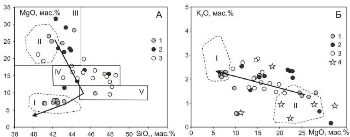
Рис. 2. Диаграммы \text{MgO} - \text{SiO}_2 (А) и \text{K}_2\text{O} - \text{MgO} (Б) для расплавных включений. Пояснения в тексте.
