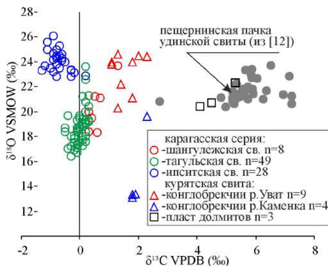
Рис. 1. Изотопно-геохимические (C, O) характеристики карбонатной составляющей позднедокембрийских пород изученного региона Присаянья.
