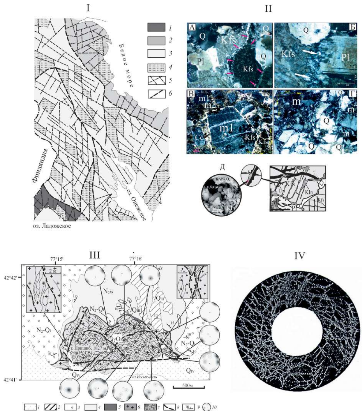
Гранулярно-блоковая инфраструктура массивов горных пород. I. Разломно-блоковая дезинтеграция мегауровня (Карельский массив) (по А.Д. Лукашову). 1–3 – геологические провинции: 1 – свекофенниды, 2 – беломорицы, 3 – Карельский массив; 4 – опущенные блоки фундамента; 5 – линеаменты и разломы; 6 – границы провинций и главные структурные линии. II. Деформация микроуровня и синтетектоническая минерализация гранитов массива Танын (Гобийский Алтай) (фото и интерпретация Е.В. Лаврушиной [5]). А, Б – кварц-полевошпатовые агрегаты (показаны стрелками) – продукт динамической рекристаллизации; В – микробрекчия с каолинит-кальцитовым матриксом; Г – микробрекчия с кластами кварца и полевого шпата в каолинит-кальцитовом матриксе; Д – развитие каолинита по трещинам спайности ортоклаза. III. Инфраструктура мезоуровня в гранитах (Тянь-Шань). Стереограммы отражают локальные поля напряжений в отдельных породных фрагментах [5]. 1 – коллювий и пролювий; 2 – лессы (верхний плейстоцен); 3–5 – горизонты и свиты палеогена – неогена; 6 – граниты (О); 7 – трещиноватость в гранитах; 8 – разломы; 9 – элементы залегания; 10 – стереограммы плотностей полюсов трещин в гранитах (нижняя полусфера). IV. Сетка напряжений, возникшая при гранулярном течении [10].
