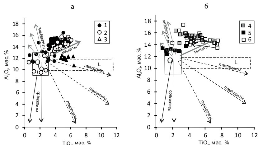
Рис. 1. Состав слюд из лампрофиров ( а ) и пород Бушканайской дайки ( б ) на диаграмме \text{Al}_2\text{O}_3 – \text{TiO}_2 . Слюды: 1 – из айлликитов, 2 – дамтьернитов, 3 – минетты, 4 – слюдяного кимберлита, 5 – оливинита, 6 – биотитового пикрита.
