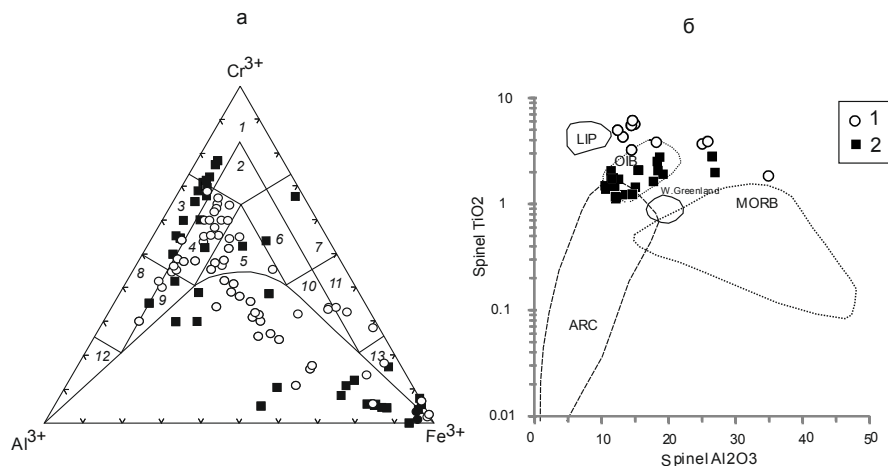
Рис. 2. Диаграмма Н.В. Павлова для шпинелидов ( а ) и дискриминационная диаграмма \text{Al}_2\text{O}_3 – \text{TiO}_2 [6] для хромшпинелидов из включений в оливине ( б ). Шпинелиды: 1 – из айлликитов, 2 – из пород Бушканайской дайки. Поля на рис. а : 1 – хромит, 2 – субферрихромит, 3 – алюмохромит, 4 – субферри-алюмохромит, 5 – ферриалюмохромит, 6 – субалюмоферрихромит, 7 – феррихромит, 8 – хромпикотит, 9 – субферрихромпикотит, 10 – субалюмохроммагнетит, 11 – хроммагнетит, 12 – пикотит, 13 – магнетит.
