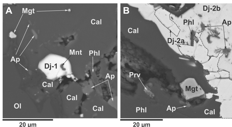
Рис. 1. Джерфишерит в основной массе исследованных кимберлитов трубки Удачная-Восточная. А – джерфишерит в виде отдельных зерен (Dj-1). В – фрагмент каймы вокруг более ранних Fe-Ni-Co-Cu-сульфидов, сложенной джерфишеритом разного состава (Dj-2а и Dj-2b). Символы: Dj – джерфишерит, Phl – флогопит, Ol – оливин, Mnt – монтицеллит, Cal – кальцит, Ap – апатит, Prv – перовскит, Mgt – магнетит.
