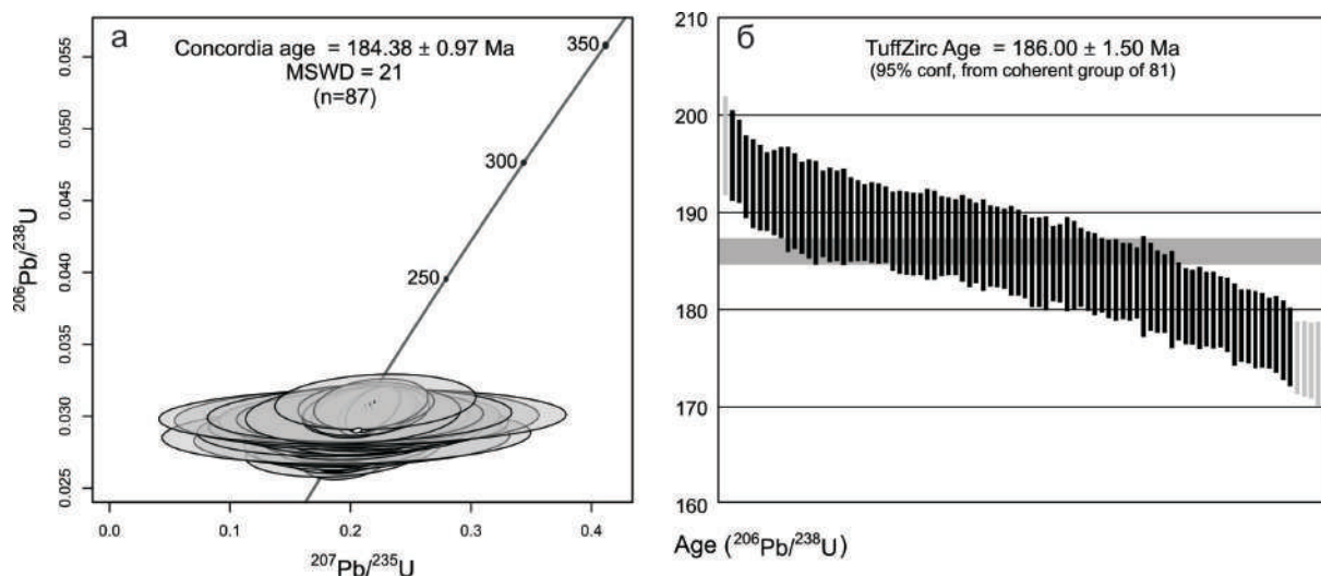
U-Pb по данные по цирконам для образца J-16-55. а – диаграмма с конкордией, возраст рассчитан по 87 зернам циркона; б – результаты, полученные с помощью алгоритма TuffZirc, выбранные и отклоненные для расчета даты показаны черным и светло-серым, соответственно; серая область соответствует датировке рассчитанной TuffZirc и ее ошибке.
