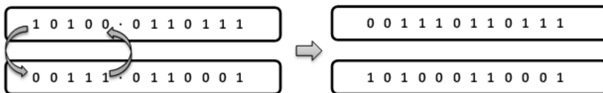
Рисунок 1. Схема одноточечного кроссинговера в генетическом алгоритме
