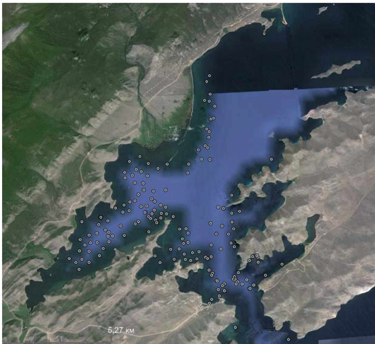
Рис. 1.4.6.5. Карта-схема обнаруженных и поднятых сетевых орудий лова в акватории Малого моря
