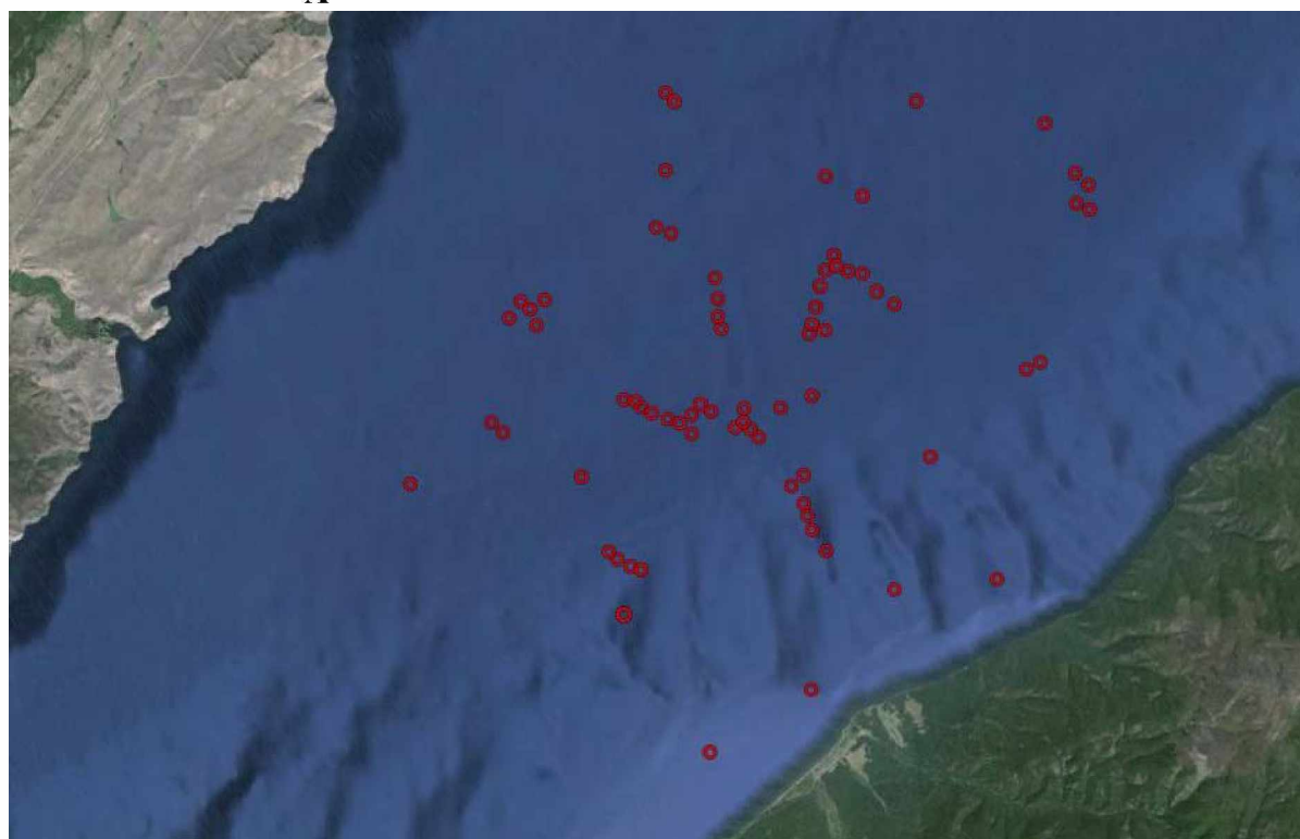
Рис. 1.1.1.5.4. Расположение логов щенных самок нерпы на Северном Байкале (А) и Среднем Байкале (Б), апрель 2013 года
