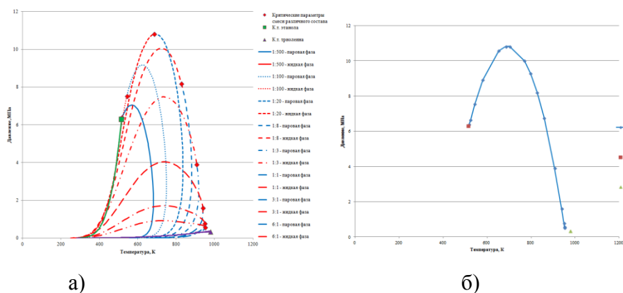
Рис. 3 – Бинодали для бинарных систем «триглицерид олеиновой кислоты - этанол» различного состава (а) и критическая линия «жидкость - пар»
