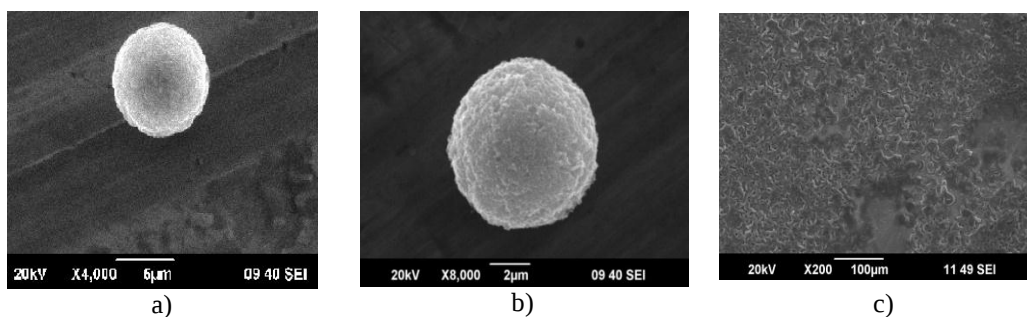
Рис. 1. Изображения микрокапсул TiO 2 в PEG8000 (фоновый газ: а)-He, b)-SF 6 и c)-CO 2 ).
