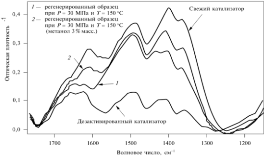
Рис. 2. ИК-спектры образцов катализатора «никель на кизельгуре», регенерированных с использованием чистого и модифицированного СК-СО 2
