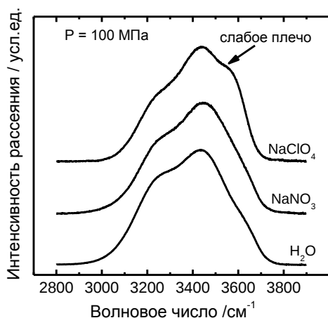
Рис.1 Спектры КР воды и водных растворов \text{NaNO}_3 (5мольн.%) , \text{NaClO}_4 (5 мольн.%).
