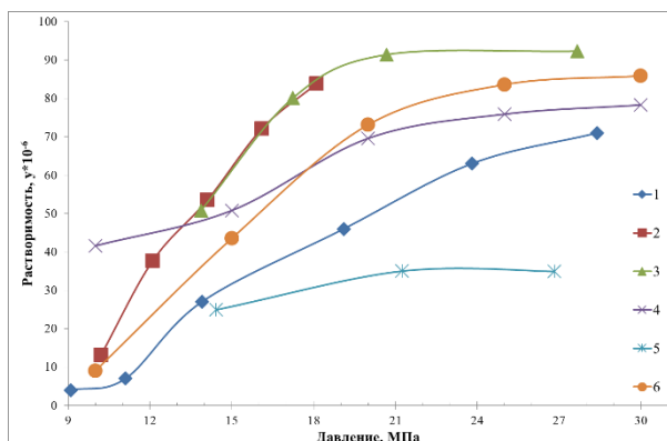
Рис. 1. Растворимость антрацена в СК CO 2 при T=308,15 \text{ K} , 1 – [2], 2 – [3], 3 – [4], 4 – [5], 5 – [6], 6 – настоящая работа.
