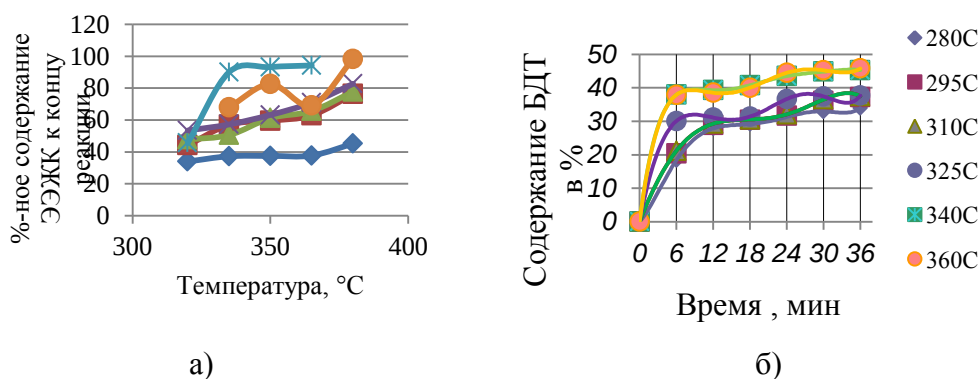
Рис. 1 Влияние характеристик процесса на величину конверсии (а) и кинетику реакции для соотношения 6:1 (б).
