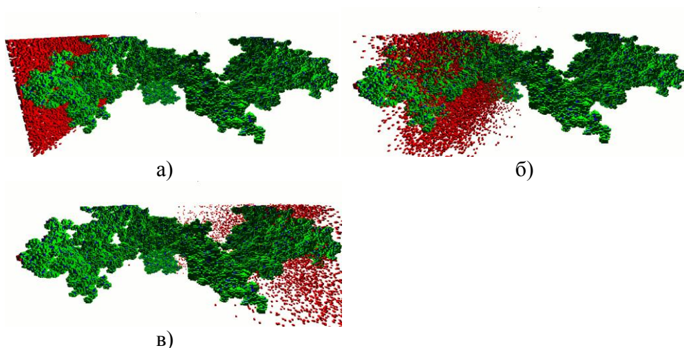
Рис.1. Процесс прохождения вещества через колонку в ходе моделирования: а) в начальный момент времени; б) в момент времени t ; в) в конце процесса
