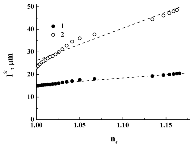
Рис.1. Зависимости транспортной длины распространения излучения (633 нм) в мезопористых слоях (на основе: 1 – волокон целлюлозы, 2 – ПТФЭ волокон), насыщенных сверхкритической двуокисью углерода (306.16 K) от показателя преломления флюида. Результат решения обратной задачи спектроскопии диффузного рассеяния.
