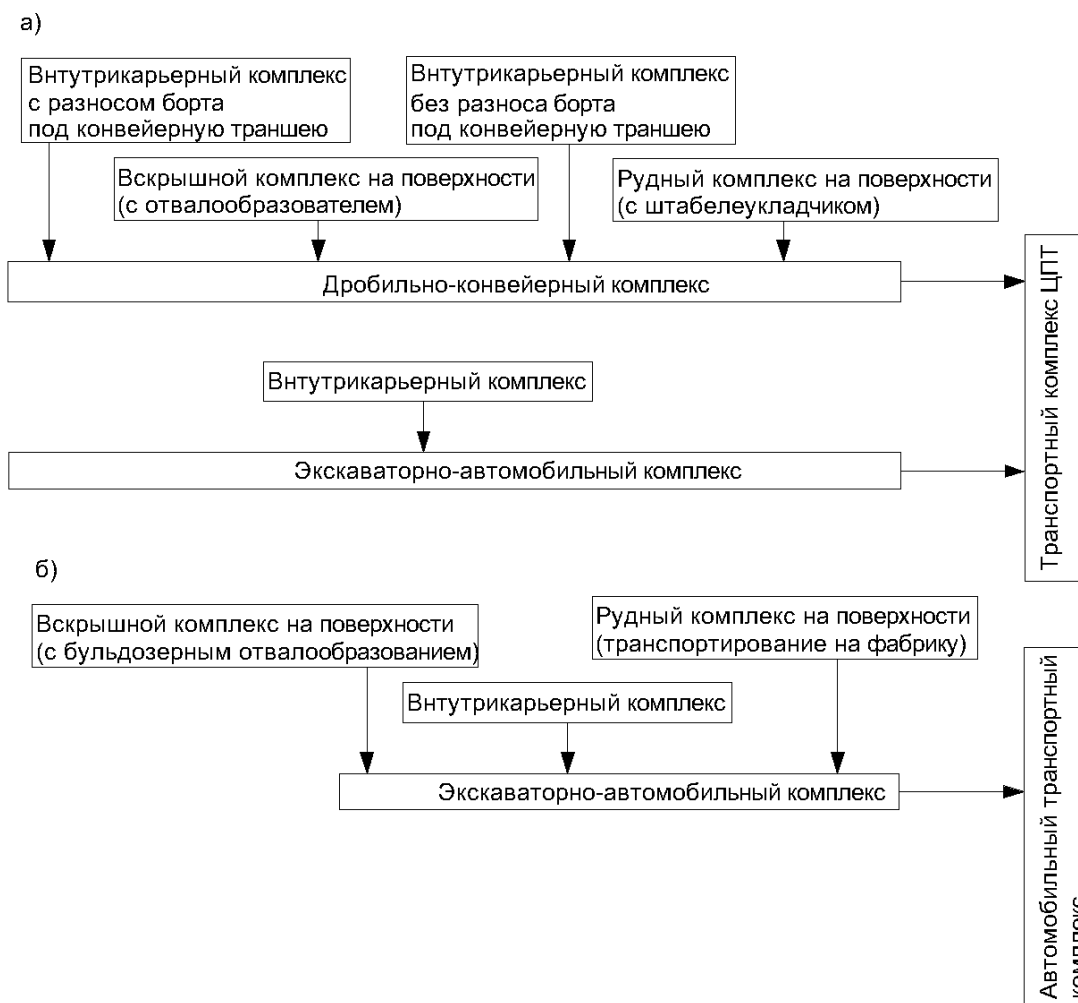
Рис. 1. Модули затрат на: а) Транспортный комплекс циклично-поточной технологии; б) Автомобильный транспортный комплекс.
