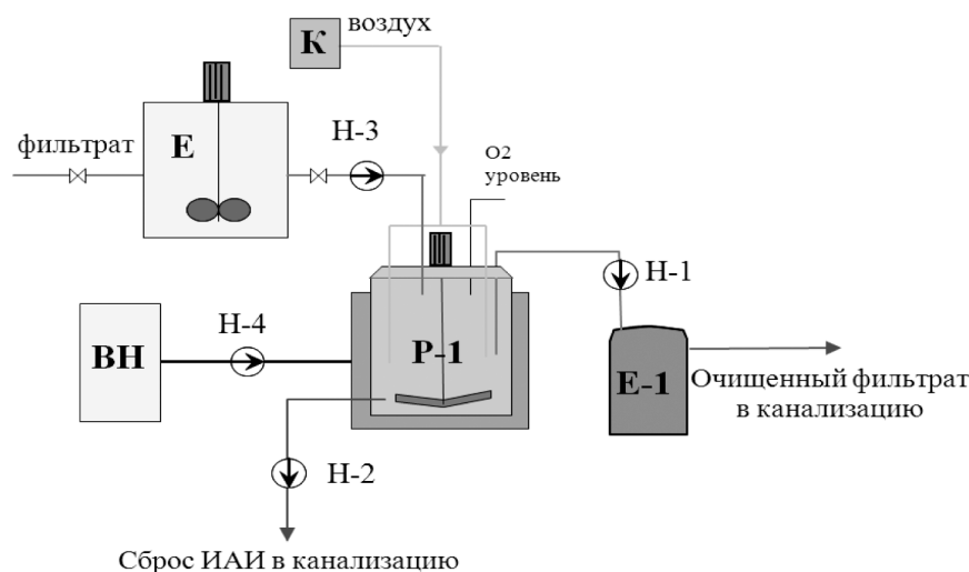
Рис. 1. Схема полупромышленной однореакторной установки Анаммокс. Условные обозначения: Е – приемная емкость исходного субстрата; Р – реактор одновременной автотрофной нитрификации-денитрификации (частичная нитрификация и аноксидное окисление аммония); К – компрессор; ВН – водонагреватель; Н-1 – Н-4 – насосы, Е-1 – емкость для сбора очищенной воды.
