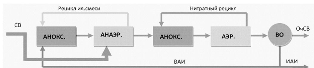
Рис. 1. Технологическая схема MISAN.
