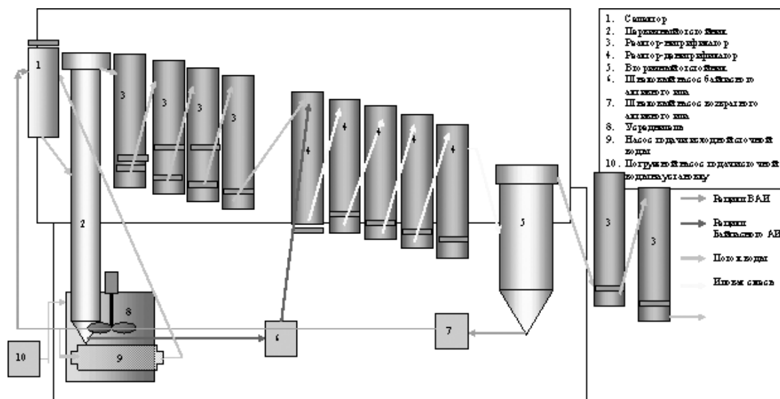
Рис. 1. Схема пилотной установки «М-Дефанокс».
