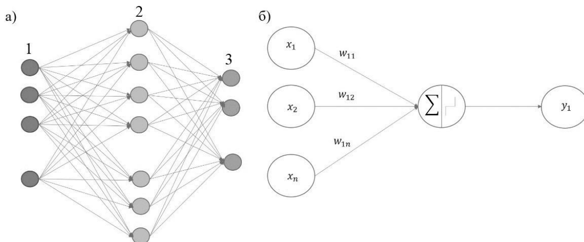
Рис. 1. Схема искусственной нейронной сети с одним скрытым слоем (а) и перцептрона (б): 1 – нейроны входного слоя; 2 – нейроны скрытого слоя; 3– нейроны выходного слоя; х – входной сигнал; w – веса нейронных связей; у – выходной сигнал
