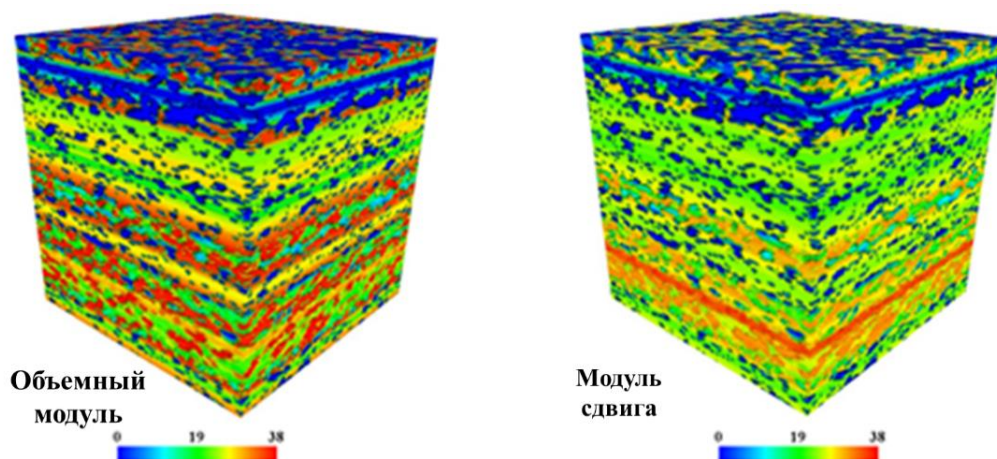
Рис. 1. Схема распределения модуля упругости трехмерного цифрового ствола скважины в интервале 2400,00-2407,35 м
