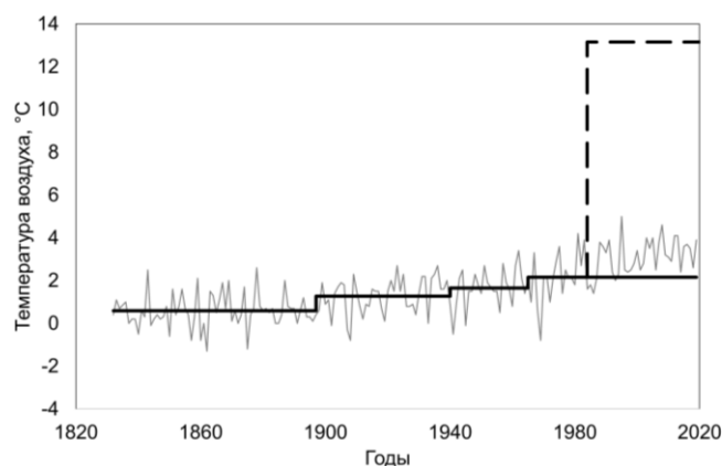
Рис. 2. Изменения среднегодовой температуры приземного воздуха на метеостанции Екатеринбурга (тонкая серая кривая) и аппроксимация вариаций температуры в отсутствии здания (сплошная черная линия) и после его строительства (штриховая черная линия)
