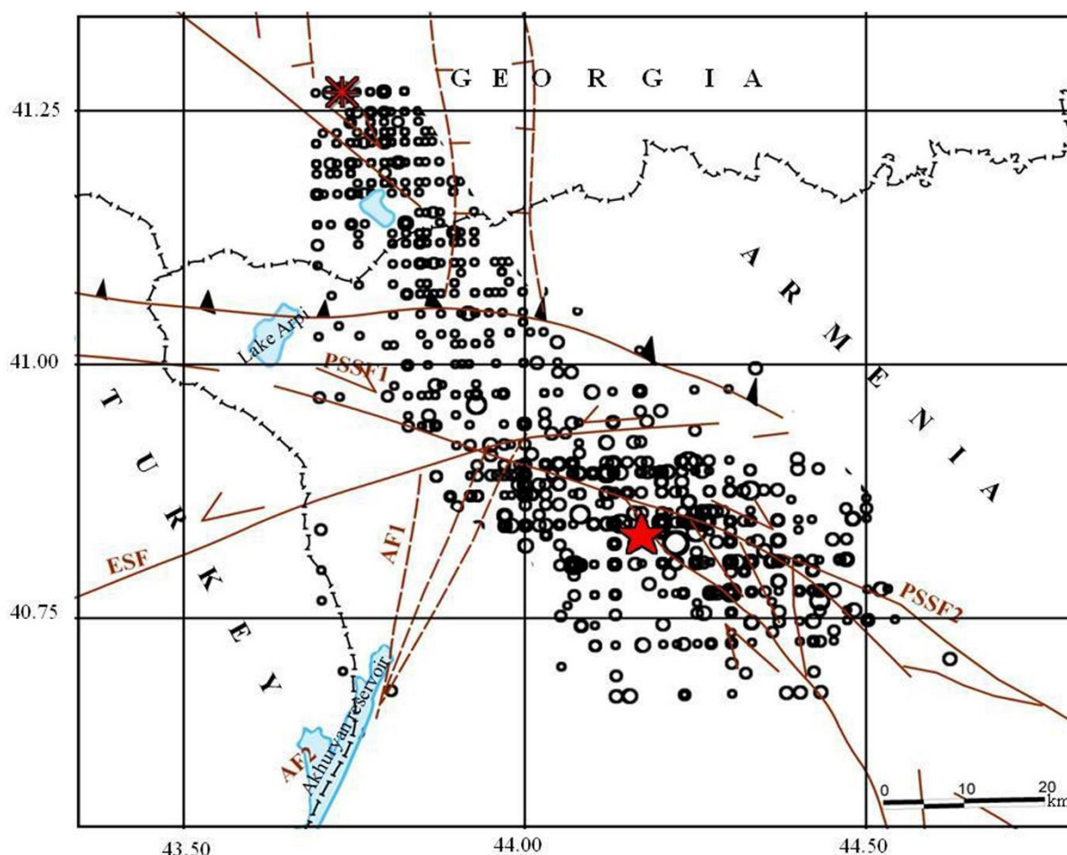
Рис. 1. Пространственное распределение афтершоков Спитакского землетрясения
