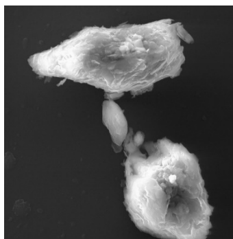
«б» – (\text{Al/Fe/Ti/Mg/K})_x\text{O}_y
