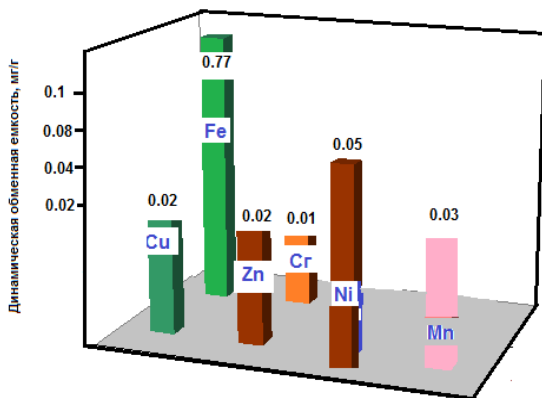
Рис. 4. Динамическая обменная емкость до проскока нанопористого окисленного углеродного сорбента (НУМС-О) по ионам \text{Fe}^{2+} , \text{Cu}^{2+} , \text{Zn}^{2+} , \text{Ni}^{2+} , \text{Cr}^{6+} и \text{Mn}^{2+} при pH раствора сорбата 5,5-6.
