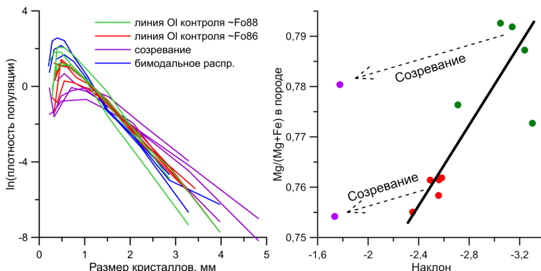
Рис. 1. а) распределение кристаллов оливина по размерам (CSD), б) прямая зависимость крутизны наклона графика CSD от отношения \text{Mg}/(\text{Mg}+\text{Fe}) в породе. Укрупнение популяции приводит к отходу от тренда.
