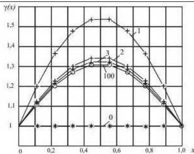
Рис. 3. Параболическое распределение коэффициента теплопроводности \gamma(x) : слева — заданное точное распределение (сплошная линия) и нулевое приближение (звездочки); справа — итерационные приближения (номер кривой соответствует номеру итерации)
