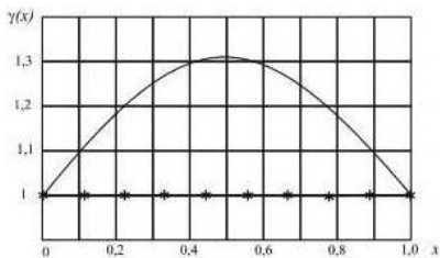
Рис. 3. Параболическое распределение коэффициента теплопроводности \gamma(x) : слева — заданное точное распределение (сплошная линия) и нулевое приближение (звездочки); справа — итерационные приближения (номер кривой соответствует номеру итерации)
