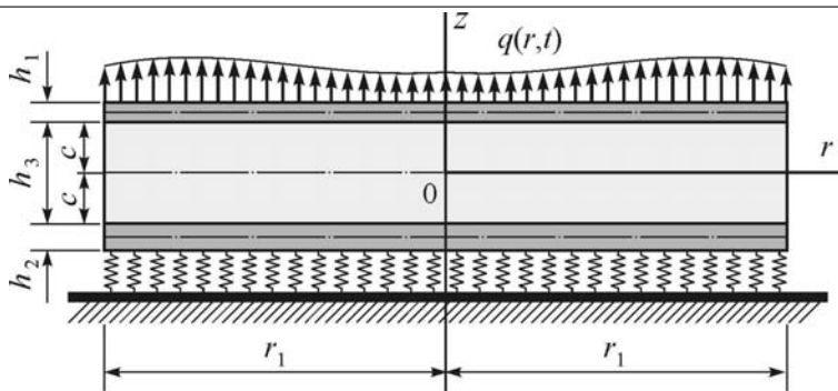
Рис. 1. Расчетная схема
