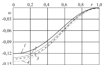
Рис. 3. Термоупругопластический прогиб
