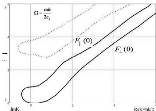
Рис. 1. Пример дисперсионных кривых низших мод колебаний упругой пластины
