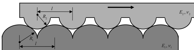
Рис. 7. Схема скольжения двух шероховатых поверхностей.
