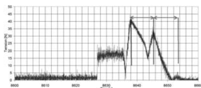
Рис. 6. Экспериментально замеренное изменение натяжения троса на катушке при окончании размотки.
