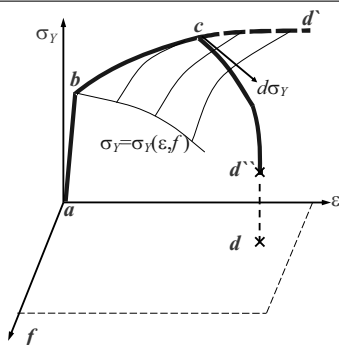
Рис. 2. Нагружения и разрушения в трехмерном пространстве
