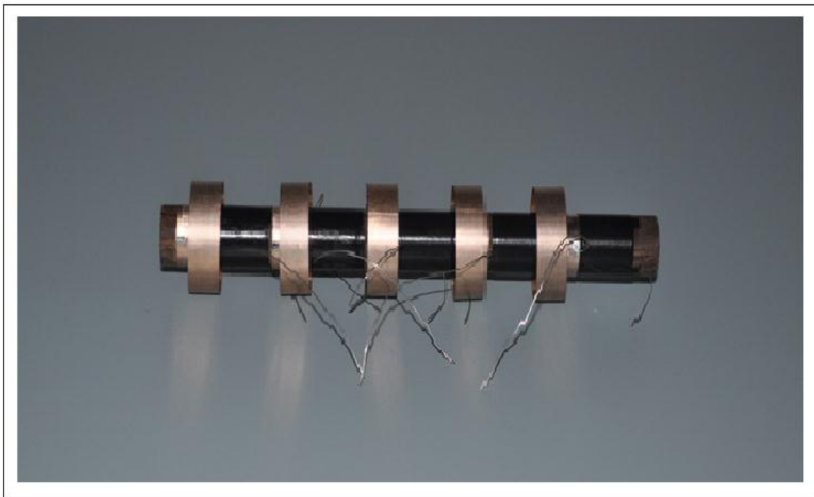
Рис. 4. Последовательное и соосное расположение активных модулей в усилителе А.Ю. Смирнова.
