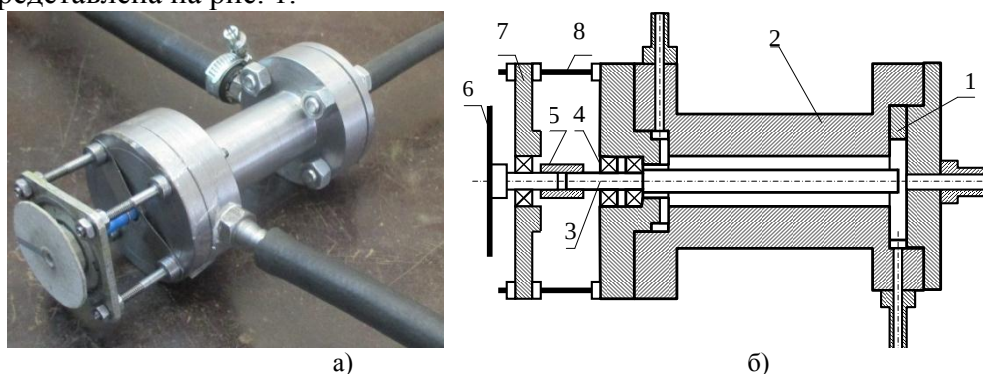
Рис. 1. Вихревое устройство: а) общий вид, б) принципиальная схема.
