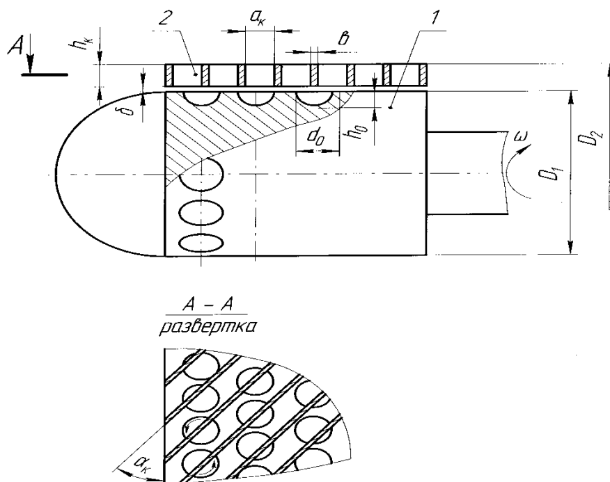
Рис. 4. Схема вихревой гидромашины с цилиндрическим ротором.
