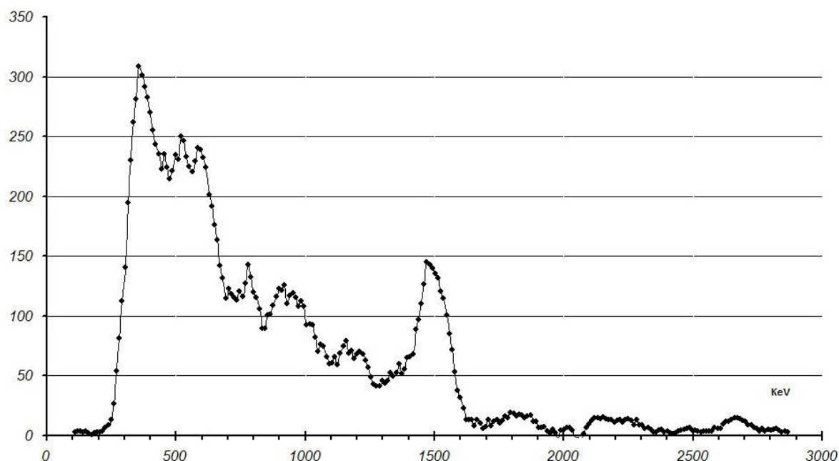
Рис. 6. Спектр гамма – излучения образца минерала красного гранита, не подвергавшегося ранее ВНП прибора «НГК-ВЕГА» и являющегося образцом сравнения. Спектр получен сцинтилляционным спектрометром на основе кристалла CsJ(Tl).
