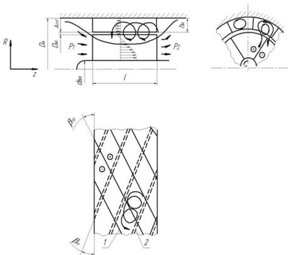
Рис. 2. Схема течения жидкости в каналах осевихврового насоса. 1 – лопастное осевое колесо, 2 – лопасти неподвижной винтовой решетки. Неподвижные лопасти условно показаны штриховыми линиями; подвижные лопасти показаны сплошными линиями.
