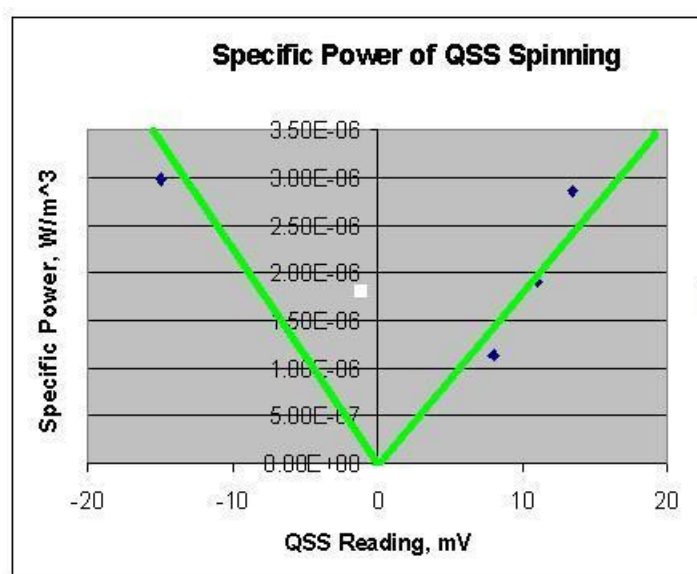
Рис. 2. Калибровка аппарата SEVA-Integral-M-3 для квазистационарного вращения ПГ на фиксированной частоте 100 кГц. Крутизна преобразования составляет (1.5 \cdot 10^{-7} \text{ W/m}^3)/\text{mV} для положительных значений отсчёта и (2.0 \cdot 10^{-7} \text{ W/m}^3)/\text{mV} для отрицательных значений отсчёта.
