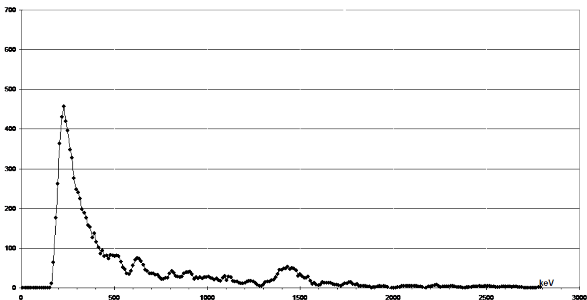
Рис. 7. Спектр гамма – излучения образца минерала красного гранита, подвергнутого ранее ВНП прибора «НГК-ВЕГА». Спектр получен сцинтилляционным спектрометром на основе кристалла CsJ(Tl).
