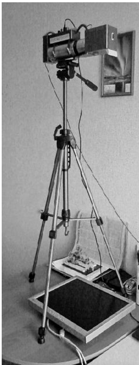
Рис. 2. Модернизированный измеритель GRG-01M1 на фотоштативе Rekam RT-M42 с монитором типа FLATRON L1810B.
