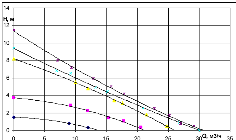
Рис. 5. Характеристики вихревой гидромашины с цилиндрическим ротором.
