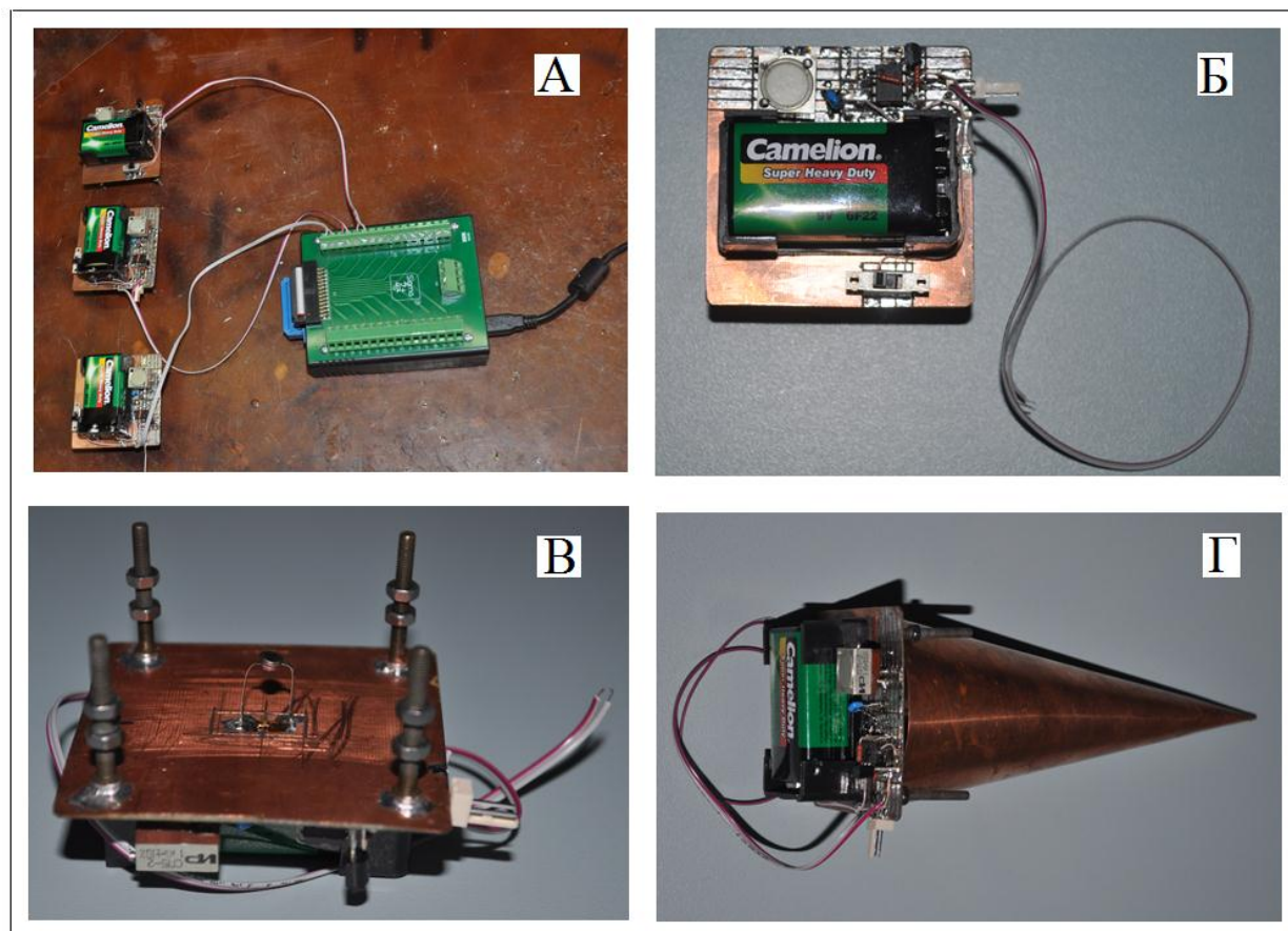
Рис. 2. Детектор фазы волновой функции на основе туннельных диодов. Обозначения: А – модуль регистрации данных Zet 210 с тремя источниками фазового шума волновой функции на основе туннельных диодов; Б – фото одного из источников; В – туннельный диод; Г – элемент системы регистрации фазы волновой функции с конусом-концентратором. Пояснения в тексте.
