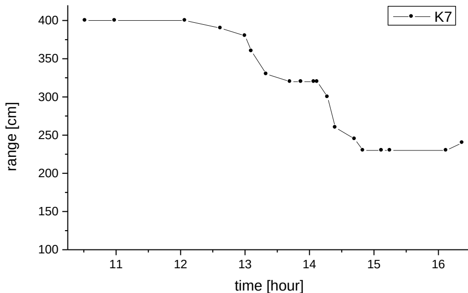
Рис. 3. Измерения изменений интенсивности Категории 7 во времени в излучении торсионного поля Солнца 21.05.2016, связанной в это время с 27-дневным циклом.
