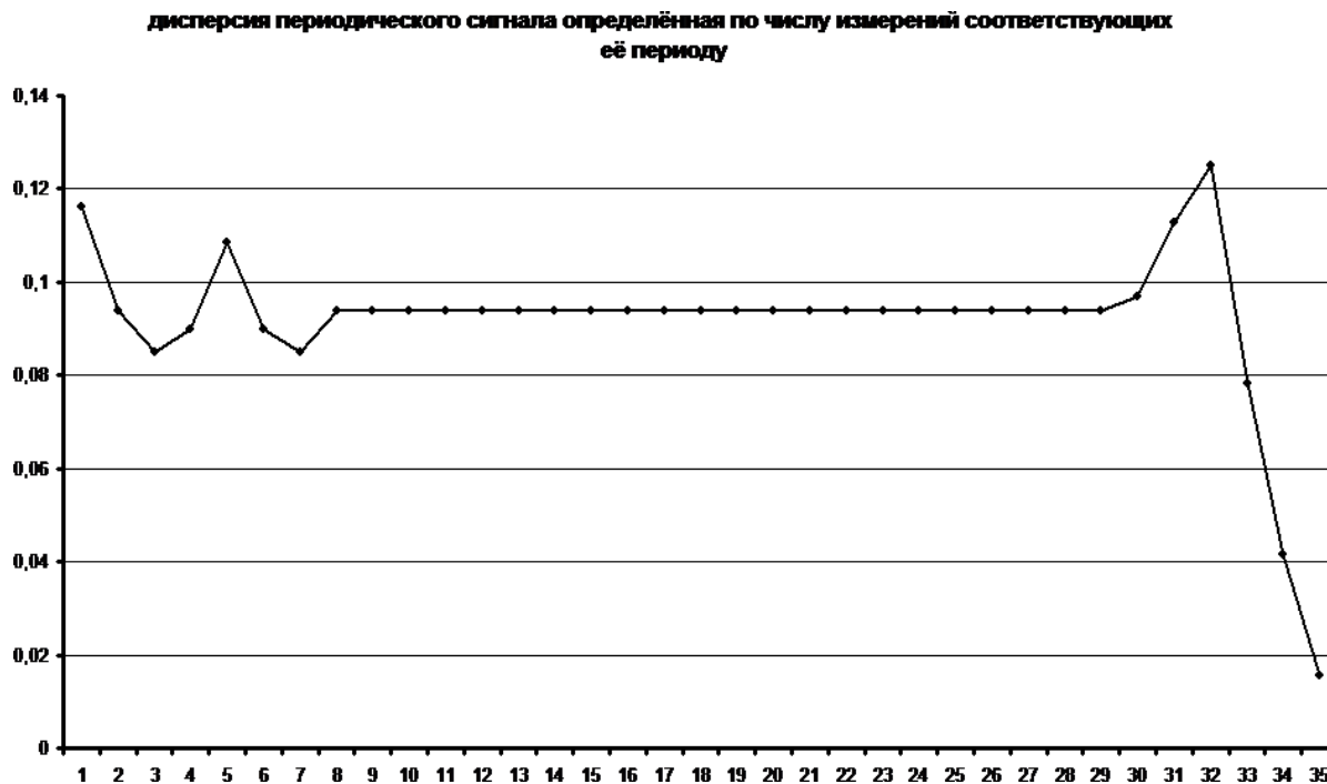
Рис. 2. Дисперсия периодического сигнала определённая по числу измерений соответствующих её периоду.
