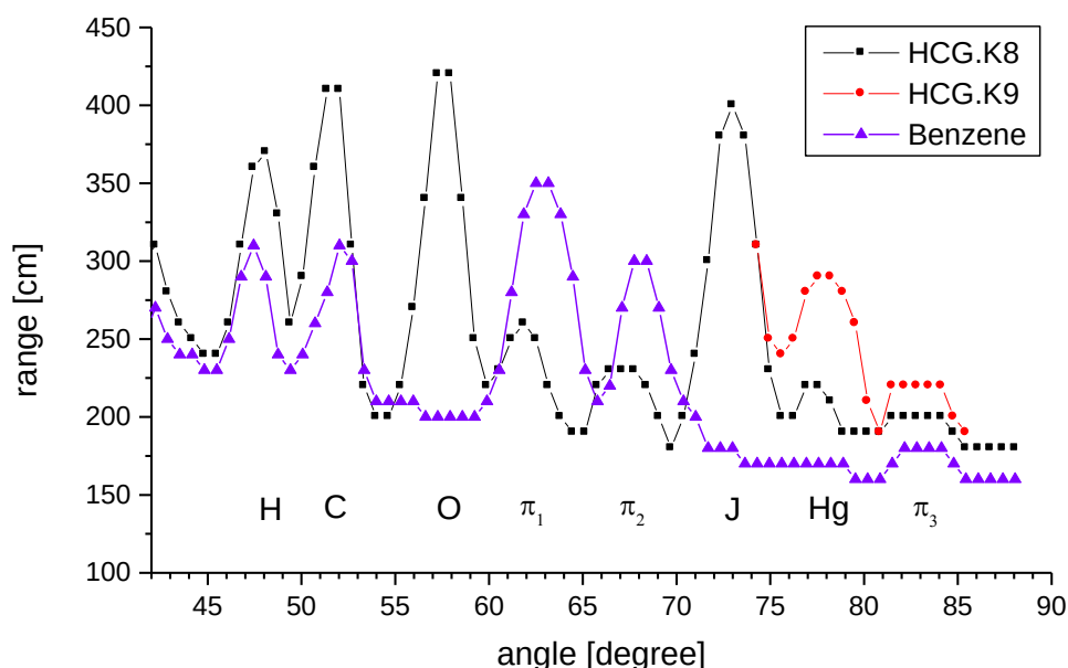
Рис. 6. Спектр препарата «Прегнил» 5000 м.е. Копия двух ампул фирмы N.V. Organon, LOT 176282. Весь график «Прегнила» был получен для самой сильной для этого препарата Категории K8. Зона пика ртути была дополнительно определена для Категории K9 для выделения присутствия этого элемента. Также был показан спектр бензола, как сравнительный для определения присутствия ароматических колец. Ось абсцисс – угол падающего пучка с перспективы преломляющей плоскости, измеряемый в градусах, ось ординат – зона излучения из проб на выходе спектроскопа, измеряемая в сантиметрах.
