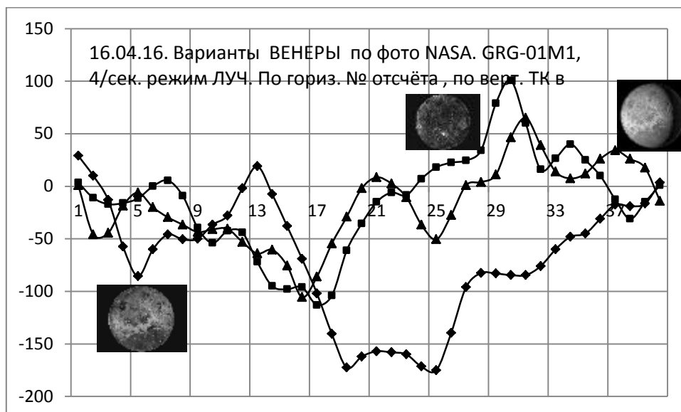
Рис. 10. Фрагменты сканирования для Венеры. Задержку распространения численно оценить можно, но скорость «освоения» определить затруднительно из-за неопределённости в расстоянии. По горизонтальной оси графиков - № отсчёта, по вертикальной оси – ТК в Ts*10 .
