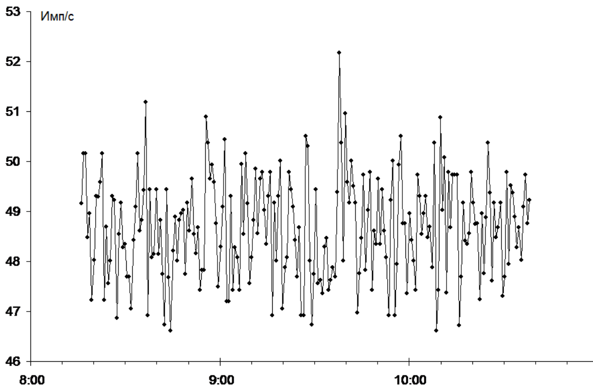
Рис. 1. Скорость счета радиометра на основе счетчика СБТ-11 с дополнительным источником альфа – излучения Pu^{239} . Регистрирование проводилось до процесса ВНП.
