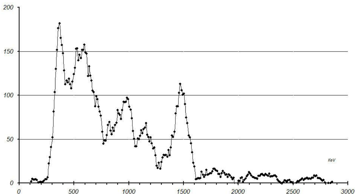
Рис. 4. Спектр гамма – излучения образца минерала красного гранита, подвергнутого ранее ВНП прибора «НГК-ВЕГА». Спектр получен сцинтилляционным спектрометром на основе кристалла CsJ(Tl).
