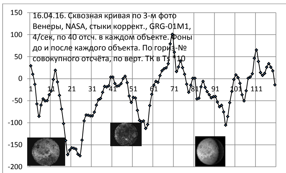
Рис. 11. Сквозная развёртка расстояния до Венеры. По горизонтальной оси - № отсчёта, по вертикальной оси ТК в Ts*10 .
