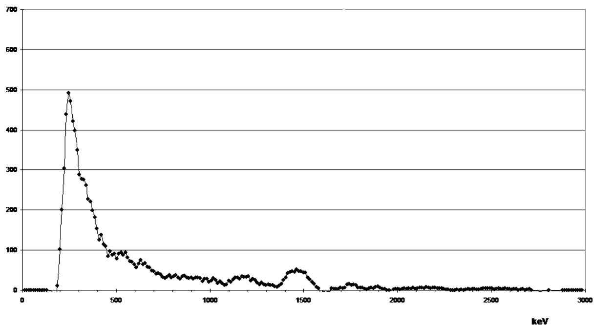
Рис. 8. Спектр гамма – излучения образца минерала красного гранита, находящегося на расстоянии 5-ти метров от источника ВНП. Спектр получен сцинтилляционным спектрометром на основе кристалла CsJ(Tl).
