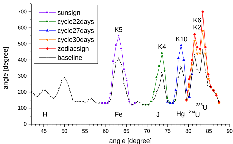
Рис. 4. Спектр торсионных полей, доходящих с Солнца, выполненный спектроном торсионных полей с архивной пробы от 27 августа 2011 г. Ось абсцисс – угол падающего пучка с перспективы преломляющей плоскости, измеряемый в градусах, ось ординат – зона излучения из проб на выходе спектрофона, измеряемая в сантиметрах.
