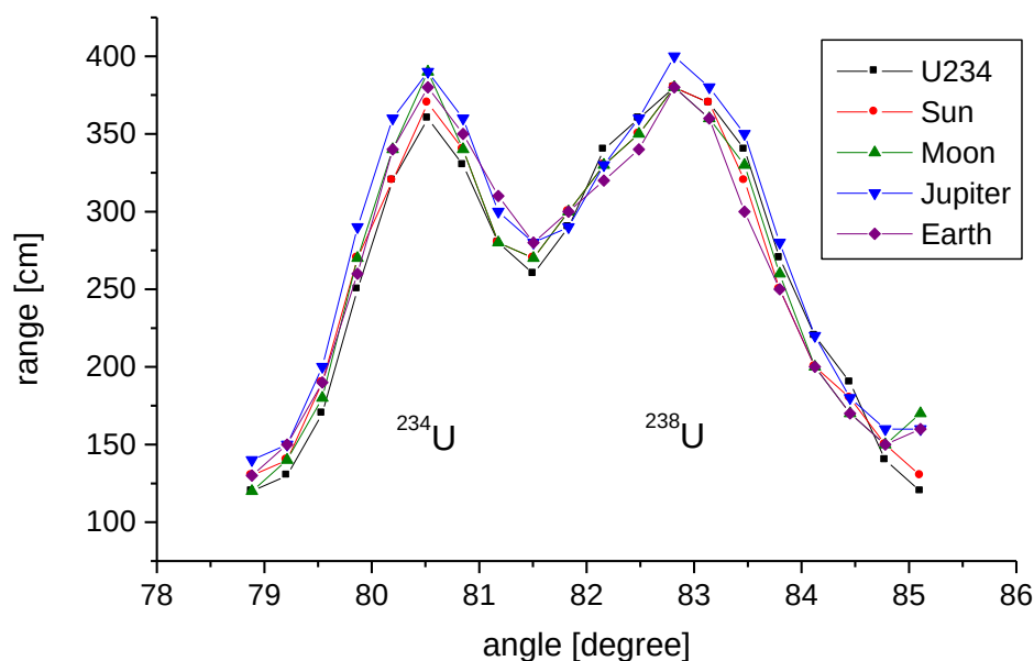
Рис. 5. Сравнение сигнала урана в доходящем торсионном поле: с излучения ацетата уранила (K8) - U234; с Солнца (6.09.2012, K6) - Sun; с Луны (6.09.2011, K10) - Moon; с Юпитера (1.10.2011, K2) - Jupiter; из глубины Земли (15.06.2016, K6) Earth. Ось абсцисс – угол падающего пучка с перспективы преломляющей плоскости измеряемый в градусах, ось ординат – зона излучения из проб на выходе спектроскопа, измеряемая в сантиметрах.
