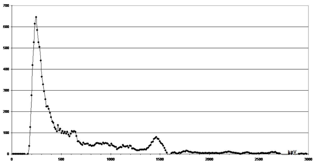
Рис. 9. Спектр гамма – излучения образца минерала красного гранита, не подвергавшегося ранее ВНП прибора «НГК-ВЕГА» и являющегося образцом сравнения. Спектр получен сцинтилляционным спектрометром на основе кристалла CsJ(Tl).
