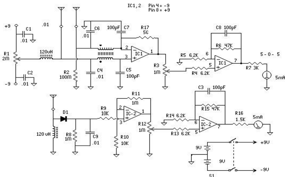
Рис. 1. Принципиальная схема прибора для обнаружения ГПЗ.
