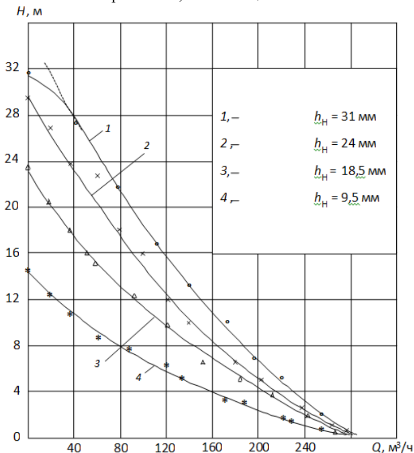
Рис. 3. Зависимости напора ОВН от подачи с различными неподвижными решетками лопастей, отличающихся высотой.
