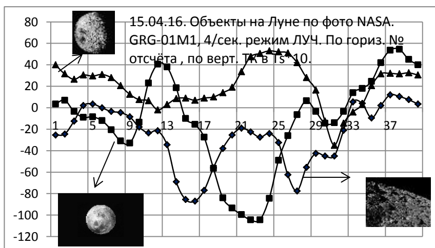
Рис. 5. Работа по фрагментам Луны. Первый свал в отрицательную область на 12 отсчёте первого фрагмента (справа внизу). Если вычсть «мёртвую зону» в 7 отсчётов, то останется 5 отсчётов, что с учётом темпа 4 отсчёта в секунду даёт 1,25 сек. Округляя до целых, получаем задержку до Луны 1 сек. По горизонтальной оси № отсчёта, по вертикальной оси торсионный контраст ТК в Ts \cdot 10 .
