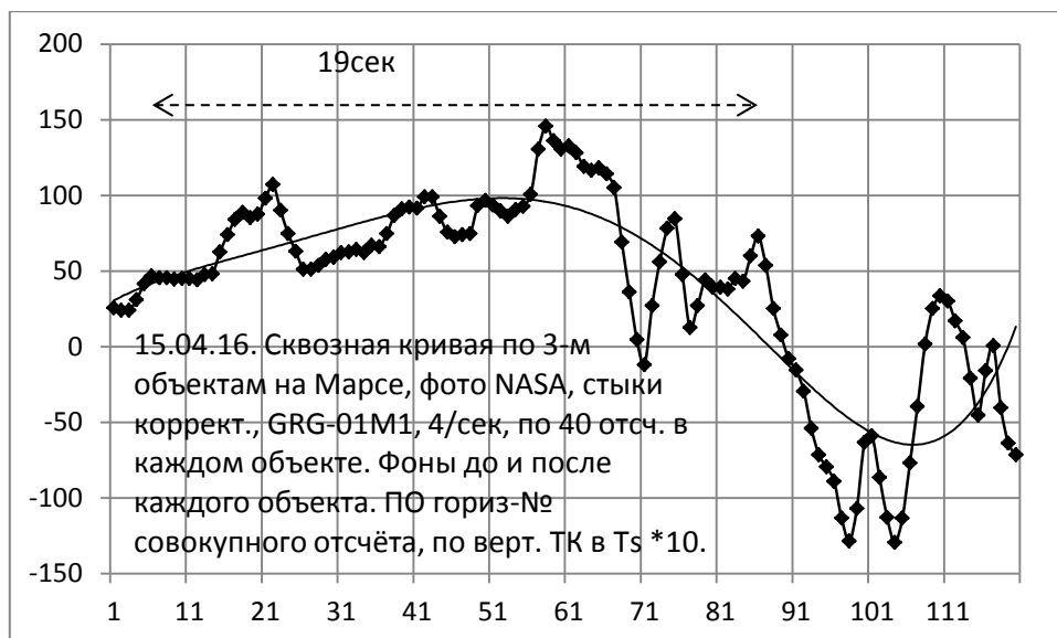
Рис. 7. Сканирование расстояния до Марса. Тонкая линия – полиномиальный тренд. По осям соответственно, № отсчёта и ТК в Ts \cdot 10 .
