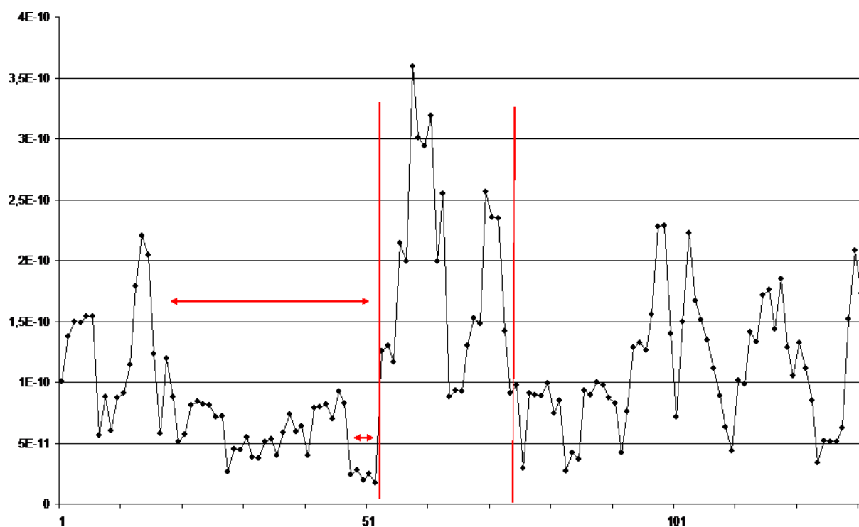
Рис. 2. Относительная дисперсия, вычисленная по пяти ближайшим измерениям. Вертикальными линиями показан участок ВНП. Горизонтальными линиями со стрелками показан эффект «предвидения».
