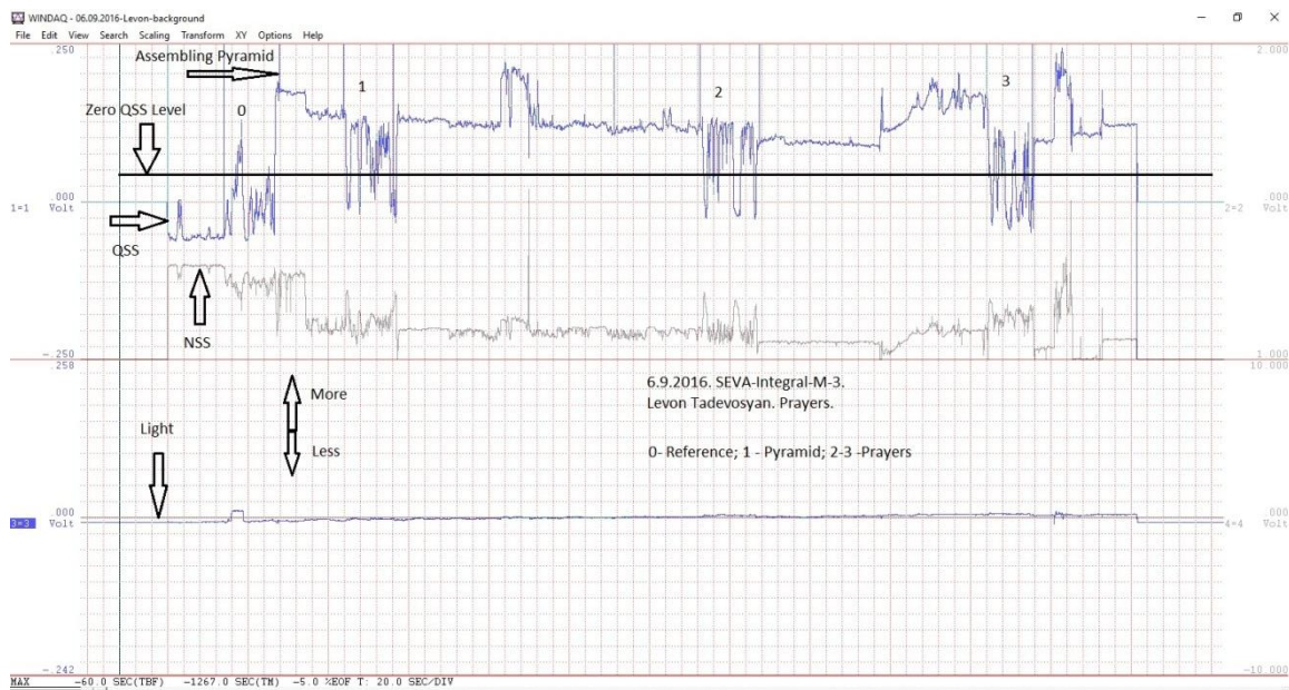
Рис. 4. Участник эксперимента Левон Тадевосян. После завершения исходного нулевого цикла над головой в расслабленном состоянии участник начал собирать небольшую картонную пирамиду. Прибор SEVA регистрирует повышение фонового уровня вращения. При этом фотометр показывает увеличение светового потока в течение 18 секунд. 1 -Пирамида приложена к телу, сканирование; 2, 3 - различные молитвы. При молитвах 2, 3 прибор фиксирует незначительное увеличение светового потока, нижняя кривая.
