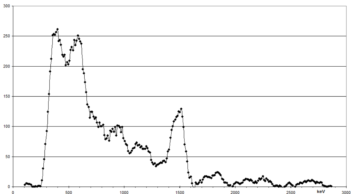
Рис. 5. Спектр гамма – излучения образца минерала красного гранита, находящегося на расстоянии 5-ти метров от источника ВНП. Спектр получен сцинтилляционным спектрометром на основе кристалла CsJ(Tl).
