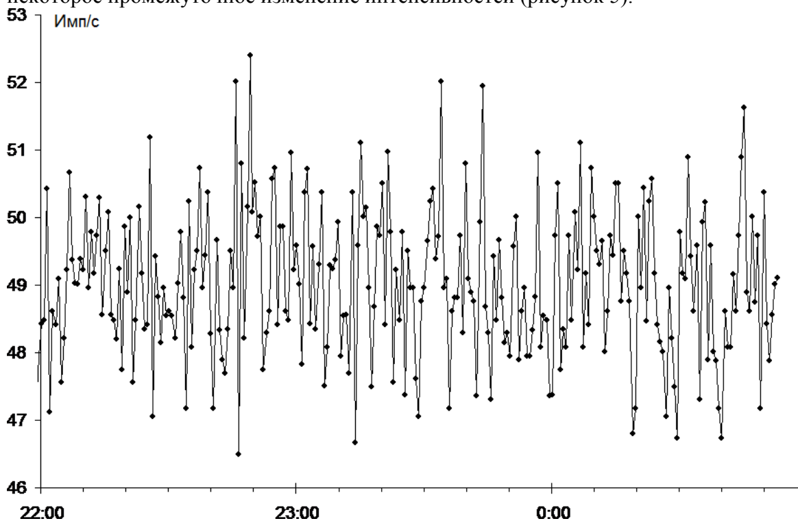
Рис. 3. Скорость счета радиометра на основе счетчика СБТ-11 с дополнительным источником альфа – излучения Pu^{239} . Регистрирование проводилось после процесса ВНП.
