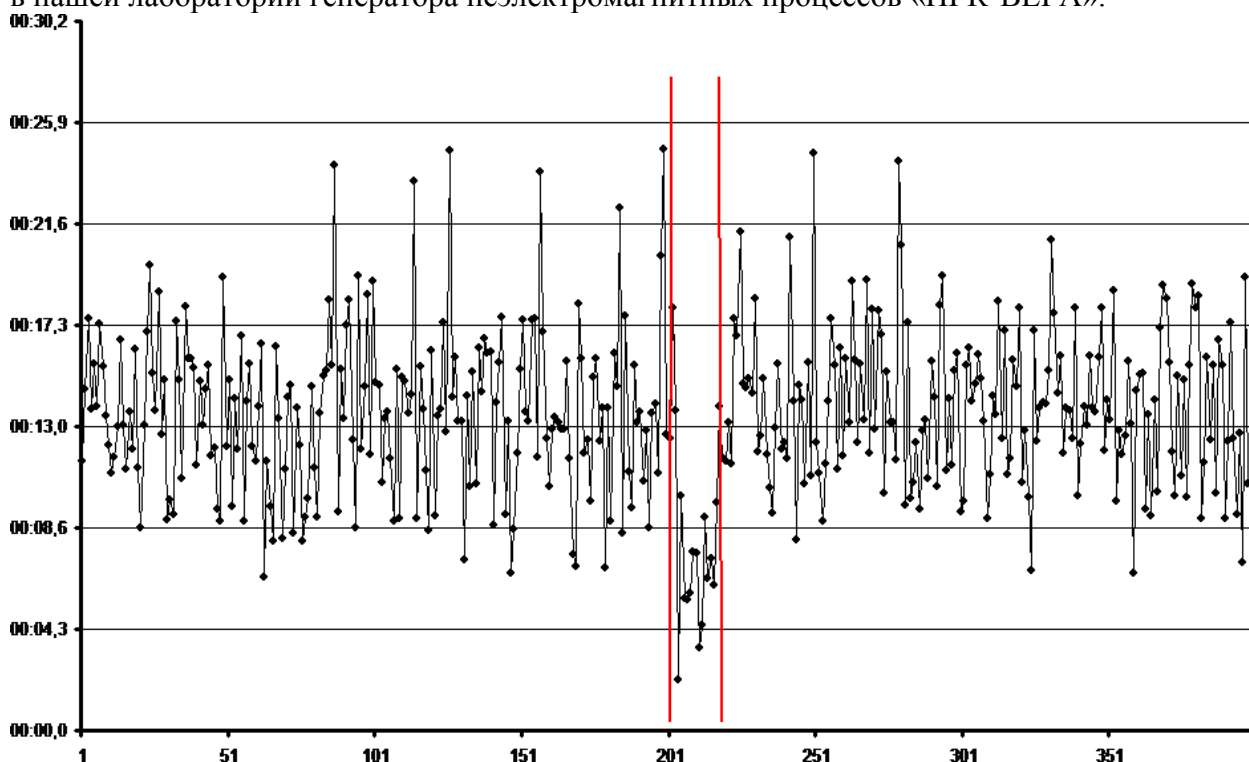
Рис. 1. Регистрируемый сигнал, представляющий собой временной ряд событий - промежутков времени набора рецепторной системой строго заданного числа регистрируемых радиоактивных частиц, параметр обратный скорости счета. Вертикальными линиями отмечен участок генерирования структурообразующего НИП прибора «НГК-ВЕГА».
