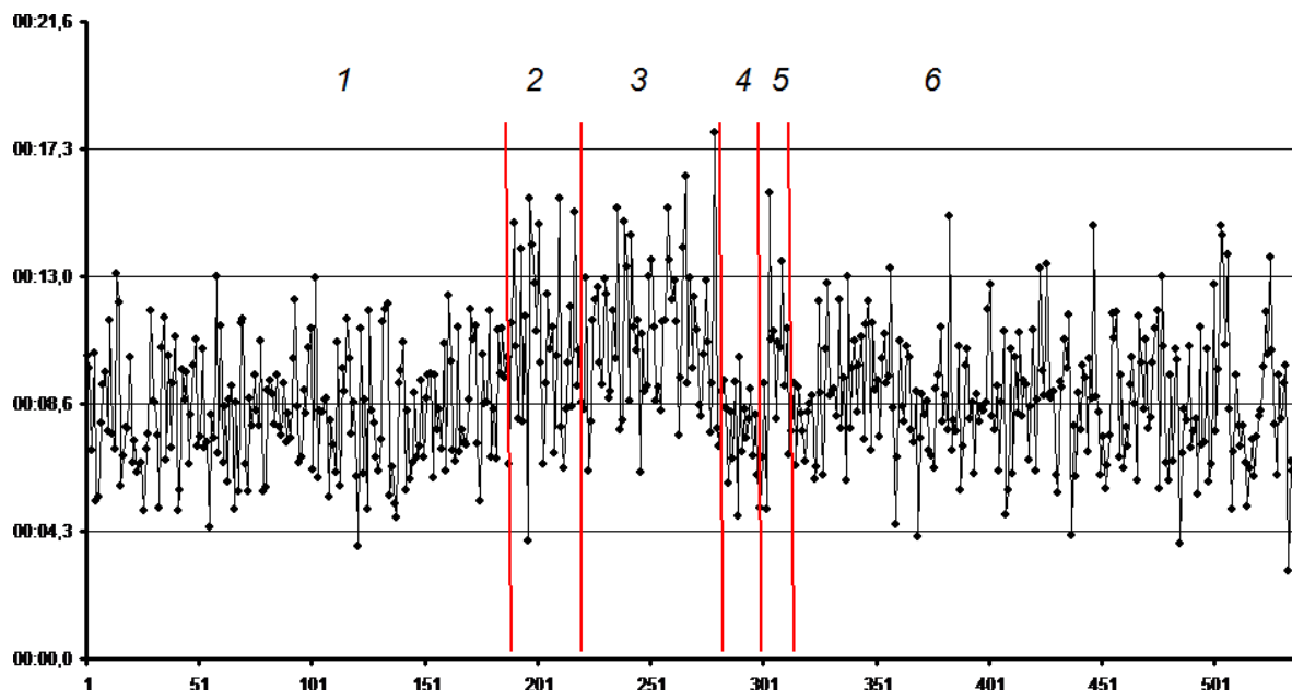
Рис. 3. Регистрируемый сигнал, представляющий собой временной ряд событий - промежутков времени набора рецепторной системой строго заданного числа регистрируемых радиоактивных частиц, параметр обратный скорости счета. Вертикальными линиями отмечены участки эксперимента. Участок 3 соответствует генерированию НИП прибора «НГК-ВЕГА» функционирующего в режиме АБИЭ.
