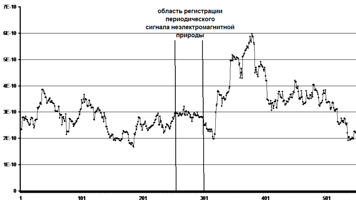
Рис. 3. Относительная дисперсия регистрируемого сигнала. Вертикальными линиями отмечен участок регистрации модулированного периодического неэлектромагнитного сигнала.
