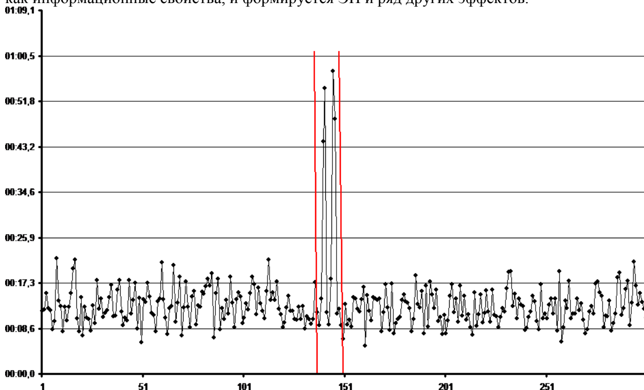
Рис. 2. Регистрируемый сигнал, представляющий собой временной ряд событий - промежутков времени набора рецепторной системой строго заданного числа регистрируемых радиоактивных частиц, параметр обратный скорости счета. Вертикальными линиями отмечен участок генерирования деструктурирующего НИП прибора «НГК-ВЕГА».
