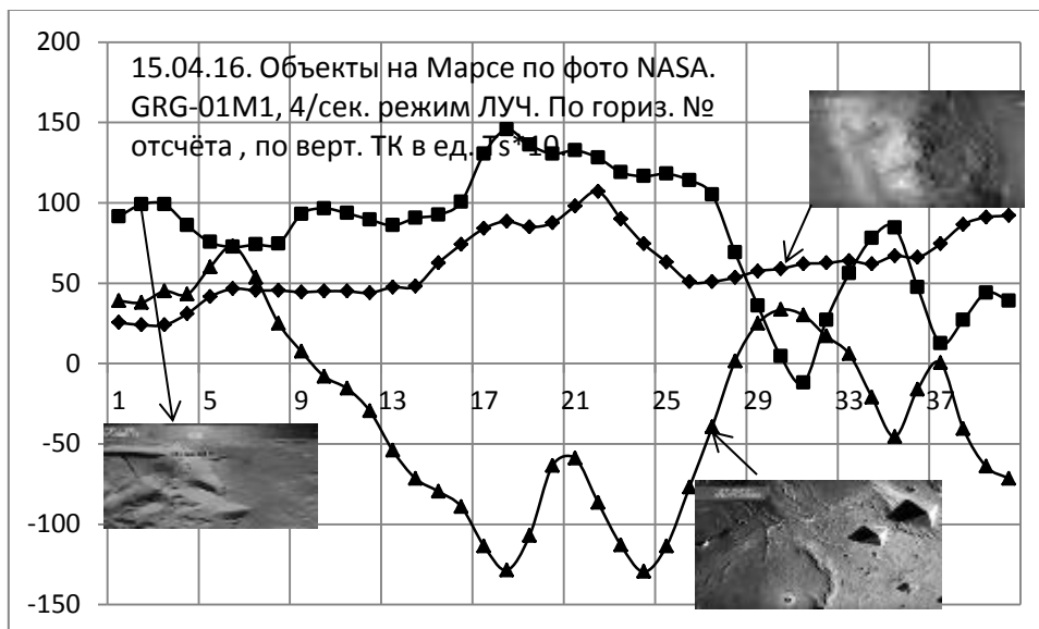
Рис. 4. К методике исследования распределения скоростей в функции расстояния. Работа по трём фрагментам Марса в отдельности. 1 проход – средняя кривая, 2 проход - верхняя кривая, 3 проход – нижняя кривая.
