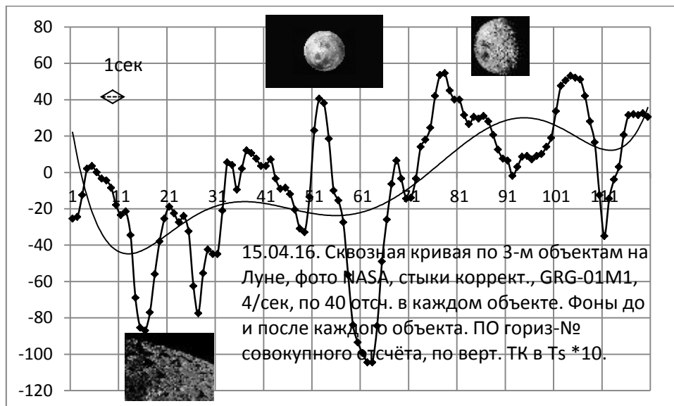
Рис. 6. Сквозная развёртка по всем трём фрагментам Луны. Видны повторы ситуации и более детальный анализ объекта Луна. Тонкая линия – полиномиальный тренд. По горизонтальной оси № отсчёта, по вертикальной оси ТК в Ts \cdot 10 .
