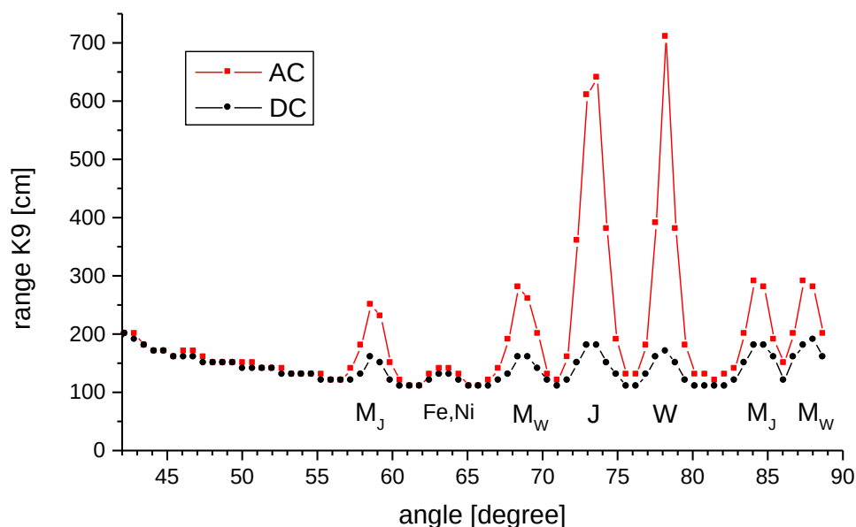
Рис. 7. Спектр галогенной лампочки Livarnolux 42W, 230V, питающейся переменным током (AC) и постоянным током (DC). В обоих случаях интенсивность освещения составляла 230 лк. Копирование сигнала с лампочки с расстояния 30 см ускорителем для исследования излучения Солнца, используя в обоих случаях такое же время копирования. MJ – сигнал йода, модулированный частотой 50Hz, Fe, Ni – сигнал железа и никеля, MW – сигнал вольфрама, модулированный частотой 50Hz, J – сигнал йода, W – сигнал вольфрама. Ось абсцисс – угол падающего пучка с перспективы преломляющей плоскости
