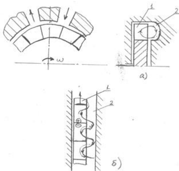
Рис. 1. Схема течения жидкости в вихревом насосе. 1 – рабочее колесо, 2 – боковой канал Первый рисунок на Рис. 1 – общий вид; а) - разрез общего вида; б) – его развертка.
