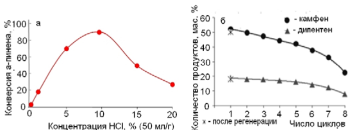
Рис. 1. Зависимость конверсии \alpha -пинена от концентрации модификатора (6 ч реакции) (а) и количества камфена и дипентена от числа циклов работы катализатора (б)
