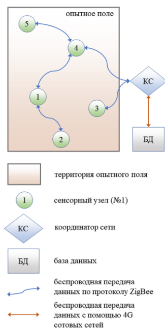
Рис. 1. Архитектура передачи данных в сенсорной сети
