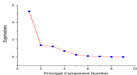
Рис. 1. Кривая осыпи
