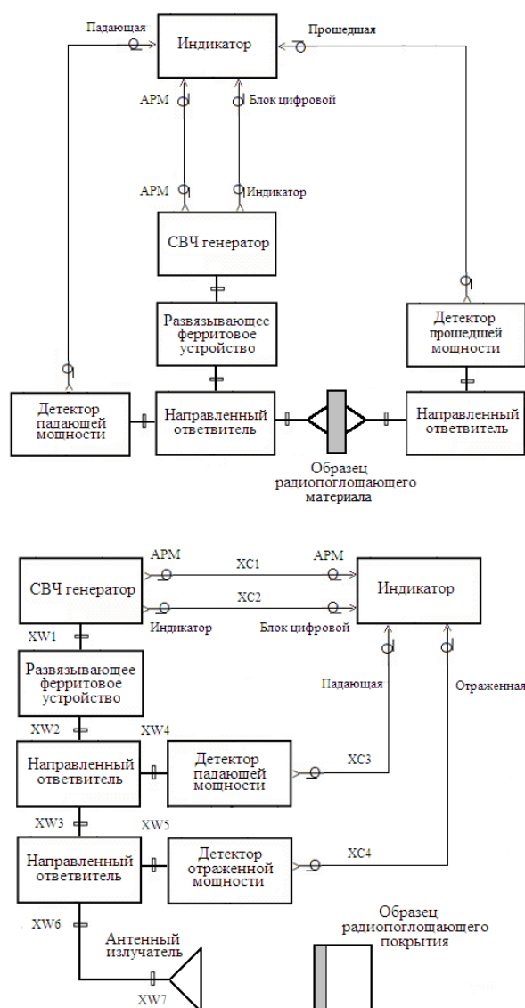
Рис.1. Структурные схемы измерения ослабления и коэффициента отражения электромагнитной волны углеродными наноматериалами.
