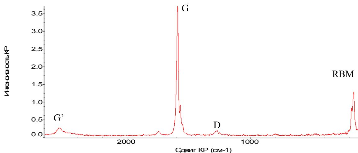
Рис. 2. Спектр комбинационного рассеяния углеродных наноматериалов
