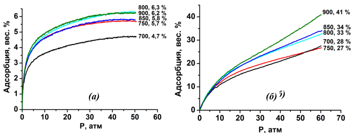
Рис. 1. Изотермы адсорбции водорода (77 К) (а) и метана (273 К) (б) на микропористых углеродных материалах из РШ.
