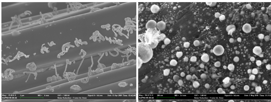
Рис. 1. Фрагмент поверхности углеродного волокна с нанесенным катализатором (Ni) и углеродного волокна декорированного УНТ.
