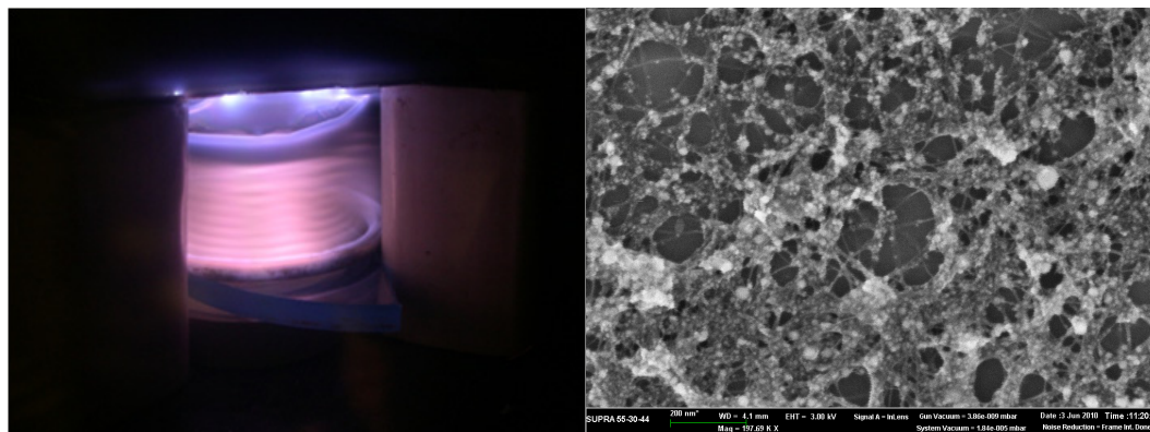
Рис. 1. Магнетронный разряд в установке CVD синтеза углеродных нанотрубок и структура формируемых горизонтально упорядоченных УНТ
