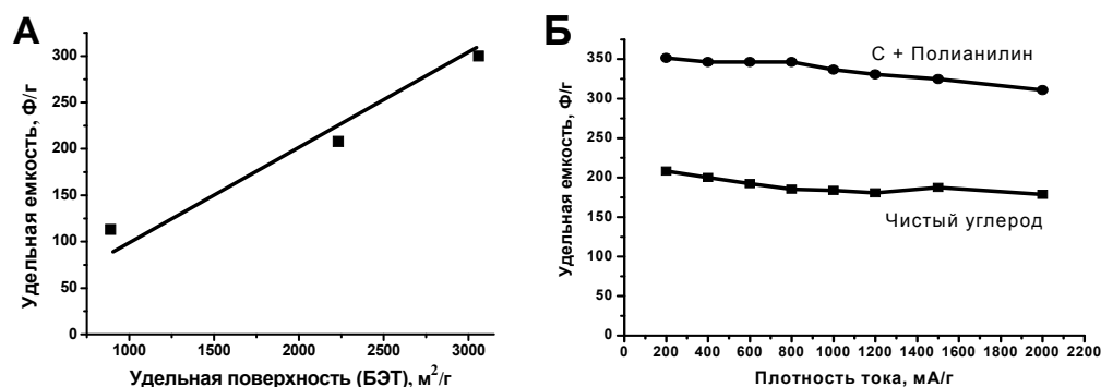
Рисунок 1. (А) Соотношение между удельной емкостью и удельной поверхностью. (Б) зависимость удельной емкости от плотности тока разряда для чистого и модифицированного полианилином углерода с
