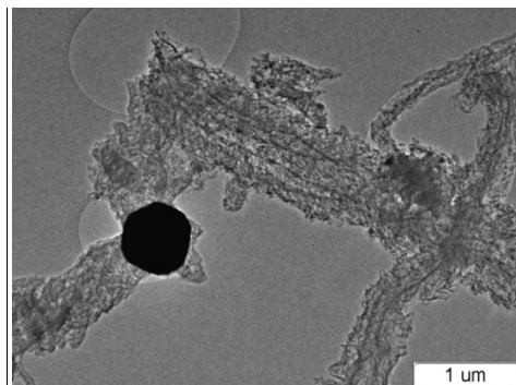
Рис. 1. Снимок ПЭМ. Активный центр роста УНВ, сформировавшийся из никель-медного сплава при контакте с 1,2-дихлорэтаном при 600°C.
