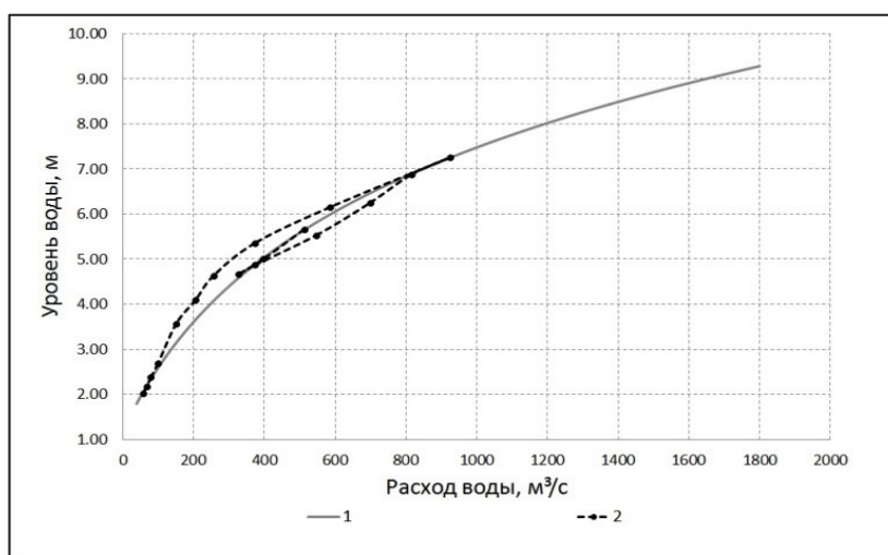
Рис. 1. Петлеобразная зависимость расходов и уровней воды в сравнении с кривой расходов при отсутствии неустановившегося режима в створе ГП р. Урал – г. Оренбург
