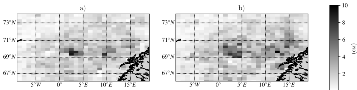
Рис. 2. Средняя амплитуда (в ячейке 1^{\circ} долготы, 0.3^{\circ} широты) вихрей, идентифицированных методом автоматической идентификации в Норвежском море за 1993-2017 гг. а) циклонических, б) антициклонических.
