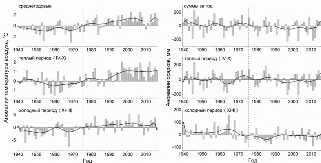
Рис. 1. Годовые и сезонные аномалии средней температуры воздуха и суммарных осадков относительно климатической нормы 1961-1990 гг., сглаженные 11-летним скользящим средним
