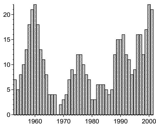
Рис. 1. Летние потепления в морской Арктике: число выходов суммы T > 0 за 95% уровень, осредненное в 5-летних интервалах
