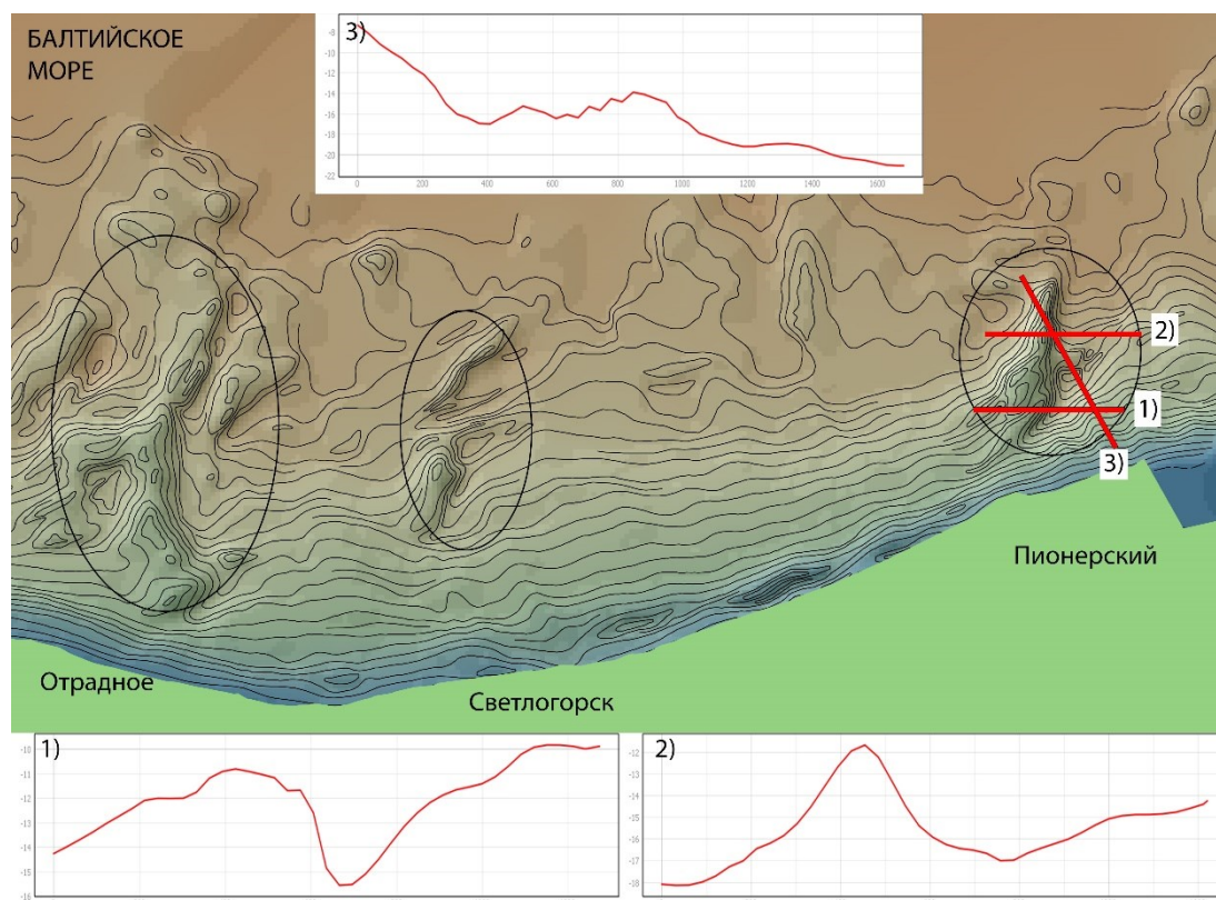
Рис. 2. Особенности донной топографии в районе Светлогорской бухты.
