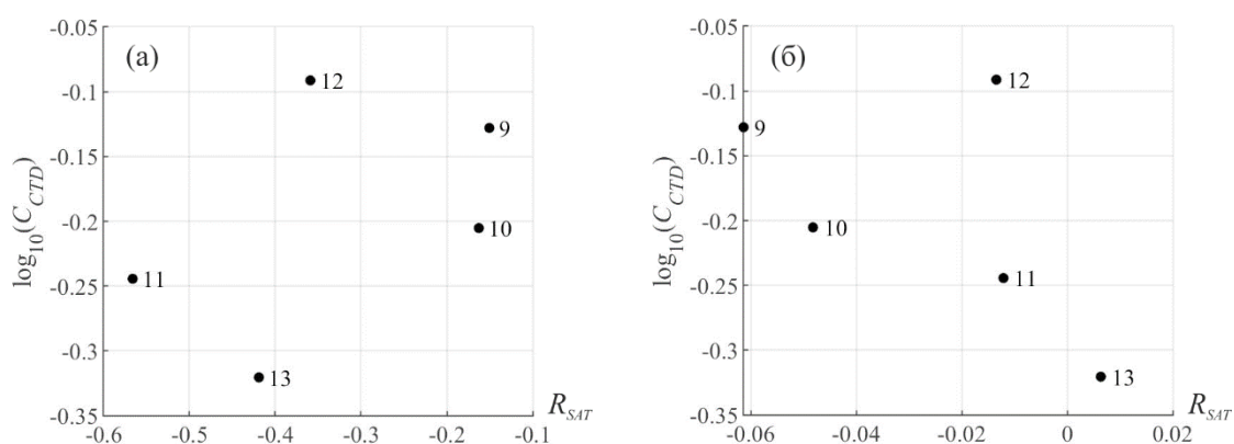
Рис. 4. Диаграмма рассеяния судовых измерений концентрации хл.-а C_{CTD} и спутниковых измерений индексов цвета R_{SAT} , посчитанных с применением алгоритма NIR(а) и MUMM (б). Цифрами около точек отмечены номера станций.
