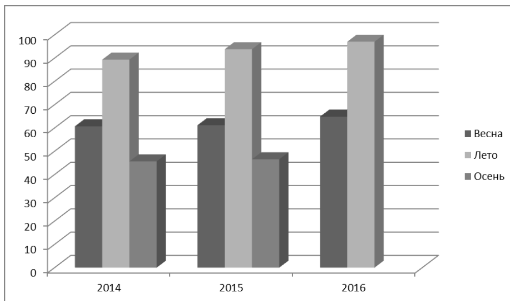
Рис. 1. Сезонная динамика биомассы мезопланктона в Азербайджанской акватории Каспийского моря в 2014-2016 гг. ( \text{мг}/\text{м}^3 ).
