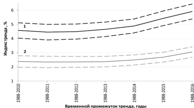
Рис. 1. Межгодовая изменчивость индексов тренда влагосодержания атмосферы (1) и температуры воздуха (2) над Мировым океаном с 1988–2010 гг. по 1988–2016 гг. Пунктирными линиями отмечены стандартные ошибки оценки тренда.
