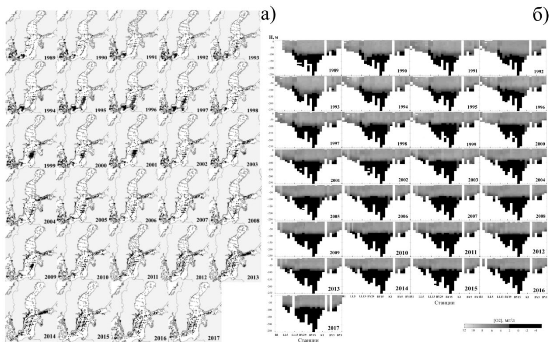
Рис. 1. Океанологические станции, где отмечались гипоксические условия ( O_2 < 2 мл/л, черные кружки), и где значения O_2 \geq 2 мл/л (серые кружки) – а. Вертикальное распределение содержания растворенного кислорода в водах Балтийского моря на разрезе океанологических станций – б
