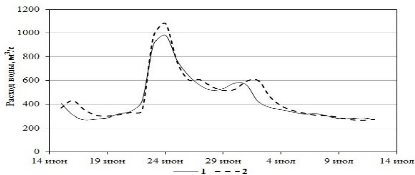
Рис. 3. Фактический (1) и прогнозный (2) гидрографы июньского паводка 2002 г. в створе р. Лаба – х. Догужиев
