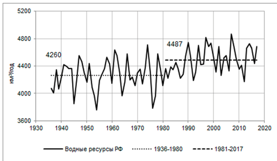
Рис. 1. Многолетняя динамика водных ресурсов Российской Федерации
