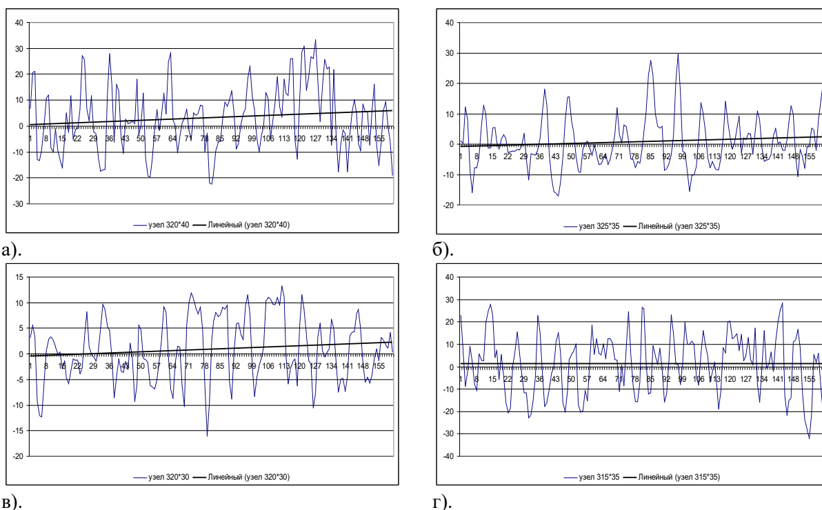
Рис. 2 (а-г). Временной ход уровня и его линейный тренд в точках с координатами (320*40 ( а), 325*35 (б), 320*30 (в), 315*35 (г)).
