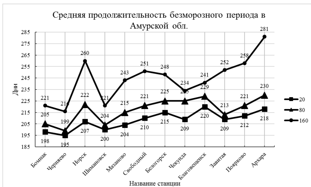
Рис. 3. Средняя продолжительность безморозного периода в Амурской области, дни (на оси абсцисс станции расположены с севера на юг).
