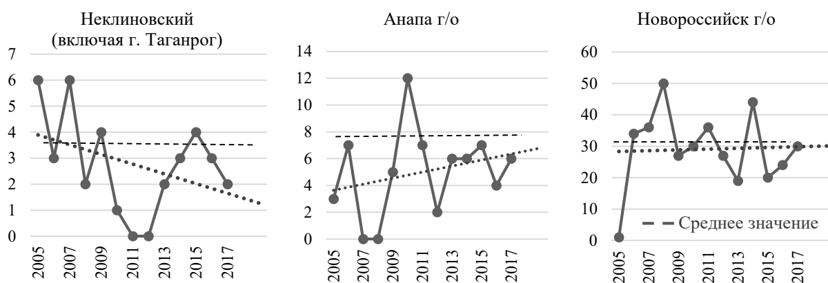
Рис. 4. Динамика возникновения сильного ветра >15\text{ м/с} с 2005 по 2017 гг. в указанных районах (кол-во дней в год)
