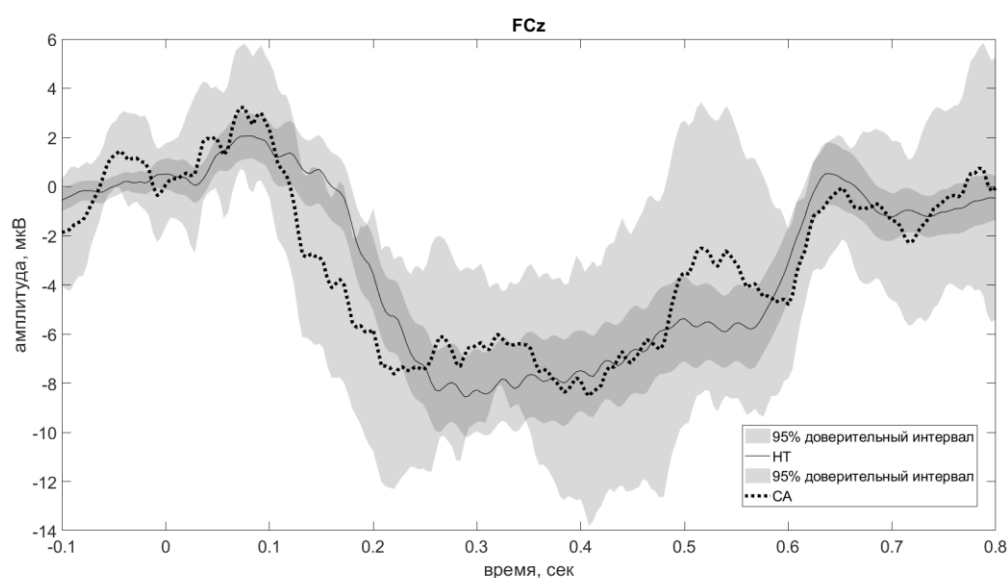
Рис 2. Устойчивая волна в ответ на предъявление последовательностей щелчков с частотой 40 Гц. Пунктиром изображен ответ испытуемых с синдромом Ангельмана (n=8), линией — контрольной группы (n=31). Светло-серая область обозначает 95% доверительный интервал.
