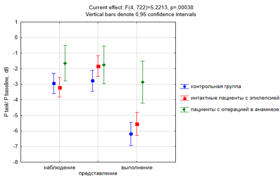
Рисунок 1. Относительные значения мощности компонент мю-ритма в контрольной группе и двух подгруппах пациентов с эпилепсией (прошедших операцию и без операции); Значения мощности спектра во время фоновой пробы (открытые глаза) равны 0.
