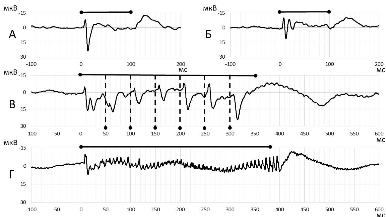
Рис 1. Вызванные потенциалы с глубинного электрода, записанные в ответ на простые тоны (А-600 Гц, Б – 4000 Гц), составной тон (В) и лексический стимул (Г – гласная “О”). Отрезки над графиками обозначают длительность звучания
