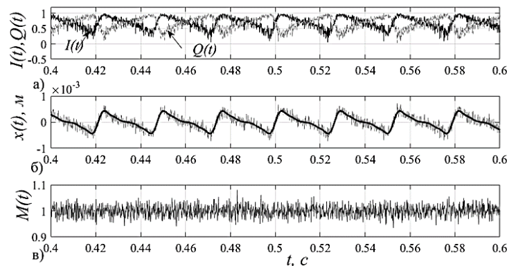
Рисунок 2. Временные диаграммы работы СВЧ датчика вибрации - а) сигналы I(t) и Q(t) ; б) сигнал вибрации (перемещение) x(t) ; в) модуль аналитического сигнала M(t) .
