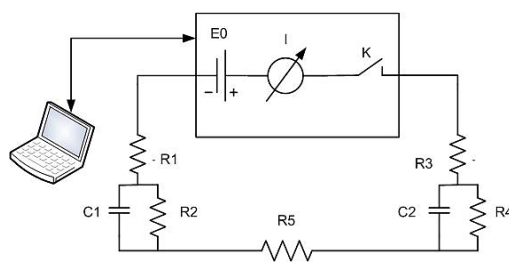
Рисунок 2. Эквивалентная схема измерения на физической модели с графитовыми электродами.
