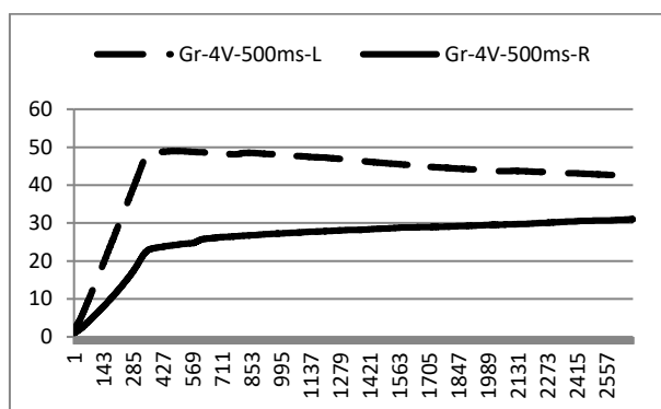
Рисунок 7. Сравнение динамики тока при измерениях на симметричных участках кожи (точки TR4) слева и справа при использовании графитовых электродов. Испытуемый А., измерительное напряжение 4 В.
