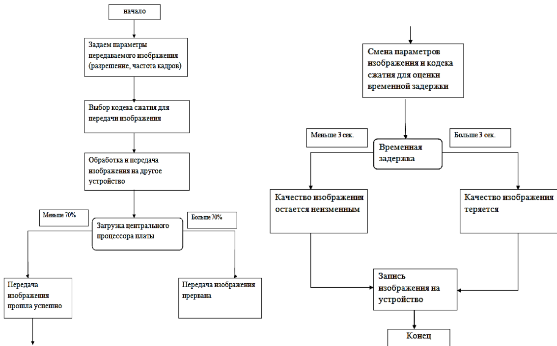
Рисунок 2. Блок-схема алгоритма передачи изображения
