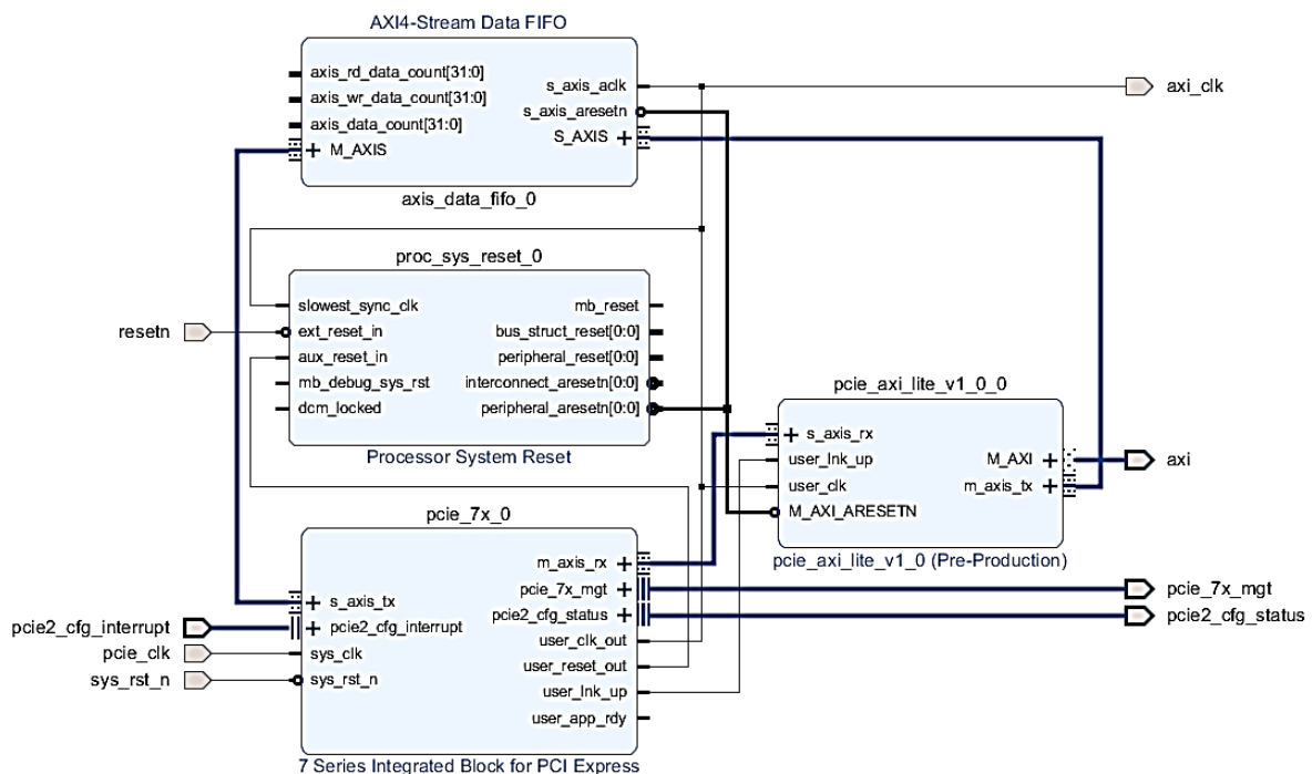
Рисунок 2 – Структурная схема модифицированного адаптера AXI Stream-AXI4 Lite
