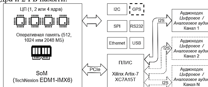
Рисунок 1 – Структурная схема устройства
