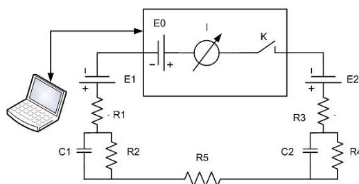
Рисунок 1. Эквивалентная схема измерения на физической модели со стальными электродами.
