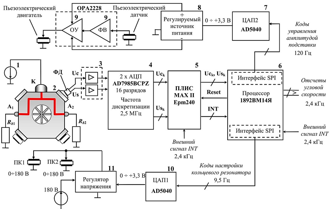
Рисунок 1. Структурная схема блока электроники ЦЛГ. 1 – источник высокого напряжения, 2 – кольцевой гелий-неоновый лазер, 3 – блок усилителей первичных сигналов, 4 – аналого-цифровой преобразователь, 5 – ПЛИС, 6 – процессор 1892ВМ14Я, 7, 11 – цифро-аналоговые преобразователи, 8 – источник питания, 9 – петля обратной связи электромеханического автогенератора частотной подставки (ФВ – фазовращатель, ОУ – операционный усилитель), 11 – регулятор напряжения на пьезопреобразователях ПК, перемещающих зеркала кольцевого резонатора
