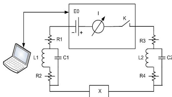
Рисунок 4. Эквивалентная схема измерения на коже человека с графитовыми электродами.
