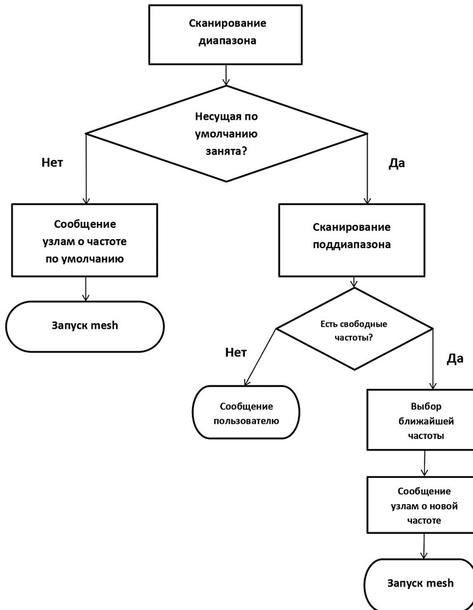
Рисунок 2. Блок-схема алгоритма выбора несущей частоты
