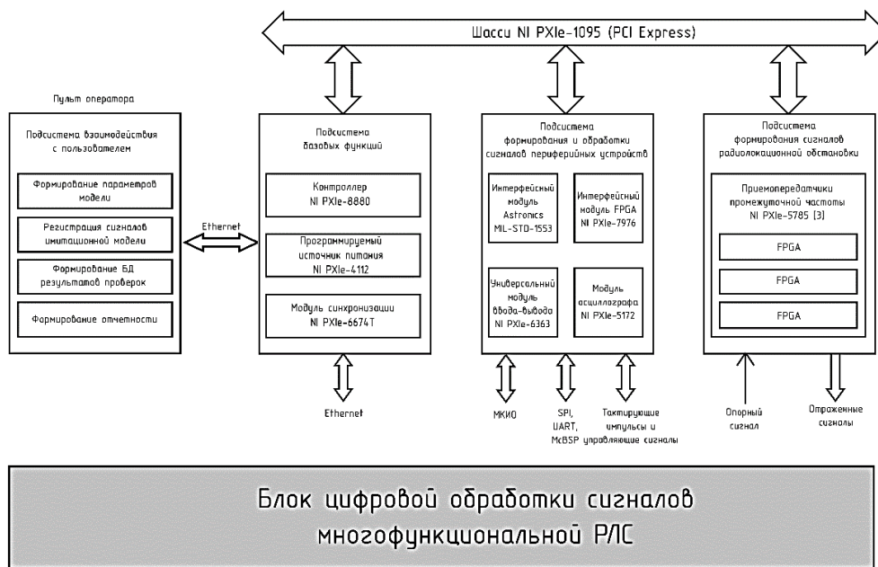
Рисунок 2 — Структурная схема комплекса
