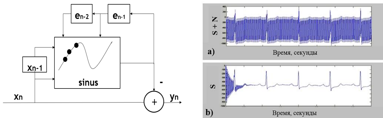
Рисунок 1 – Блок-схема адаптивного режекторного фильтра 50 Гц (слева). Здесь x_t – входной сигнал, y_t – выходной сигнал, n – индекс времени, e_n – текущая невязка между реальной помехой и ее моделью в форме синусоиды 50 Гц. Пример подавления сетевой помехи (справа). S – полезный сигнал, N – шум.
