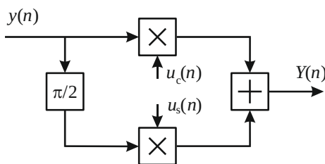
Рисунок 1. Структурная схема синхронного квадратурного амплитудного детектора
