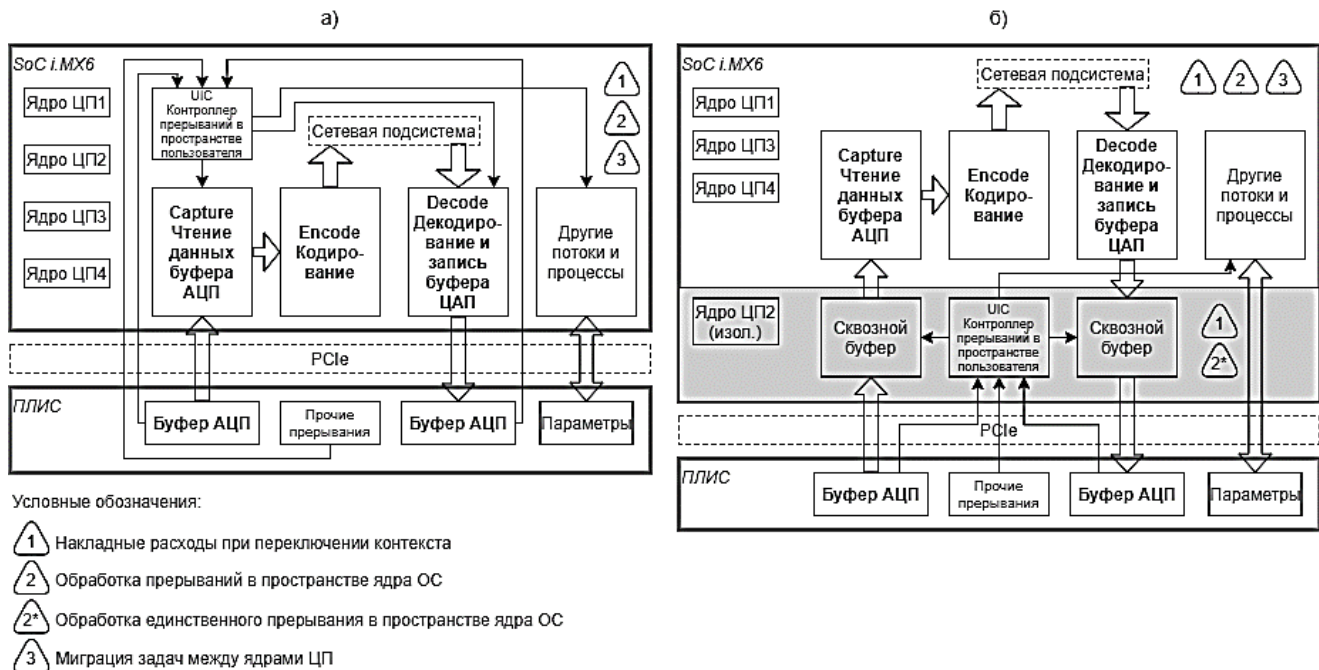
Рисунок 4 – Обработка аудиобуферов в приложении: а) до оптимизации; б) после оптимизации
