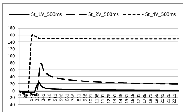
Рисунок 6. Динамика тока при измерении проводимости модели стальными электродами при напряжениях 1 В, 2 В и 4 В.
