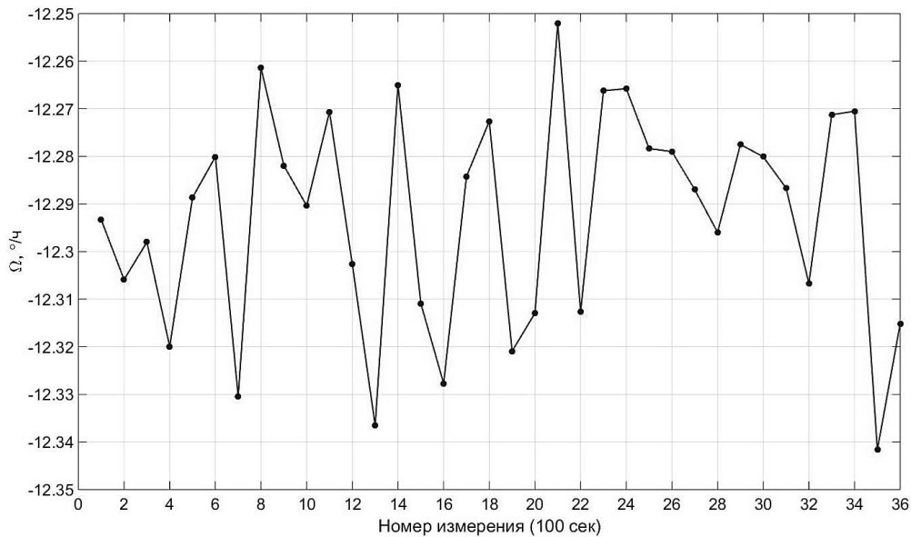
Рисунок 3 – Средние значения угловой скорости при 100 секундном усреднении. Среднее значение угловой скорости 12,29 °/ч, среднеквадратическое отклонение 0,023 °/час
