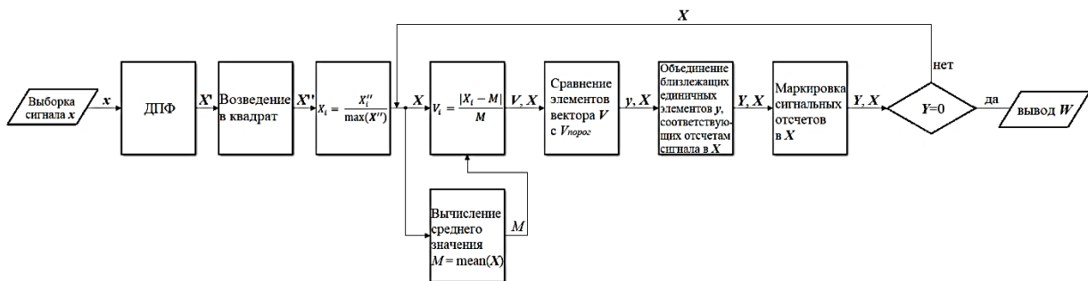
Рисунок 1 – Структурная схема разработанного алгоритма обнаружения
