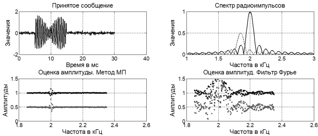
Рисунок 1. Сравнение оценок амплитуды при фильтрации фильтром Фурье и фильтром максимального правдоподобия. Разность фаз случайна. Отношение сигнал/шум = 20 дБ.
