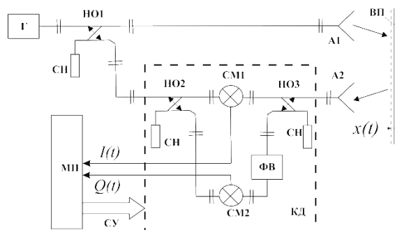
Рисунок 1. Структурная схема СВЧ датчика для измерения параметров вибрации.
