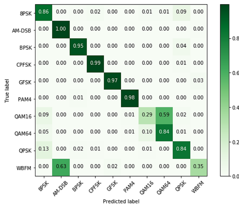
Рисунок. 4. Матрица ошибок для сигналов с ОСШ 0 дБ
