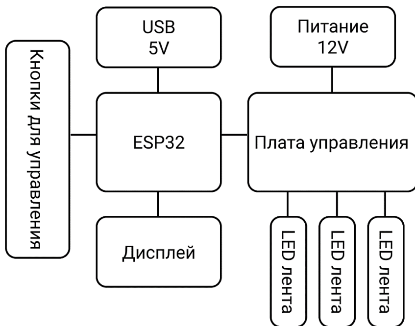
Рисунок 2 – Блок- схема устройства
