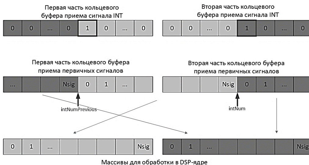
Рисунок 2 — Схема приёма первичных сигналов и обработки управляющего сигнала INT
