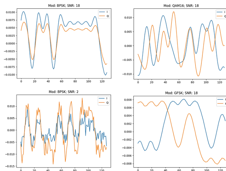
Рисунок 1. Примеры визуализации данных из набора для различных видов модуляции и ОСШ
