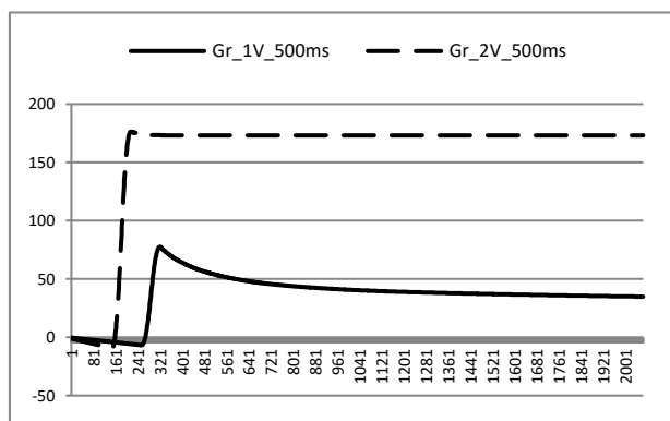
Рисунок 5. Динамика тока при измерении проводимости модели графитовыми электродами при напряжениях 1 В и 2 В.
