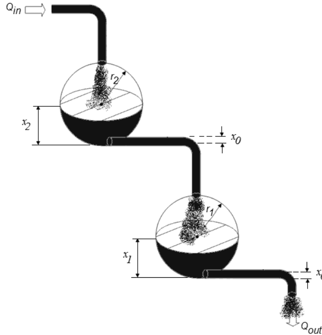
Рисунок 1. Схематическая модель двух связанных сферических резервуаров
