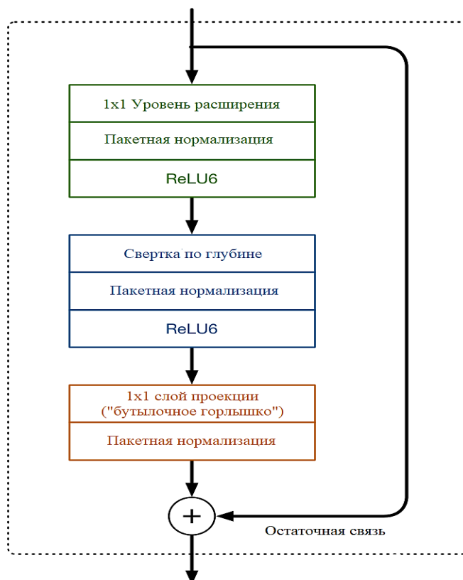
Рис. 2. Структурная схема основного составного блока CHC MobileNet SSDv2
