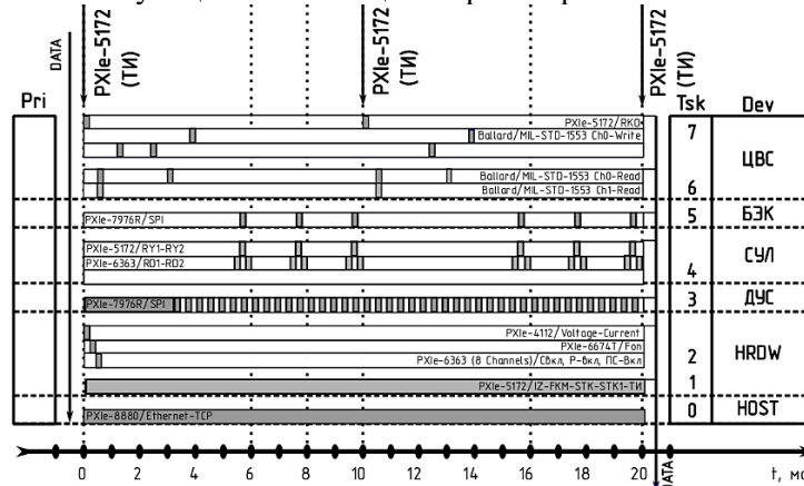
Рисунок 3 — Схема планирования процессорного времени системы реального времени
