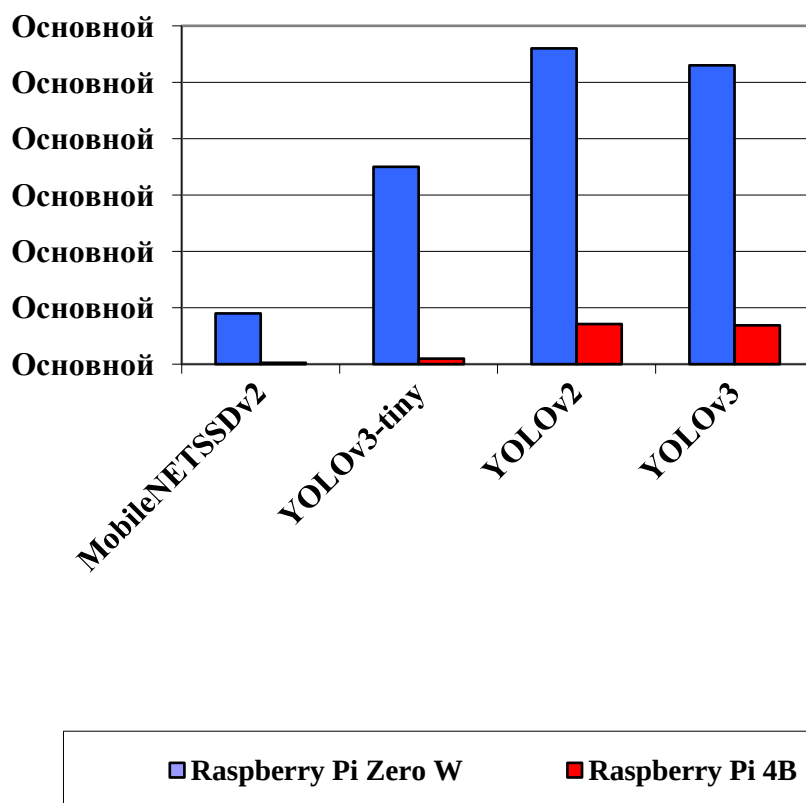
Рис. 3. Диаграмма зависимости времени обработки одного изображения от используемой СНС и модели микрокомпьютера
