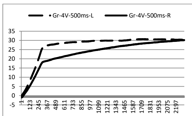
Рисунок 9. Сравнение динамики тока при измерениях на симметричных участках кожи (точки С7) слева и справа при использовании графитовых электродов. Испытуемый Б., измерительное напряжение 4 В.
