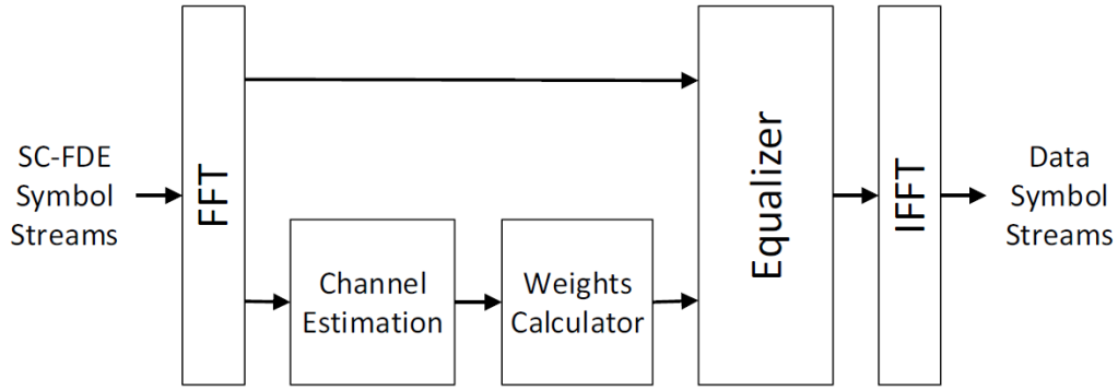
Рисунок 1. Схема обработки сигнала в SC-FDE приёмнике
