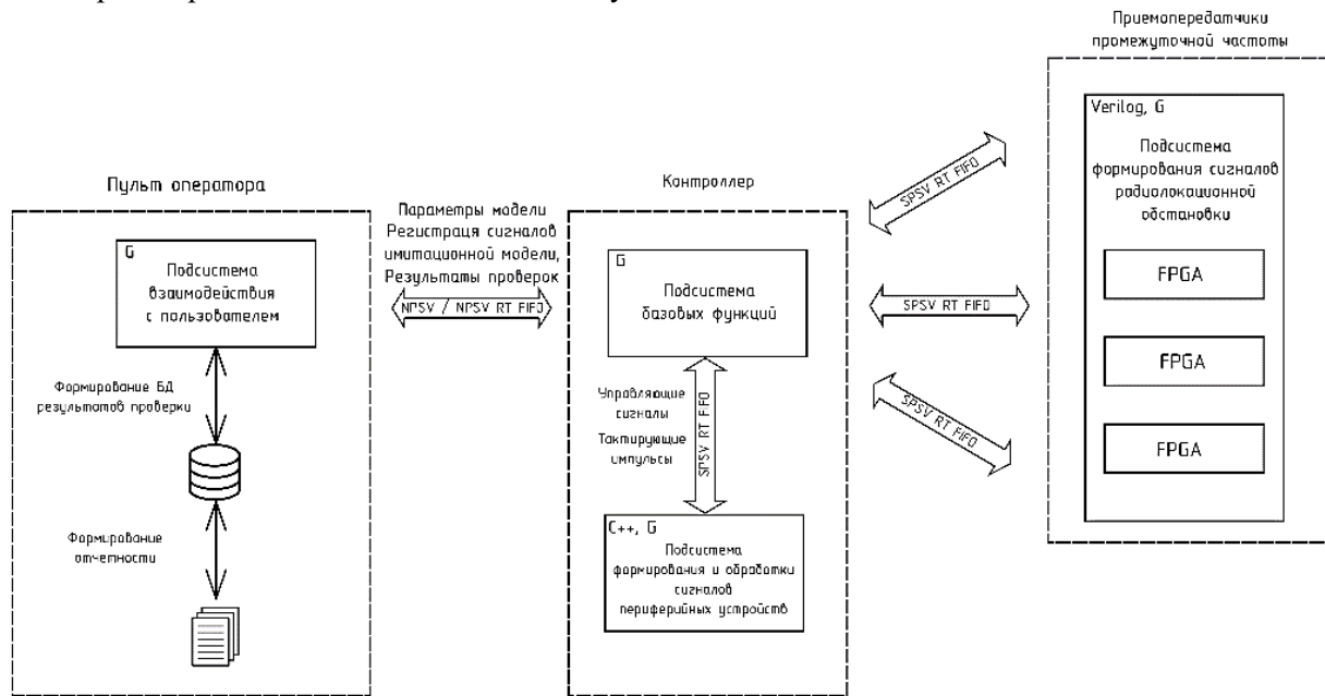
Рисунок 4 — Структурная схема программного обеспечения комплекса
