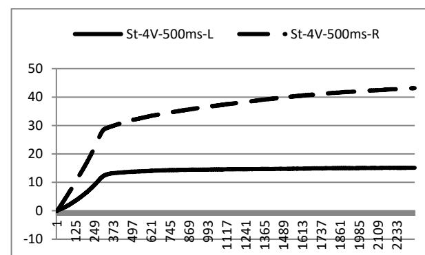
Рисунок 10. Сравнение динамики тока при измерениях на симметричных участках кожи (точки С7) слева и справа при использовании стальных электродов. Испытуемый Б., измерительное напряжение 4 В.
