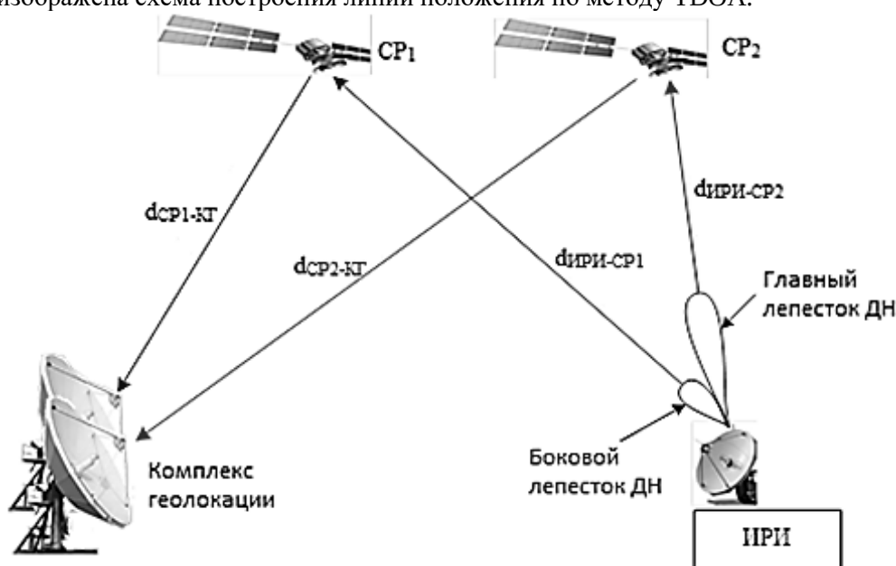
Рисунок 1. Схема построения линии положения по методу TDOA
