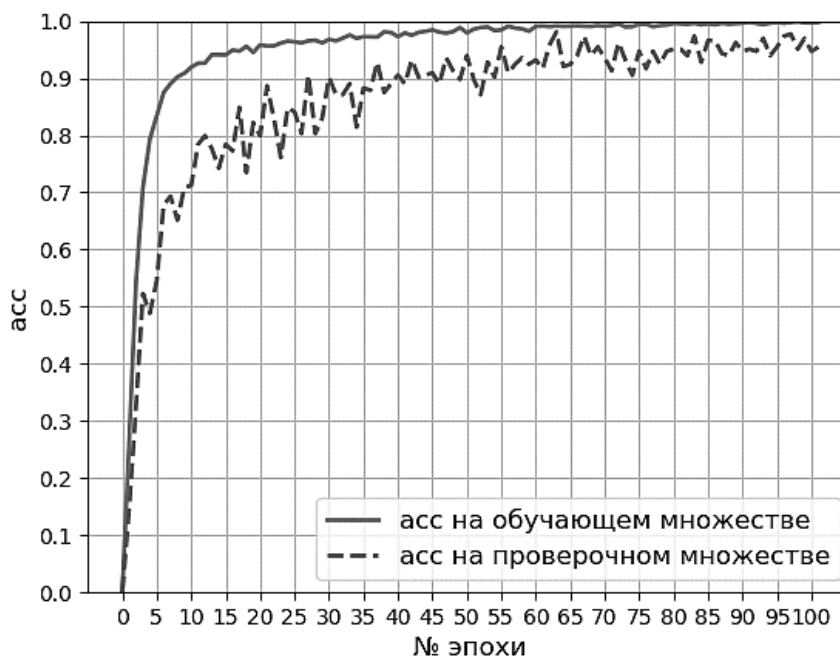
Рисунок 3. Кривые изменения доли правильных ответов в процессе обучения CNN-VGGMulti
