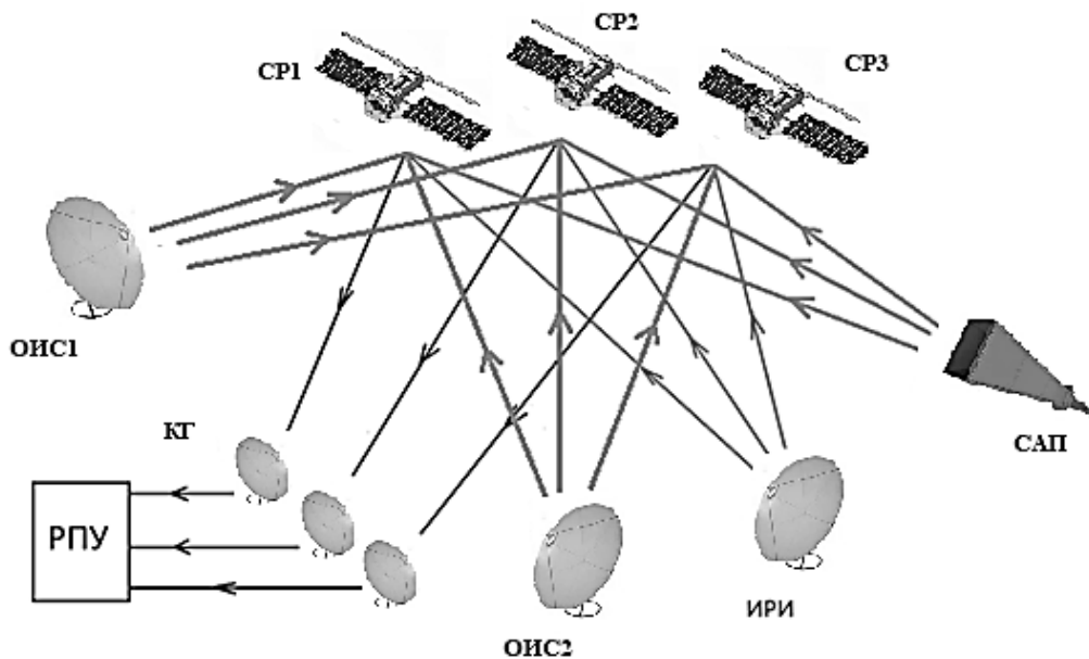
Рисунок 2. Схема системы геолокации, работающей по предложенному методу
