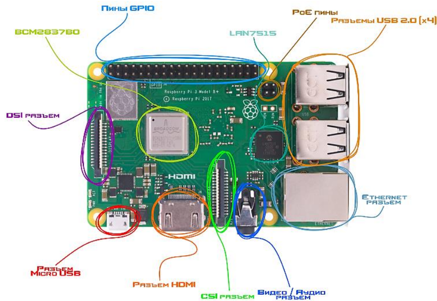
Рисунок 1. Одноплатный микрокомпьютер Raspberry Pi 3 Model B+
