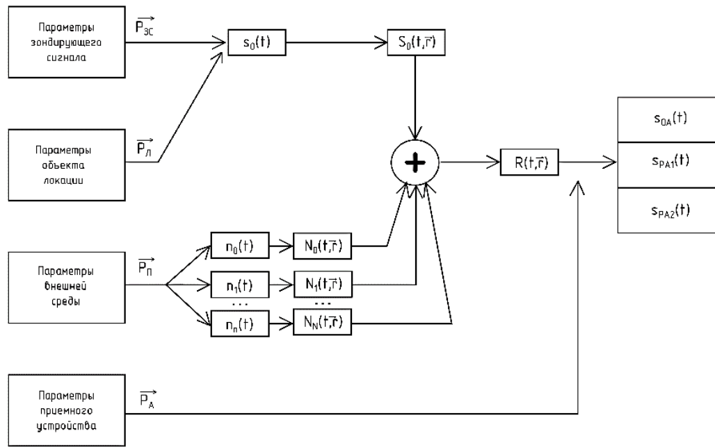
Рисунок 1 — Обобщенная модель РЛС
