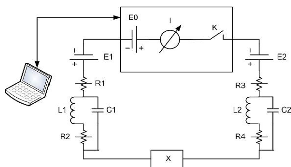
Рисунок 3. Эквивалентная схема измерения на коже человека со стальными электродами.
