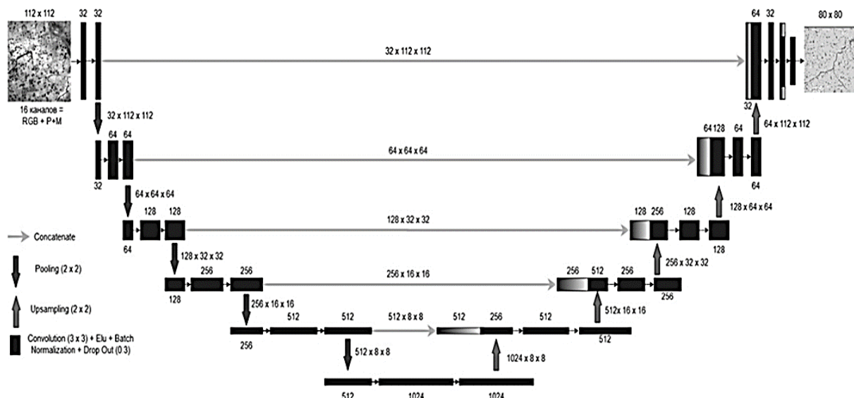
Рисунок 1 – Структура модифицированной СНС
