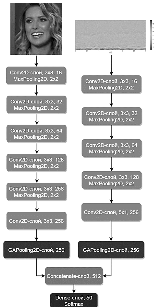
Рисунок 2. Архитектура сверточной нейронной сети CNN-VGGMulti
