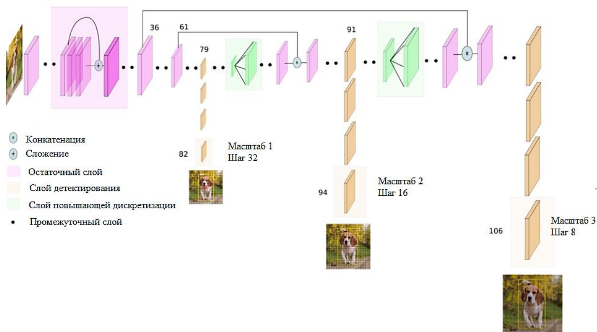
Рис. 1. Структурная схема сверточной нейронной сети YOLOv3
