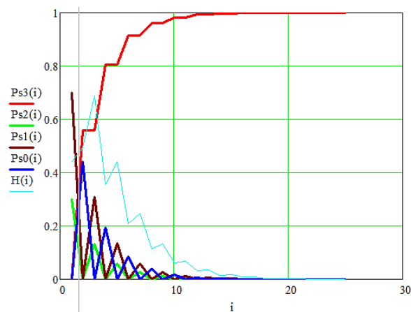
Рисунок 3 - Графики вероятностей нахождения цепи в своих состояниях и энтропии системы от шагов процесса
