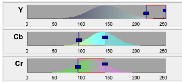
Рисунок 2 – Гистограммы YCbCr
