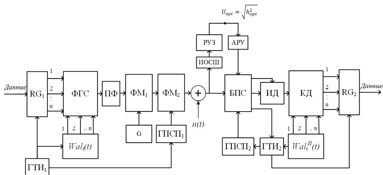
Рисунок 1 – Структурная схема релейского радиоканала связи с кодовым уплотнением данных
