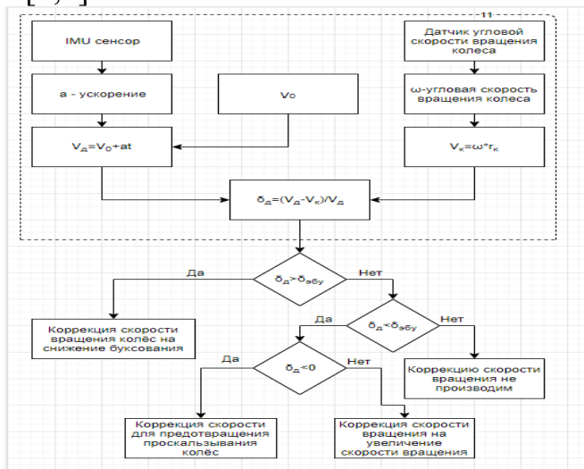
Рис. 1. Блок схема системы управления активным приводом колёс
