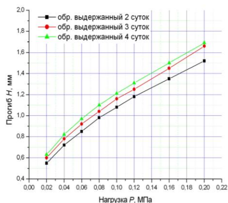
Рис.2 – Зависимость «Р-Н»
