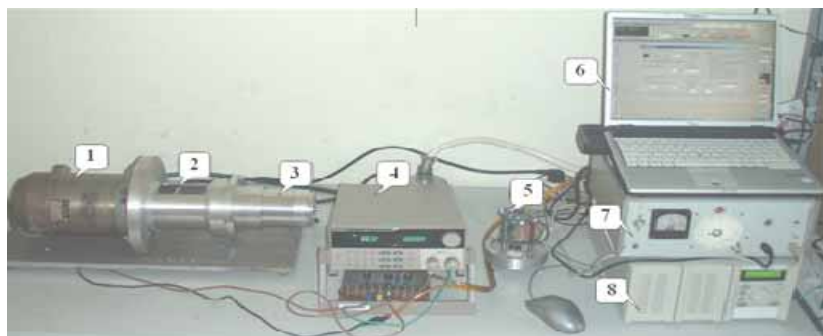
1 – нагрузочный генератор; 2 – согласующая муфта; 3 – вентильный электродвигатель в герметичном контейнере; 4 – электронная нагрузка генератора; 5 – блок управления электродвигателем; 6 – управляющий компьютер; 7 – блок электроники стенда; 8 – блок питания.
