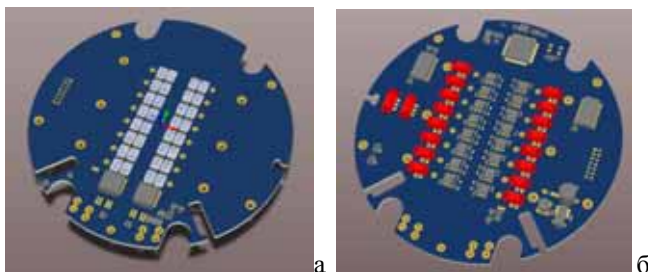
Рис. 2. Вид плат управления аккумуляторной батареей
