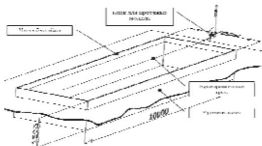
Рис. 1. Схема малого опытового бассейна гравитационного типа
