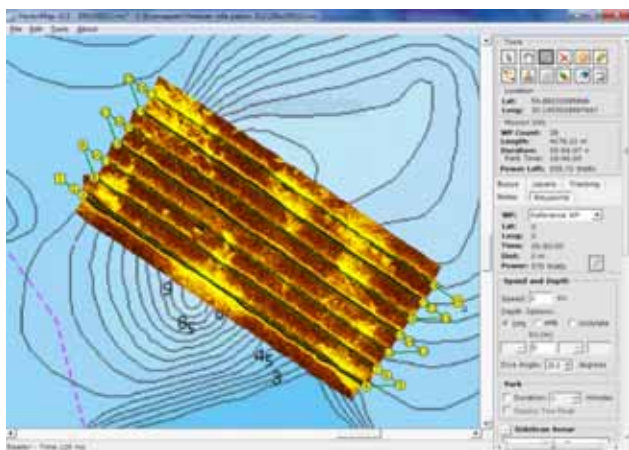
Рис. 4. Измерения ГБО в акватории Невской губы
