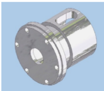
3D модель детали «Корпус гайки поворота»
