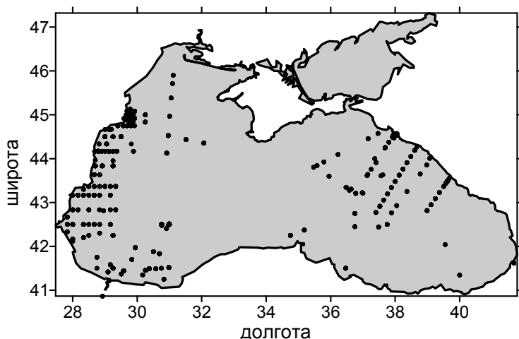
Рис. 1. Расположение по акватории Чёрного моря станций с измерениями нитратов, использовавшимися для валидации результатов моделирования
