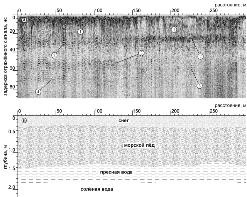
Рис. 3. Временной георадарный разрез по маршруту М-13 1- граница, между снегом и льдом; 2- положение нижней кромки морского льда; 3- предполагаемая граница, между пресной и морской водой; 4- граница неустановленного генезиса
