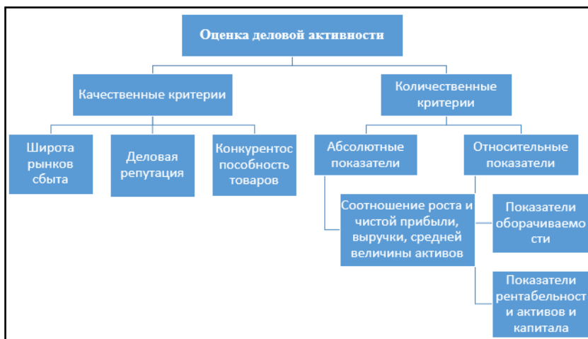
Р и с. 3. Оценка деловой активности
