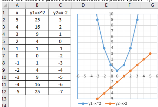
Рис. 4. Решение уравнения x^2 - x + 2 = 0 графическим способом.
