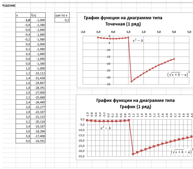
Р и с. 1. Решение системы уравнений, включающее 1 ряд данных
