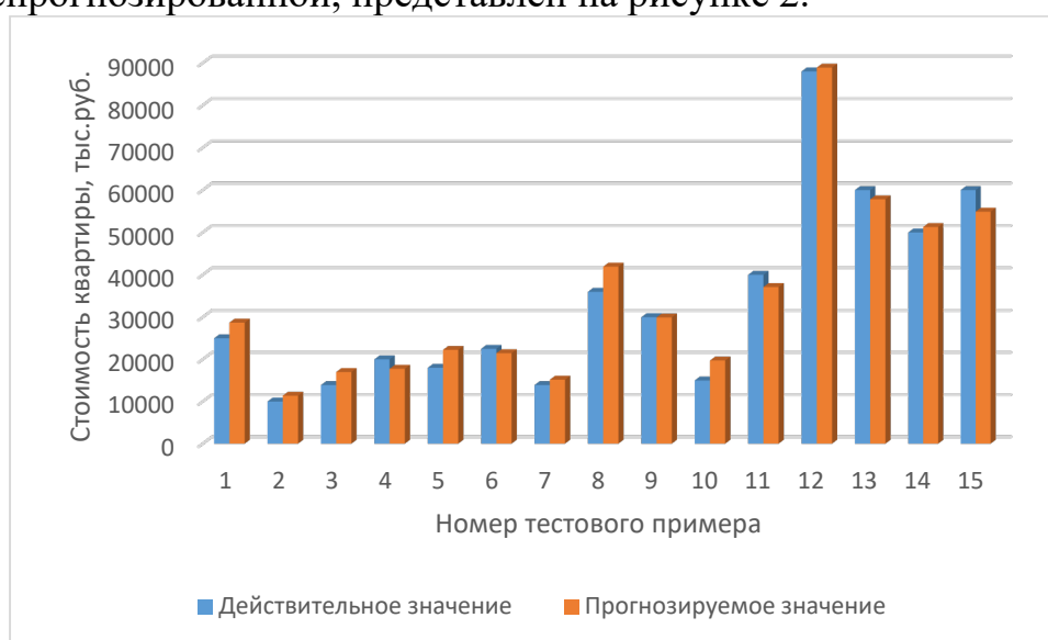
Рисунок 29. Результаты тестирования нейронной сети
