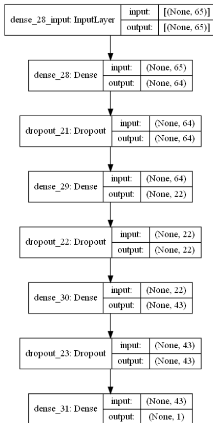
Рисунок 3. Архитектура нейронной сети
