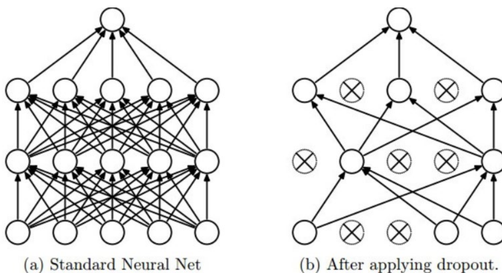
Рисунок 19. Пример работы метода Dropout
