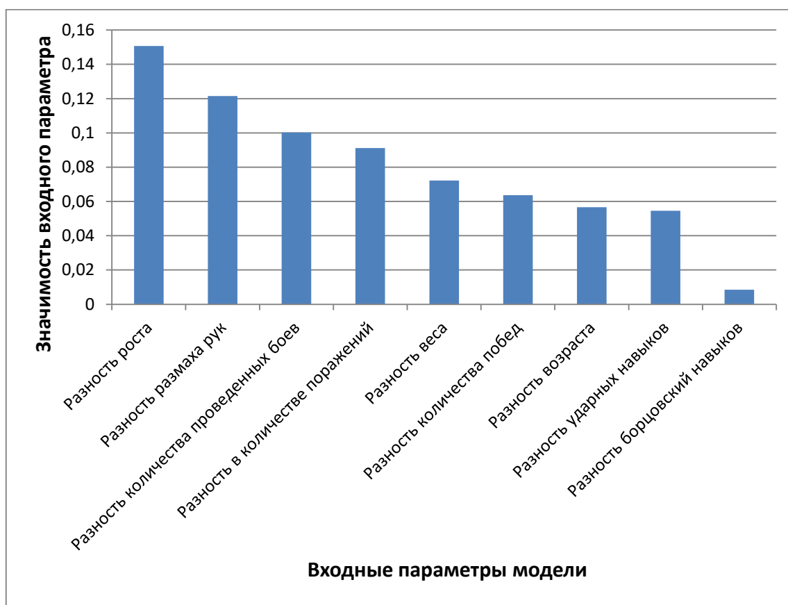
Рисунок 3. Значимость входных параметров нейронной сети
