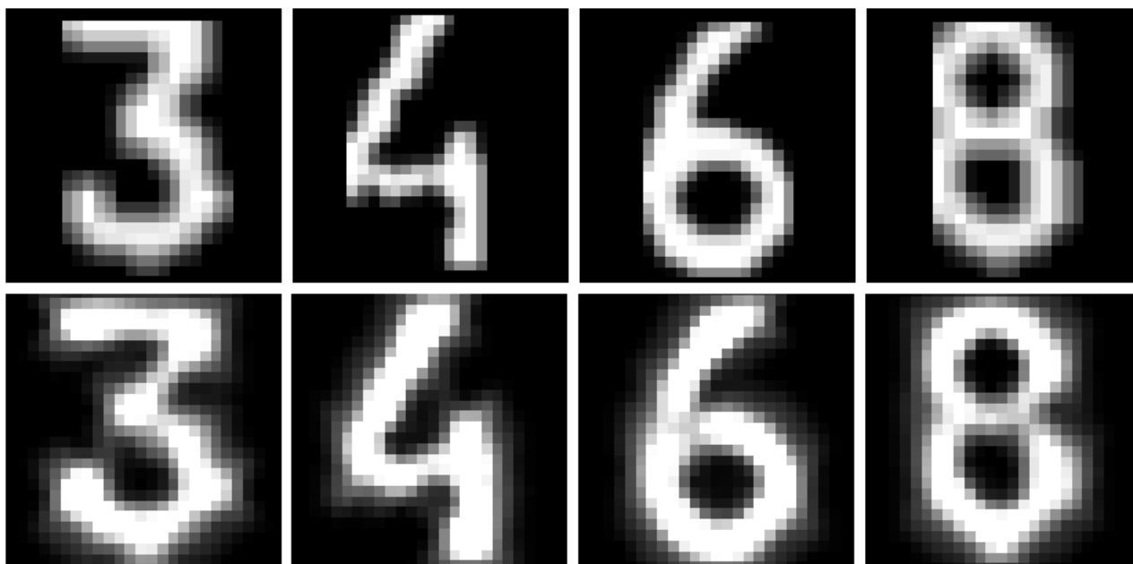
Рисунок 5. Визуализация работы блока выделения линий на основе вероятности активации (вверху – исходное изображение, внизу – активация примитивов линий)
