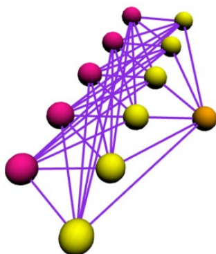
Рисунок 1. Нейронная сеть персептронного типа с пятью входными нейронами, одним скрытым слоем из шести сигмоидных нейронов и одним выходным нейроном
