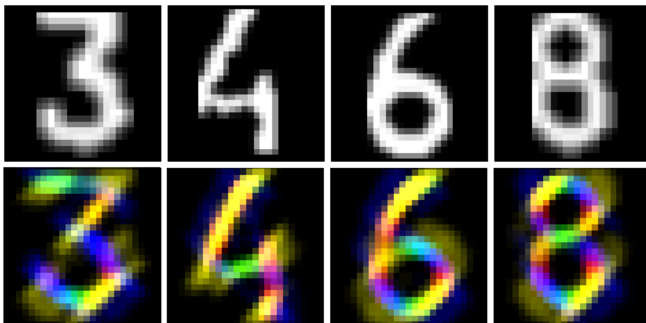
Рисунок 7. Визуализация работы блока выделения линий на основе перцептивно противоположных цветов (вверху – исходное изображение, внизу – активация примитивов линий)
