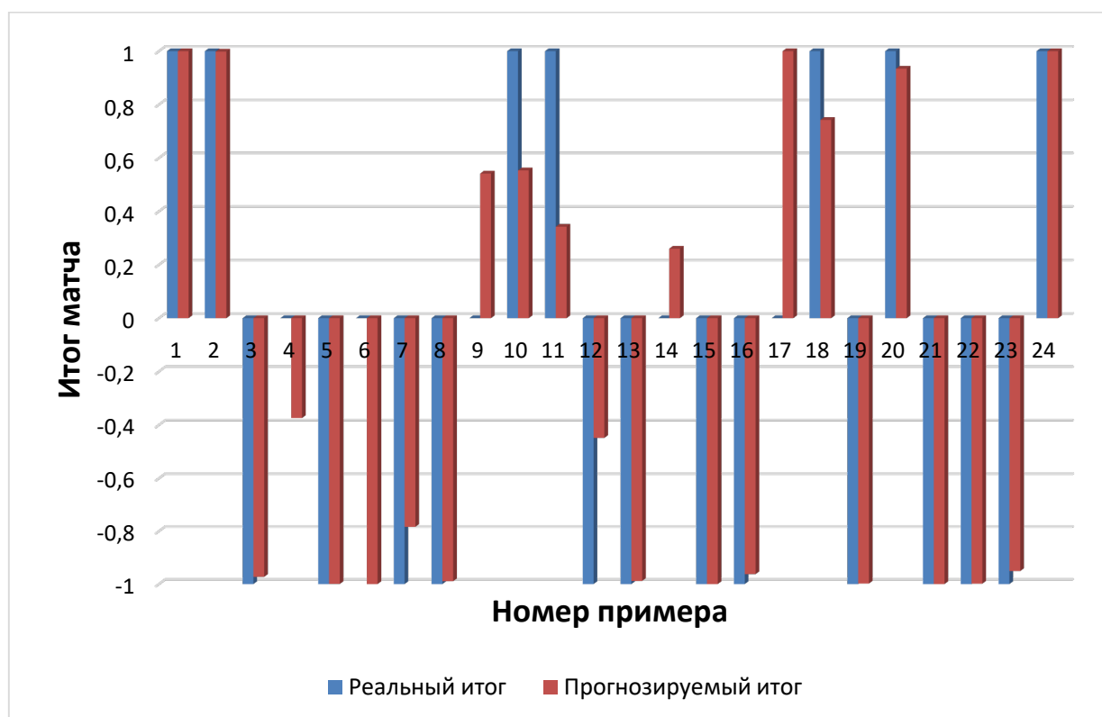
Рисунок 40. Результат тестирования нейронной сети
