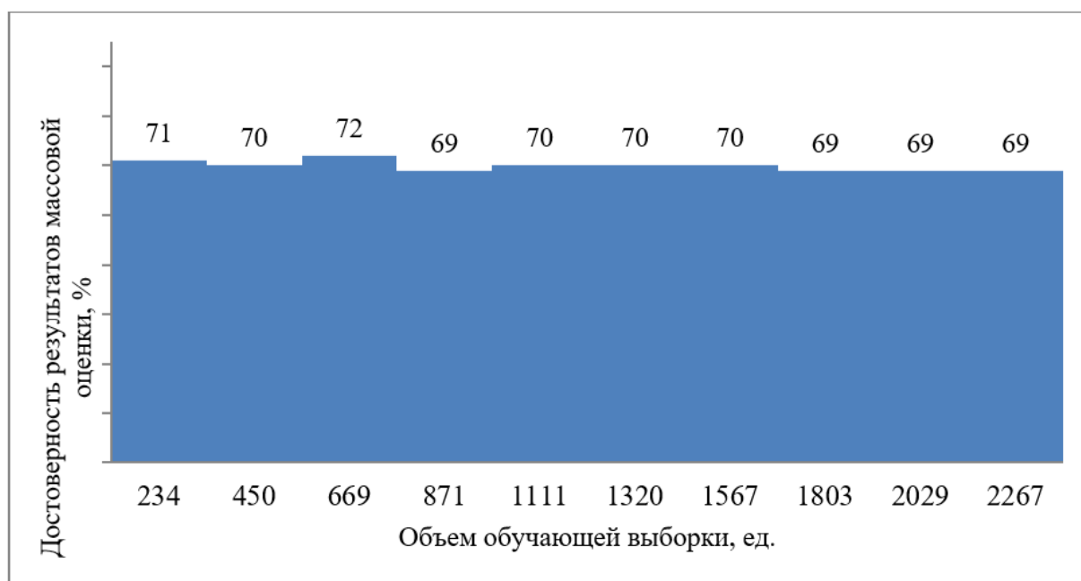
Рисунок 4. Зависимость достоверности массовой оценки от объема обучающей выборки
