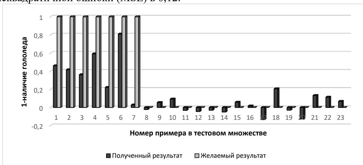
Рисунок 2. Результат тестирования нейронной сети, обученной на примерах 0–12 часов
