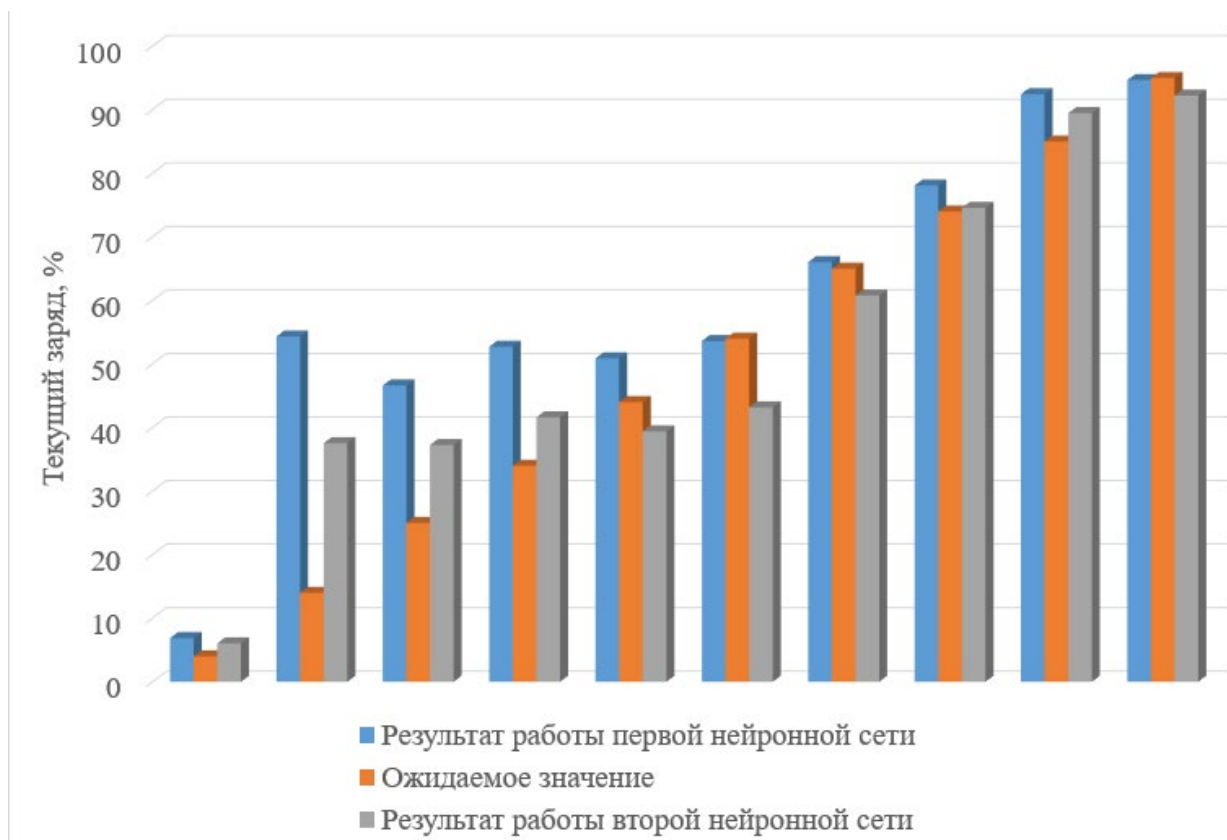
Рисунок 3. Проверка достоверности результатов работы нейронных сетей (процент заряда)
