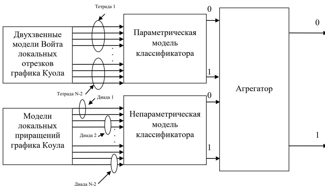
Рисунок 3. Модель гибридного классификатора
