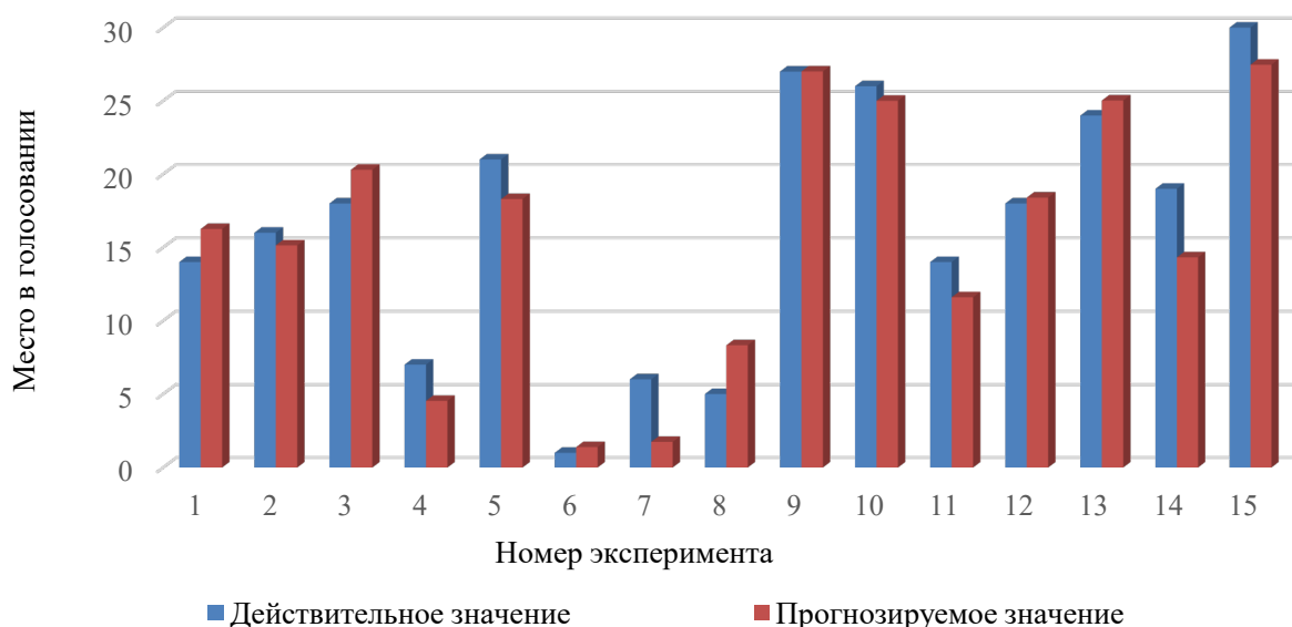
Рисунок 1. Результаты тестирования
