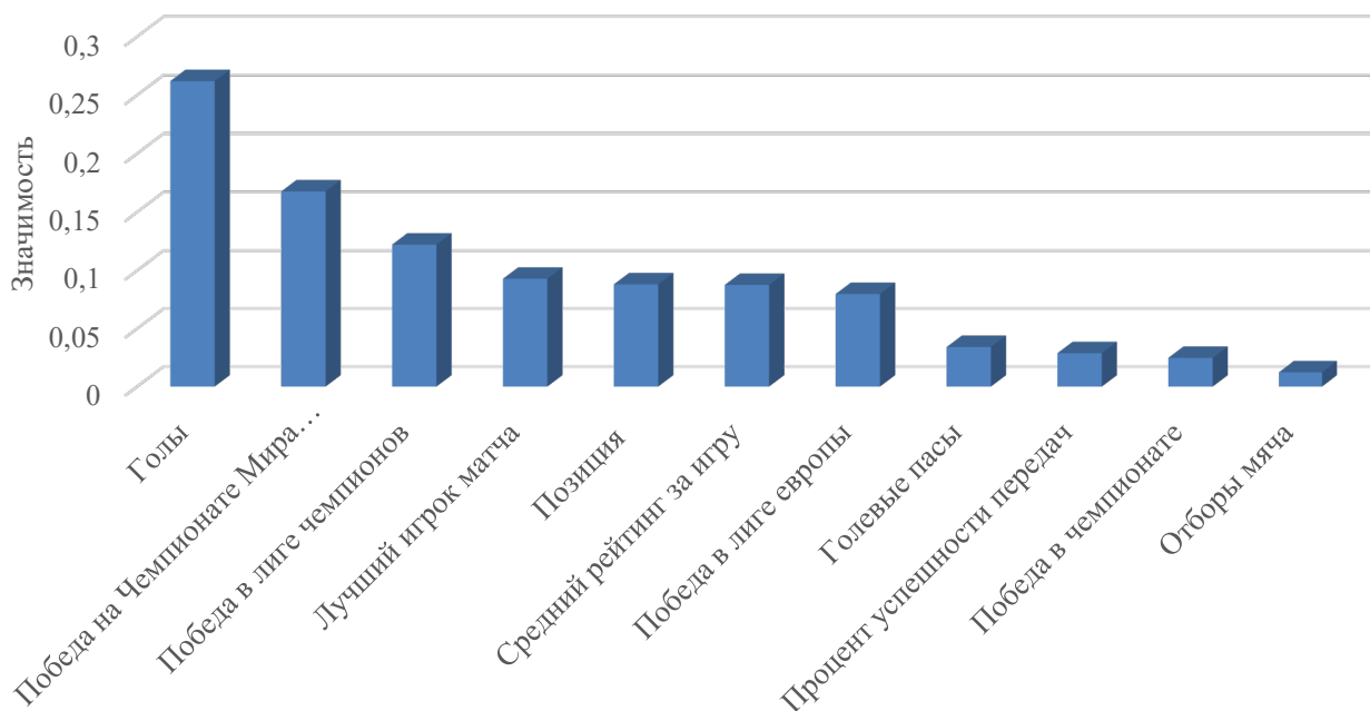
Рисунок 2. Значимость параметров
