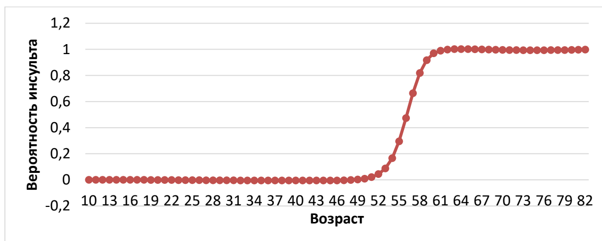
Рисунок 7 – Влияние возраста
