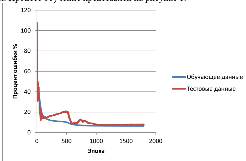
Рисунок 1. Результат обучения нейронной сети.
