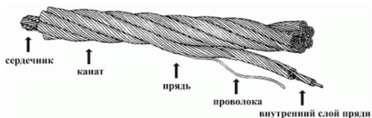
Рисунок 1. Устройство стального троса
