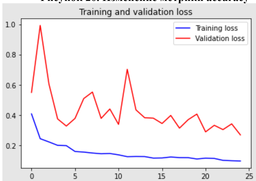
Рисунок 21. Изменение значения функции ошибок
