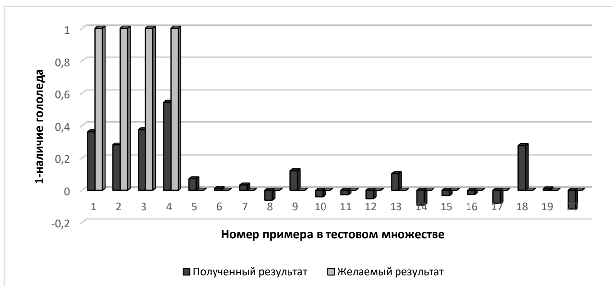
Рисунок 1. Результат тестирования нейронной сети, обученной на примерах 12–0 часов
