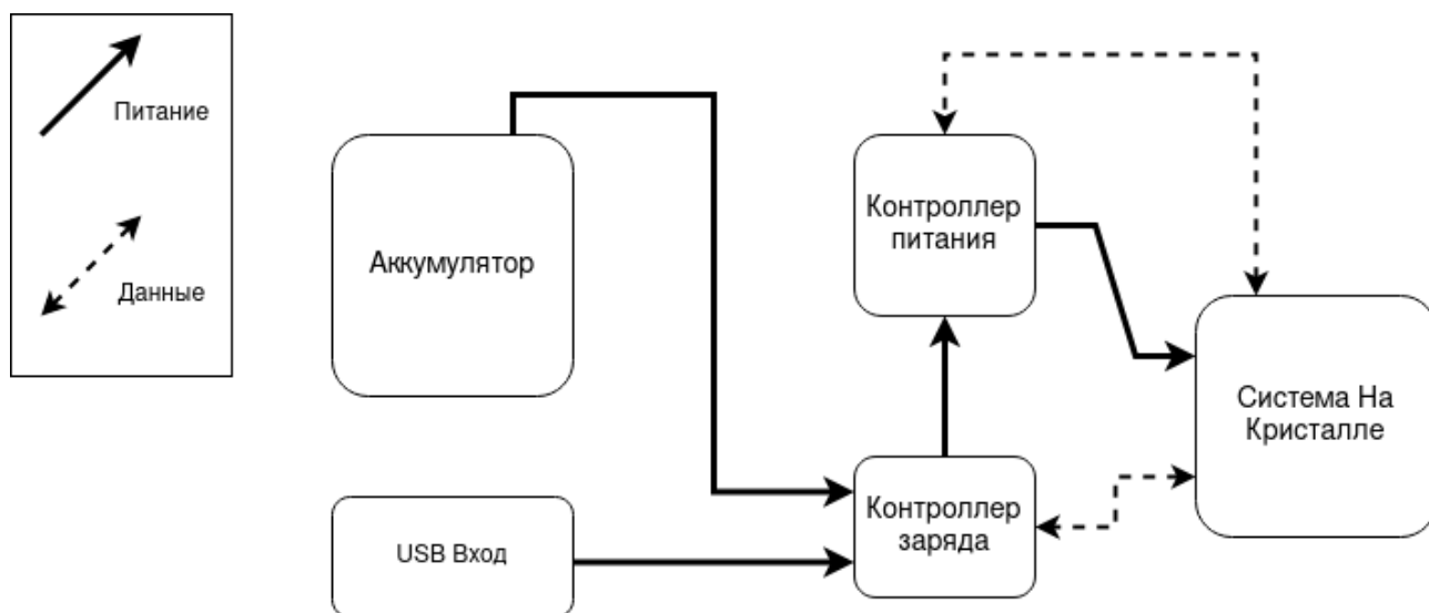
Рисунок 2. Схема питания тестовой системы
