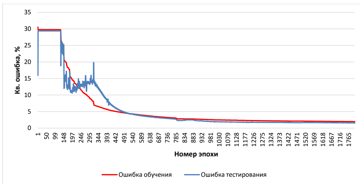
Рисунок 1. График обучения нейронной сети
