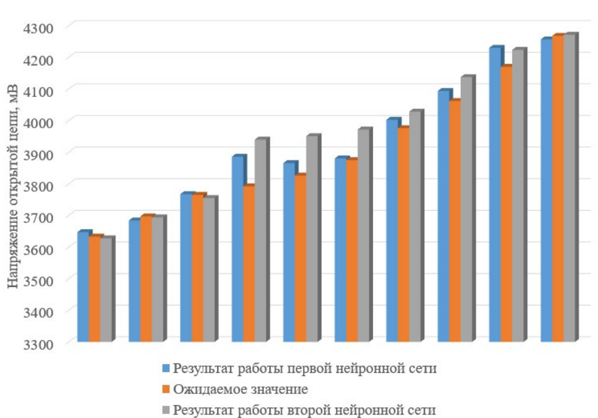
Рисунок 4. Проверка достоверности результатов работы нейронных сетей (напряжение открытой цепи)
