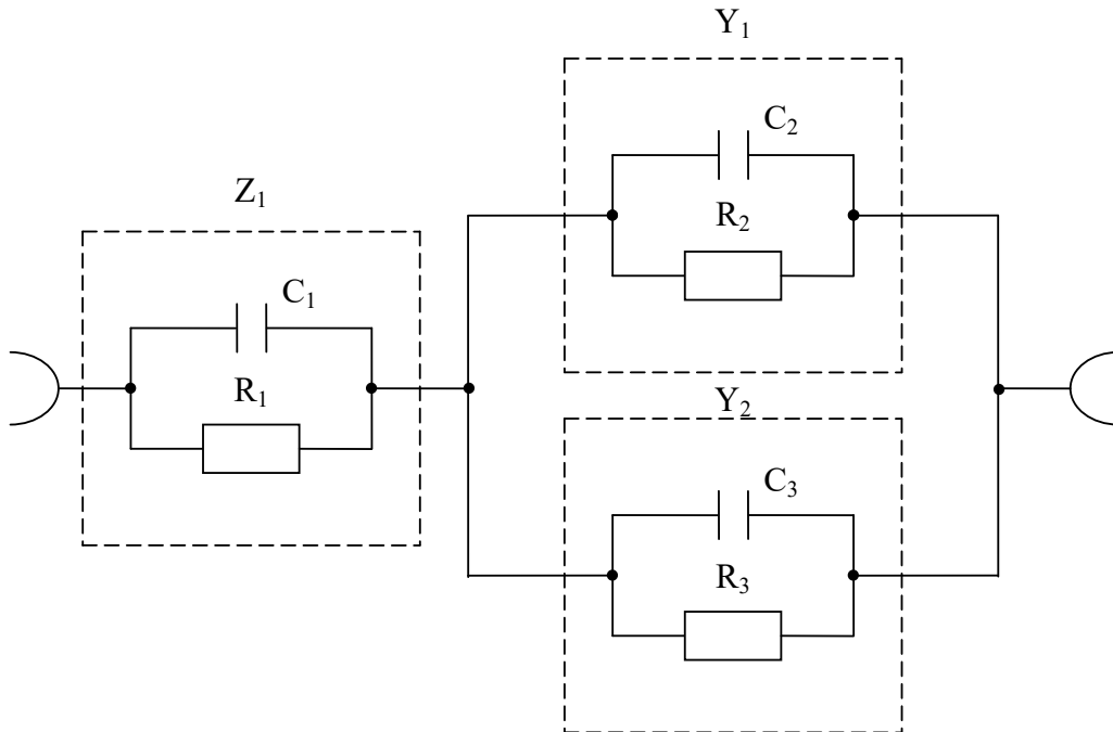
Рисунок 1. Модифицированная модель Войта
