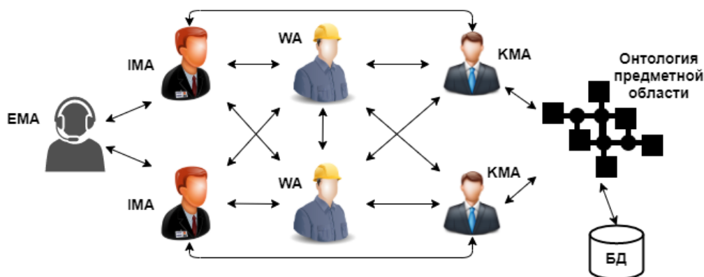
Рис. 1 Схема взаимодействия агентов в системе
