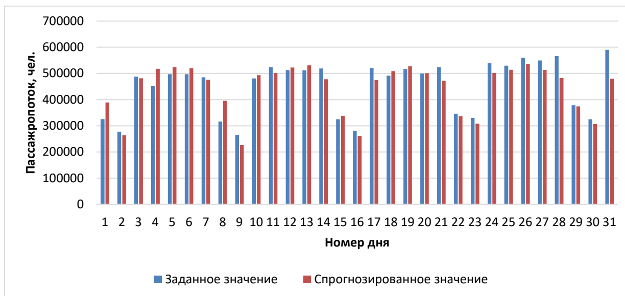
Рисунок 2. Результат тестирования нейронной сети
