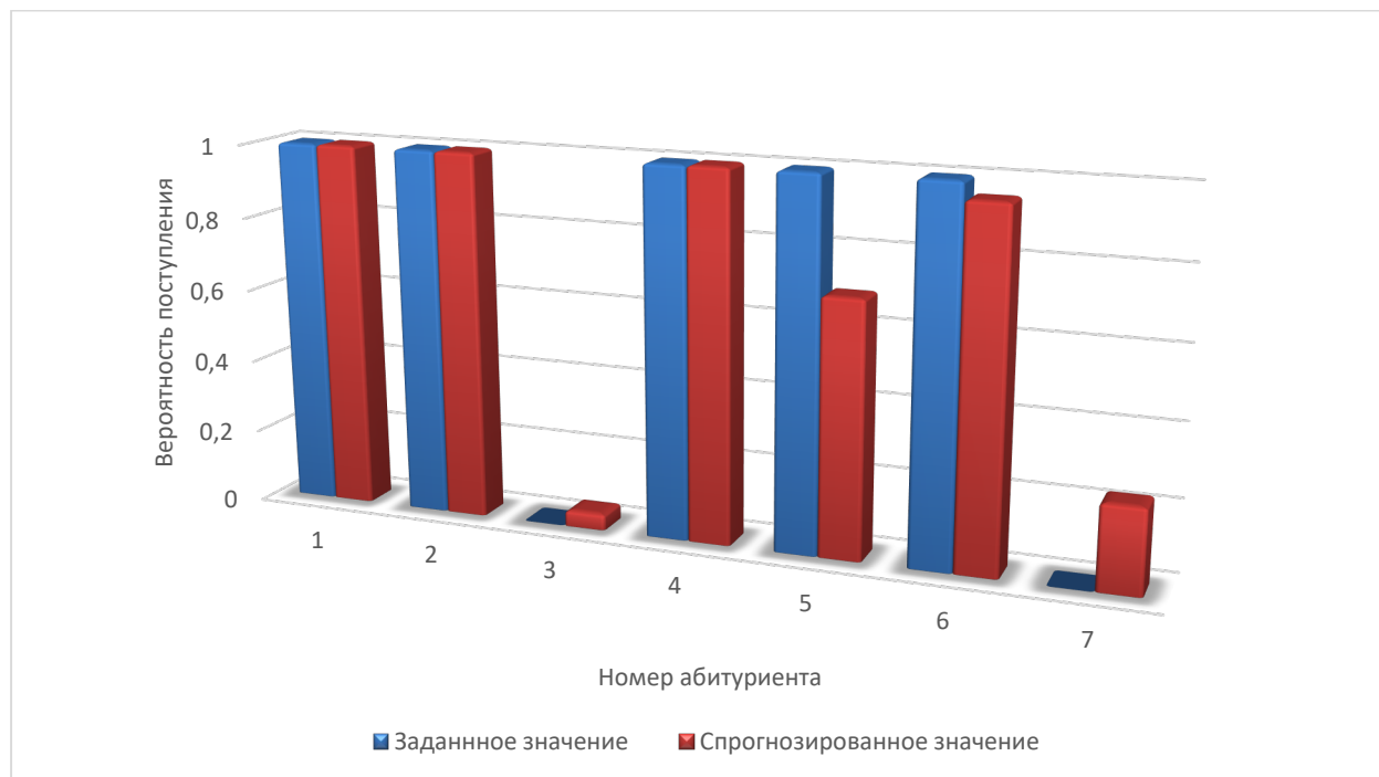
Рисунок 1. Результат тестирования нейронной сети
