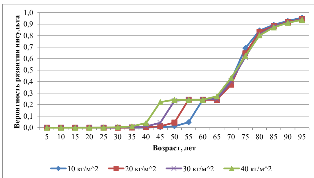
Рисунок 10. Влияния ИМТ
