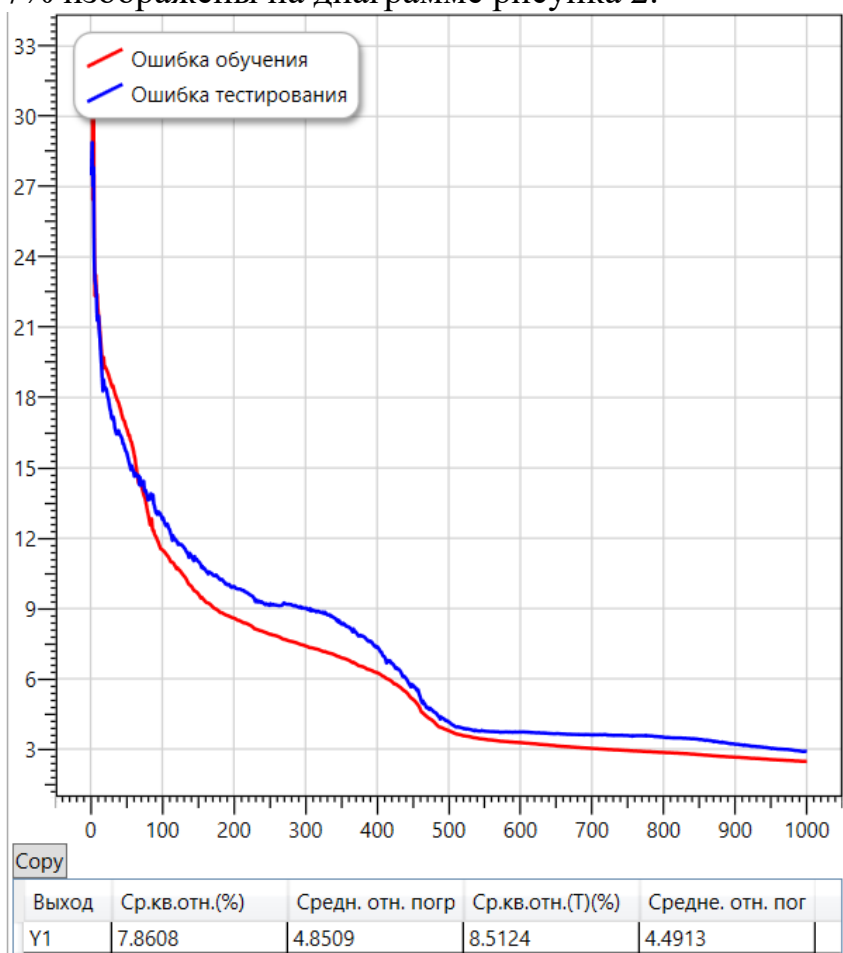
Рисунок 2. Результаты обучения
