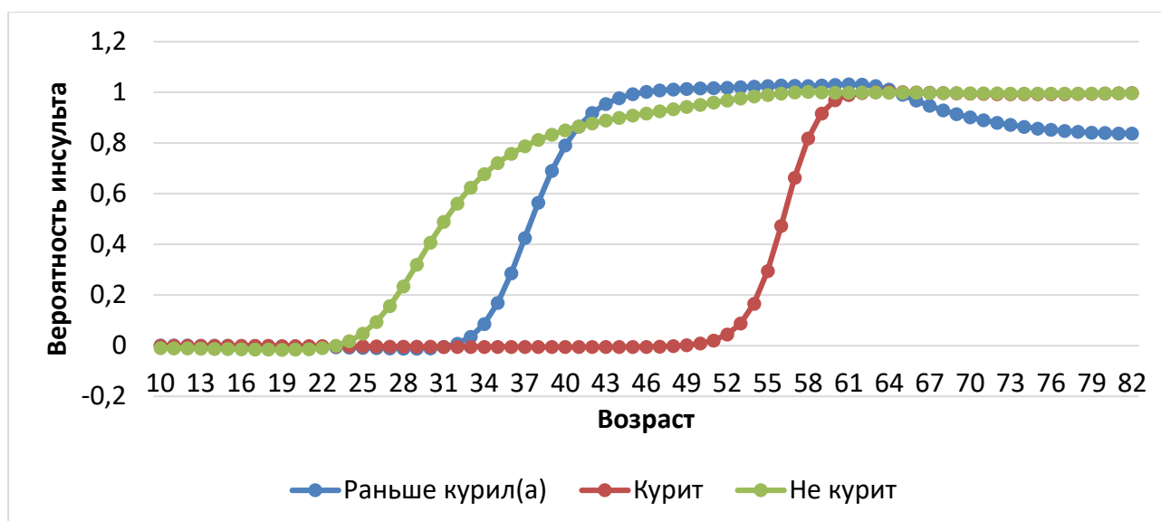
Рисунок 15 – Влияния курения
