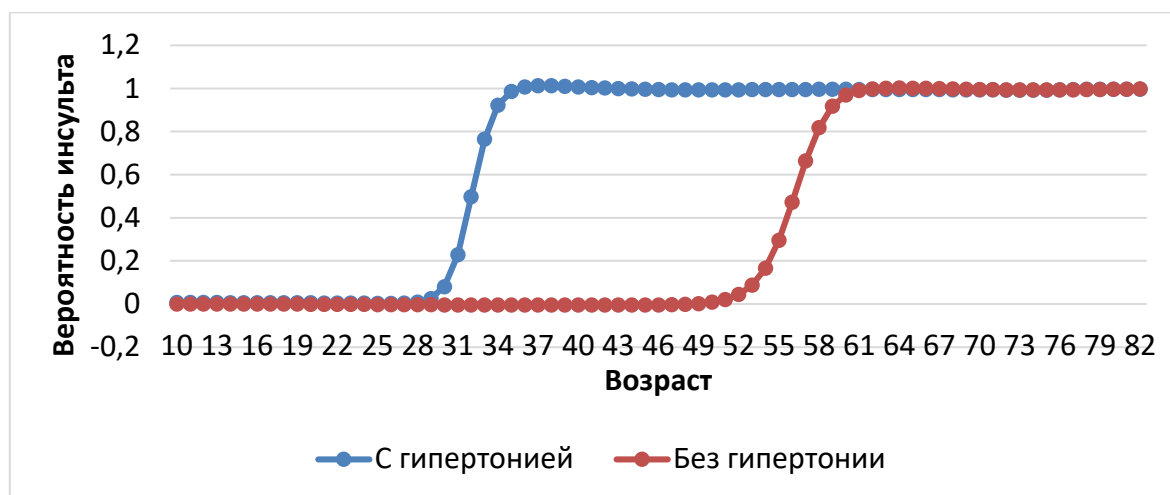
Рисунок 8 – Влияния гипертонии
