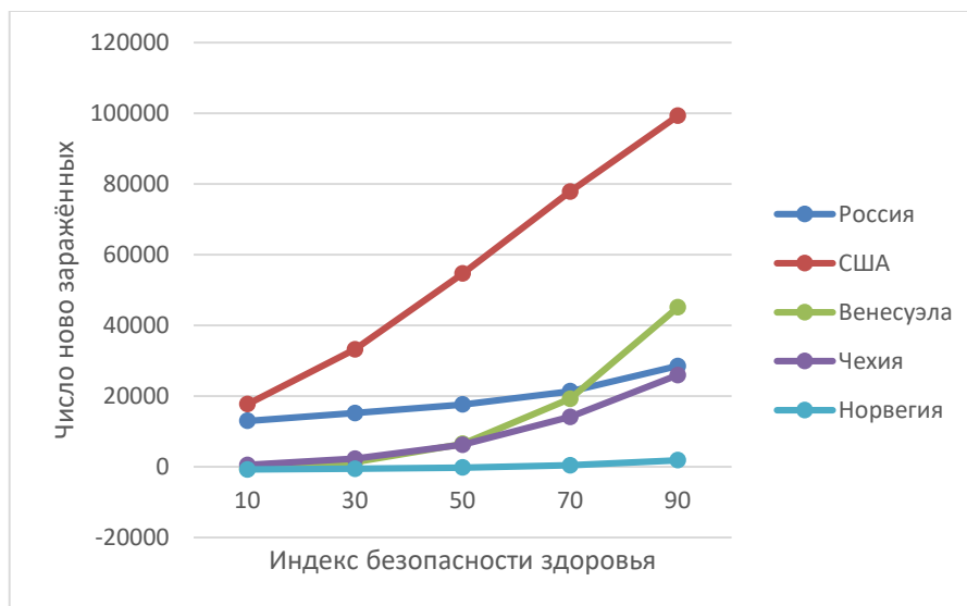
Рисунок 7. Зависимость числа ново заражённых от индекса безопасности здоровья
