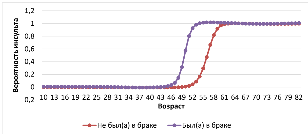
Рисунок 10 – Влияния брака
