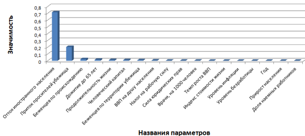
Рисунок 30. Значимость параметров
