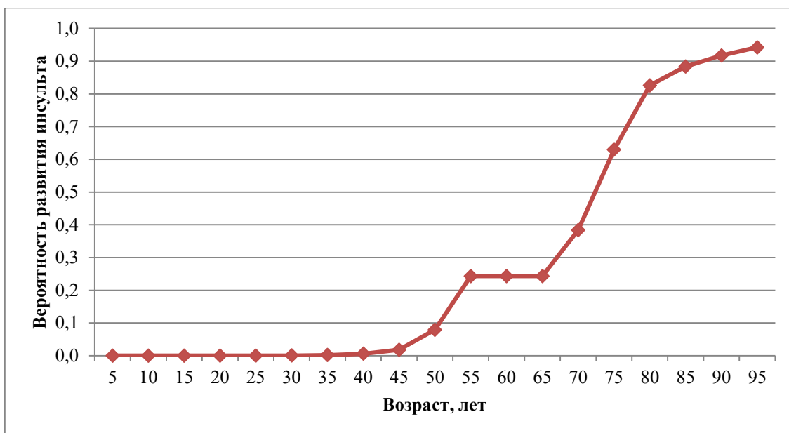
Рисунок 3. Влияние возраста
