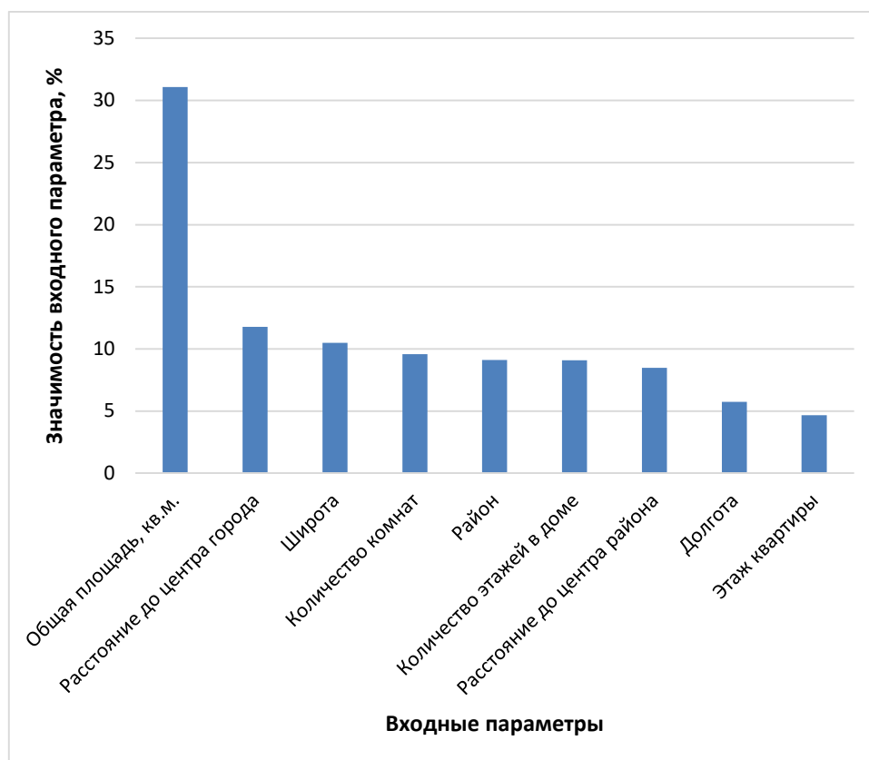
Рисунок 2. Значимость входных параметров нейросетевой модели
