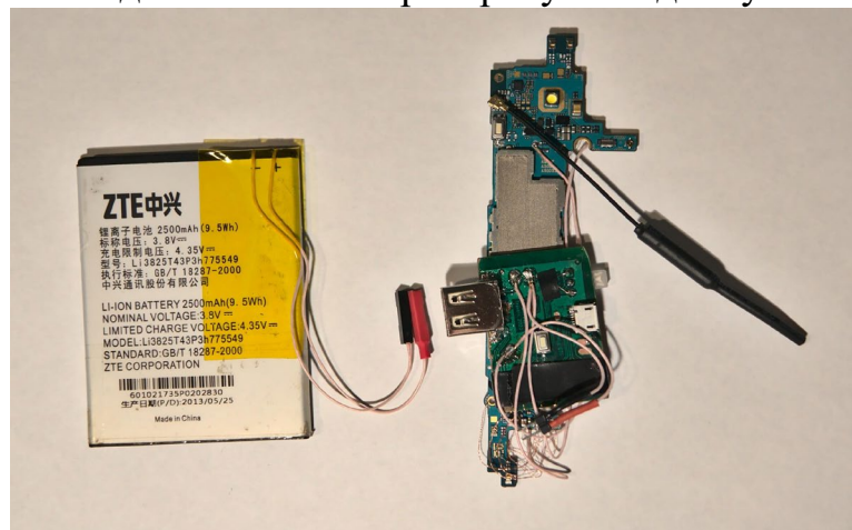
Рисунок 1. Устройство для записи данных о состоянии батареи
