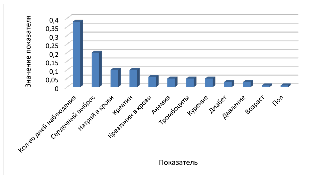
Рисунок 3. Значимость входных параметров нейросетевой модели
